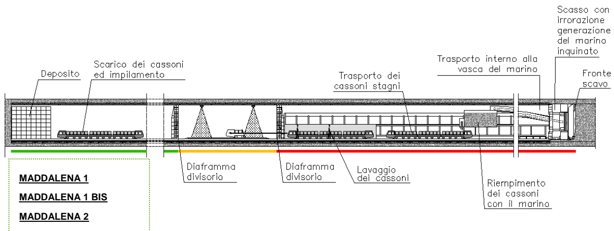
Trasporto smarino prima e dopo il suo confezionamento
