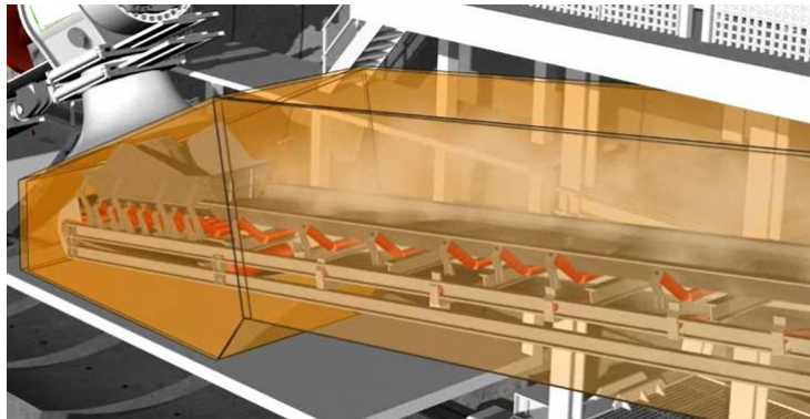
Nastro trasportatore chiuso e in depressione
