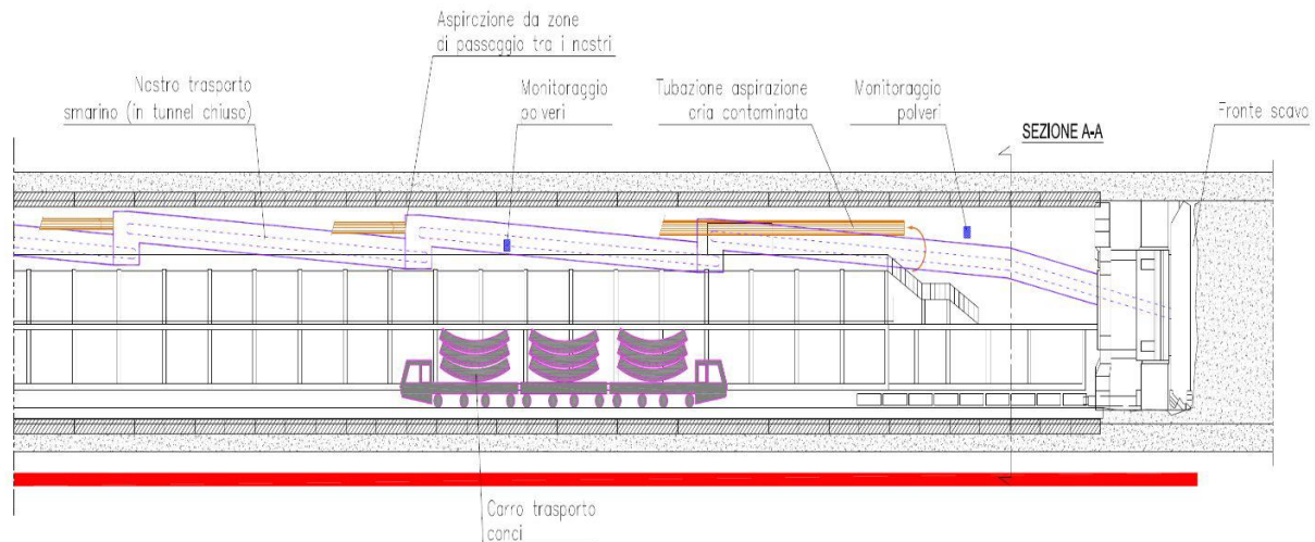
Impianto di ventilazione Particolare dei silenziatori e carter di insonorizzazione dei motori
