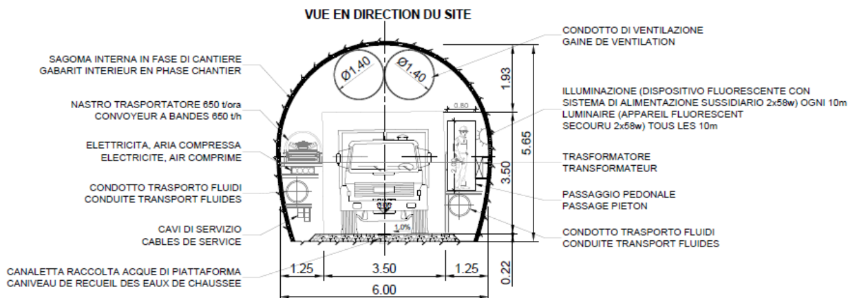
Galleria Maddalena 1 e Galleria Connessione 1: fase di cantiere
