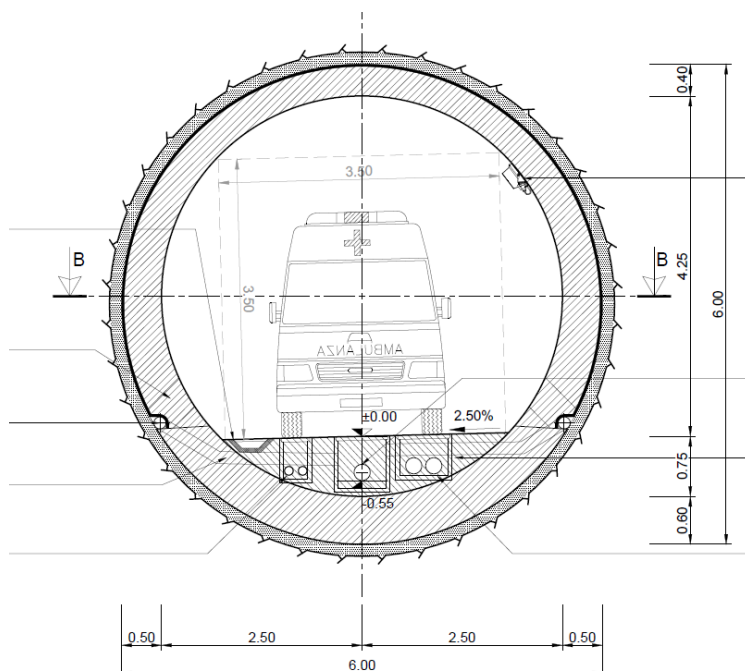
Sezione maddalena 1 in esercizio
