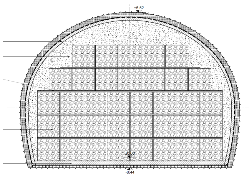
Ramo/nicchia Galleria Maddalena 2
