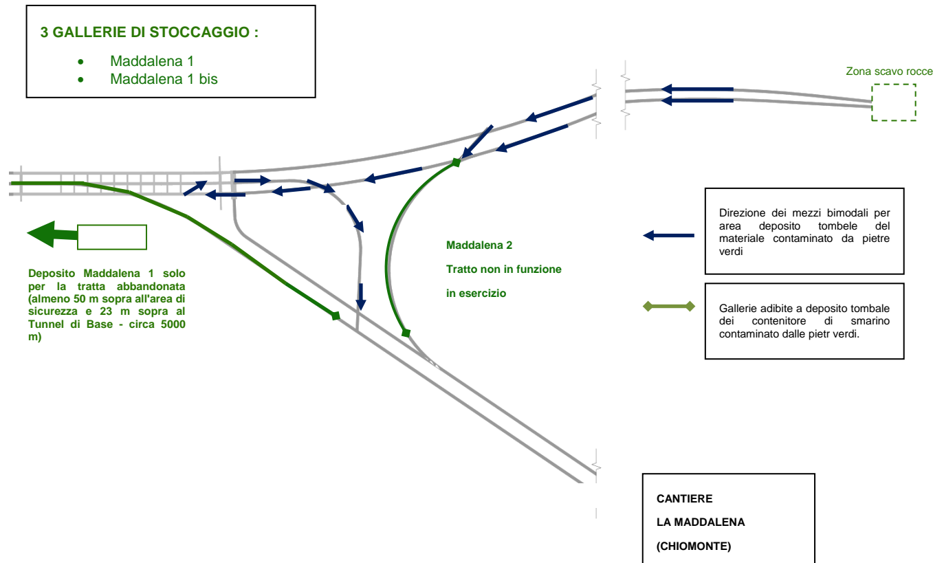
Percorso smarino verso le Gallerie di stoccaggio tombale
