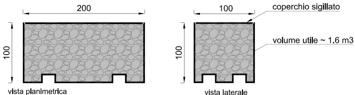
Contenitori a perdere
