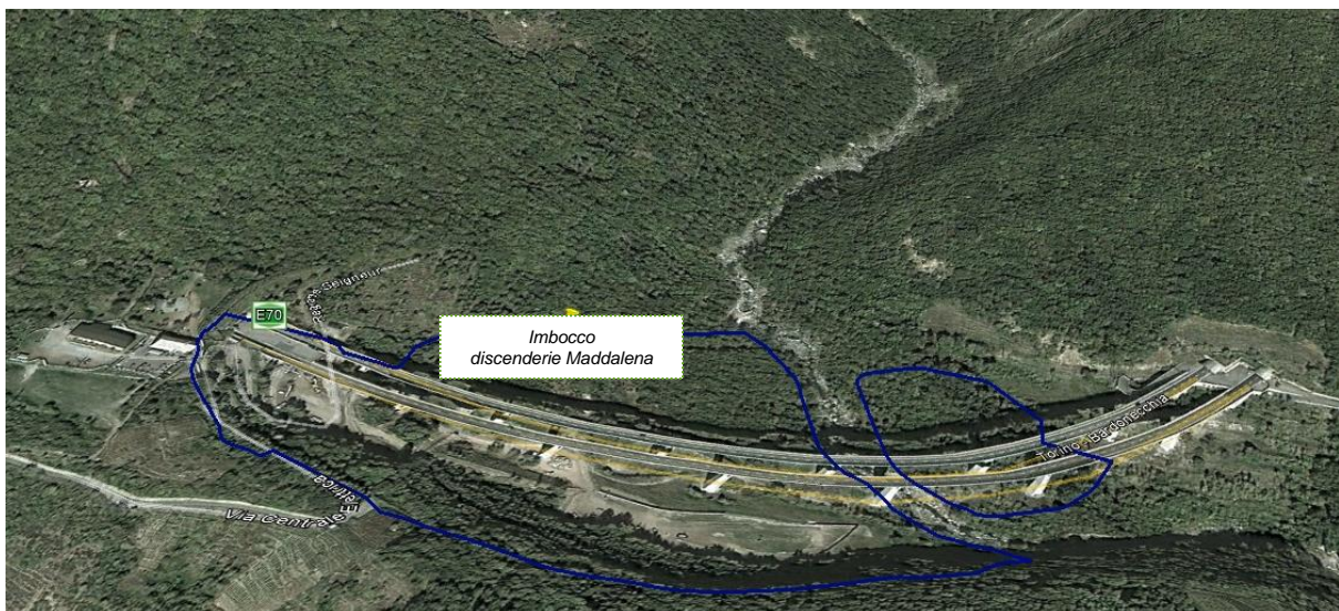
Ortofoto cantiere Maddalena
