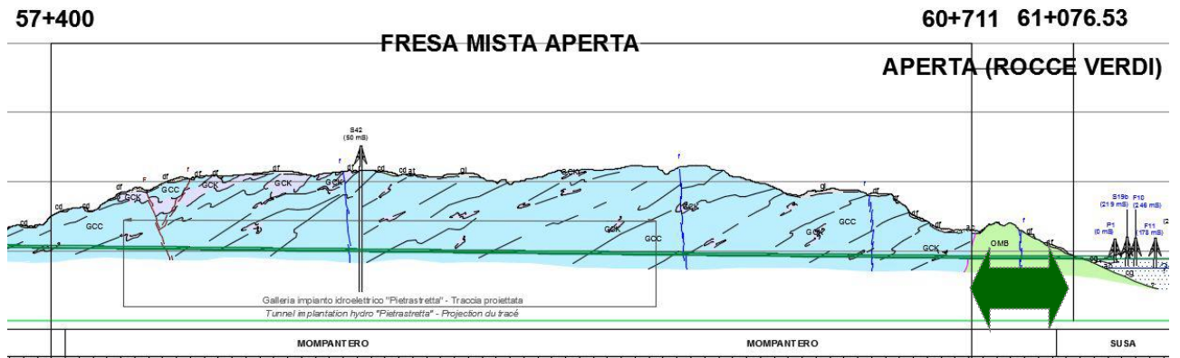
Profilo geologico della zona interessata dalle rocce verdi
