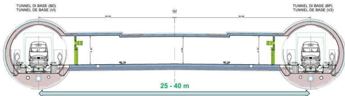
Sezione tipo Tunnel di Base in corrispondenza di un ramo di collegamento
