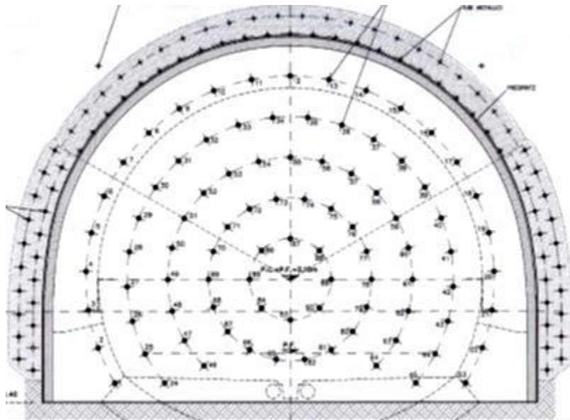
Esempio tracciamento dei fori
