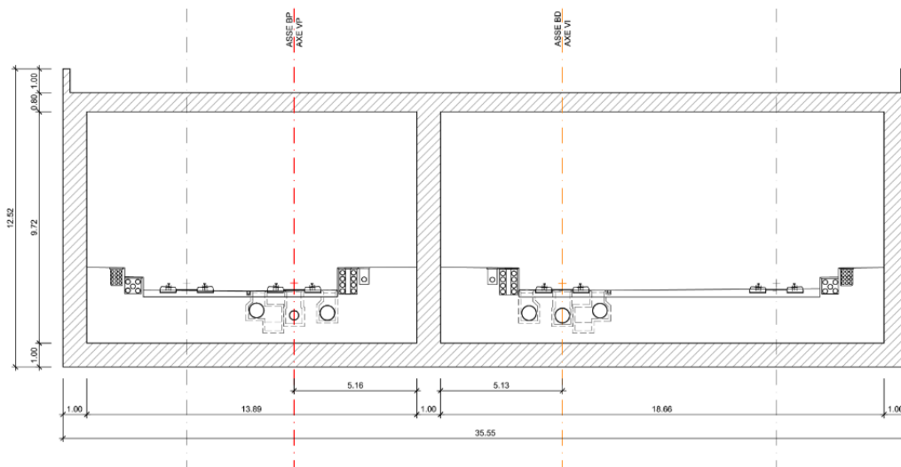
Sezione tipo galleria artificiale
