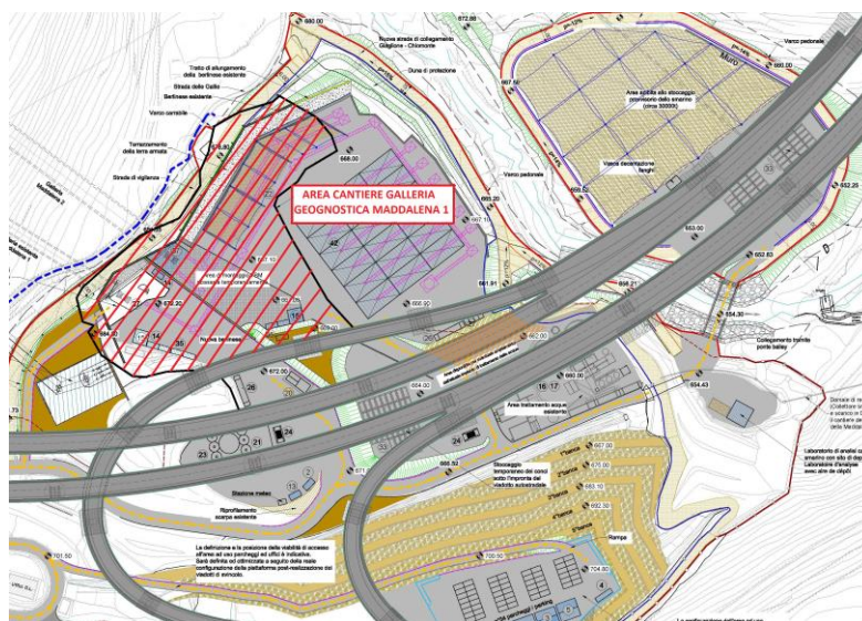
Estratto da PRV C3A 6431 – Confronto area Cantiere Maddalena 1
