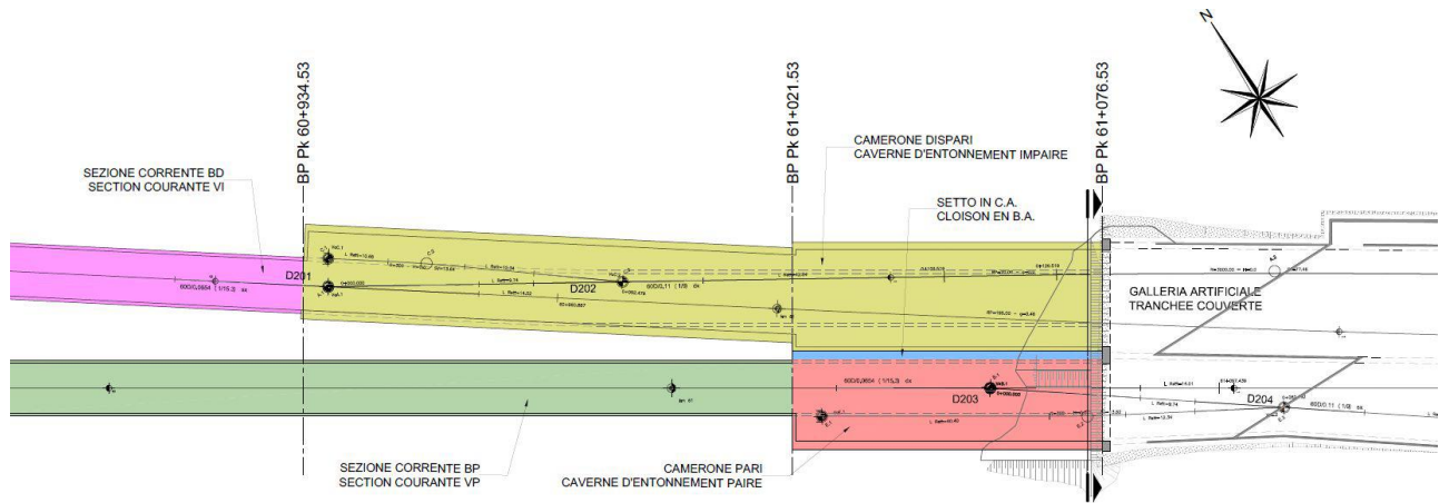
Planimetria delle sezioni allargate all'imbocco Est del Tunnel di Base (PRV_C3A_TS3_7617_33-02- 02)
