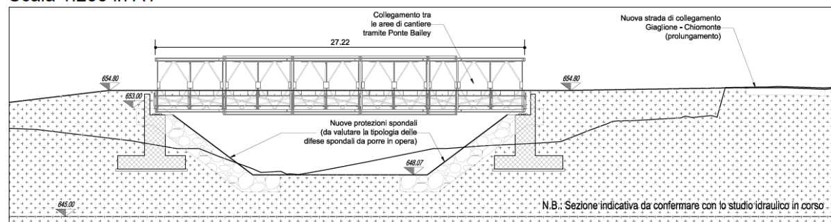
Ponte Bailey sul torrente Clarea
