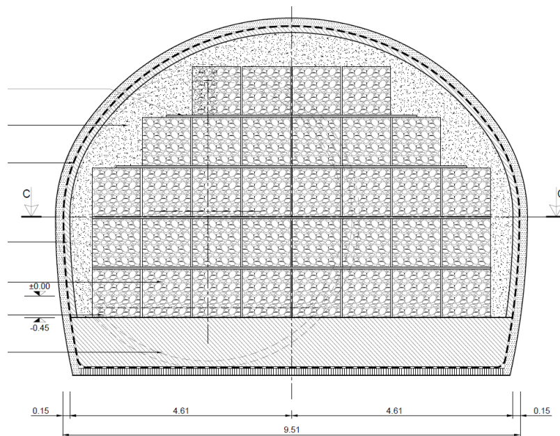
Nicchie galleria Maddalena 1
