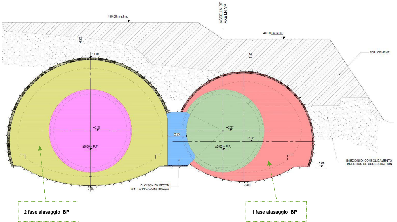
SEZIONE pk BP 61+074 COUPE pk VP 61+074
