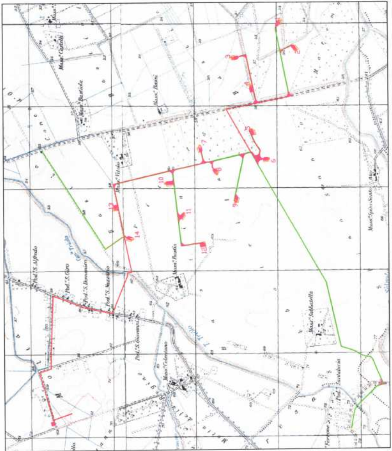
All.1 - Ubicazione impianto eolico su Tavoletta 1:25.000
