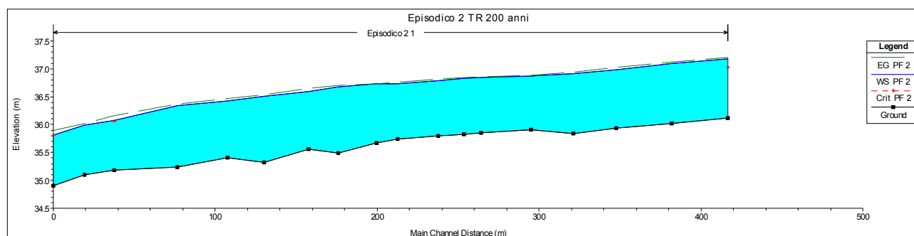
Fig. 6.2/A Profilo di corrente canale Episodico 2 per un Tr=30 anni
