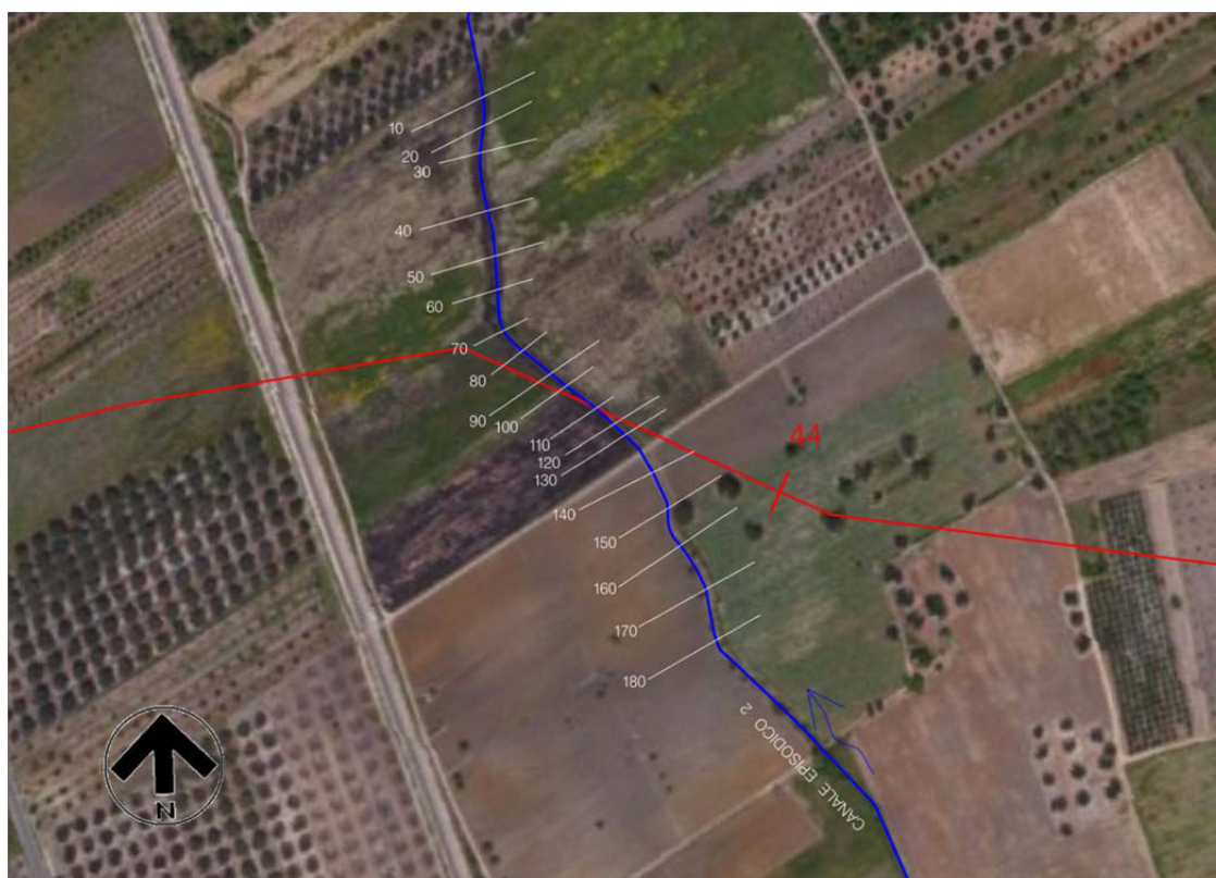
Fig.5.4/A: Tratto del canale analizzato con indicazione delle sezioni studiate
