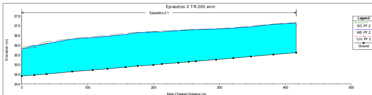
Fig.6.2/B. Profilo di corrente canale Episodico 2 per un Tr=500 anni
