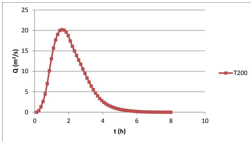
Fig.4.4/A: Idrogramma di piena del bacino del Canale Episodico 2 alla sezione di chiusura con T_r=200 anni
