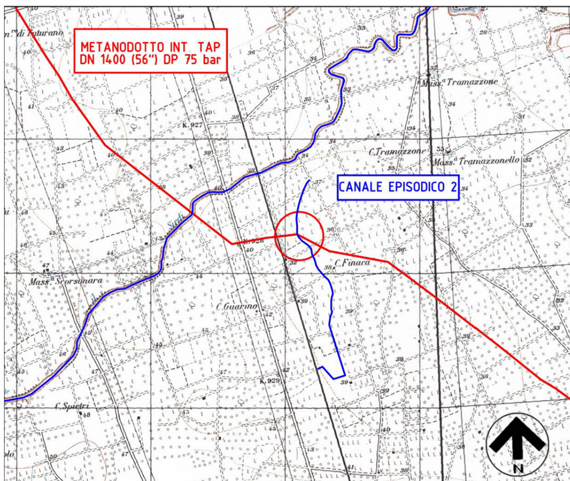
Fig. 2.1/A - Individuazione della zona di attraversamento del Canale Episodico 2 sulla Cartografia IGM 1:25.000
