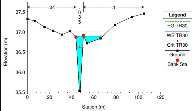
Canale Siedi_ Plan: moto permanente RS = 10
