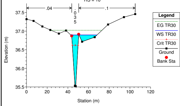
Canale Siedi_ Plan: moto permanente RS = 10
