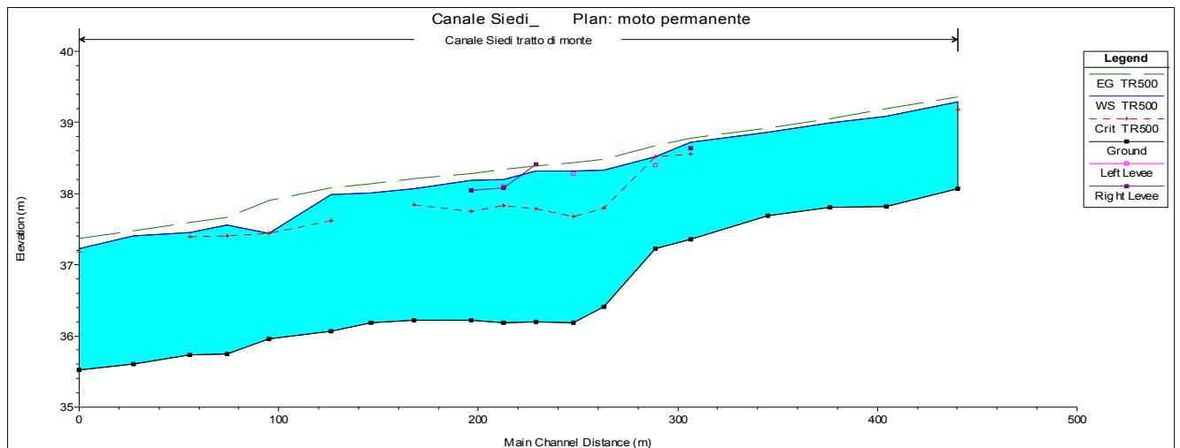
Fig. 6.2/B Profilo di corrente canale Siedi per un Tr=500 anni
