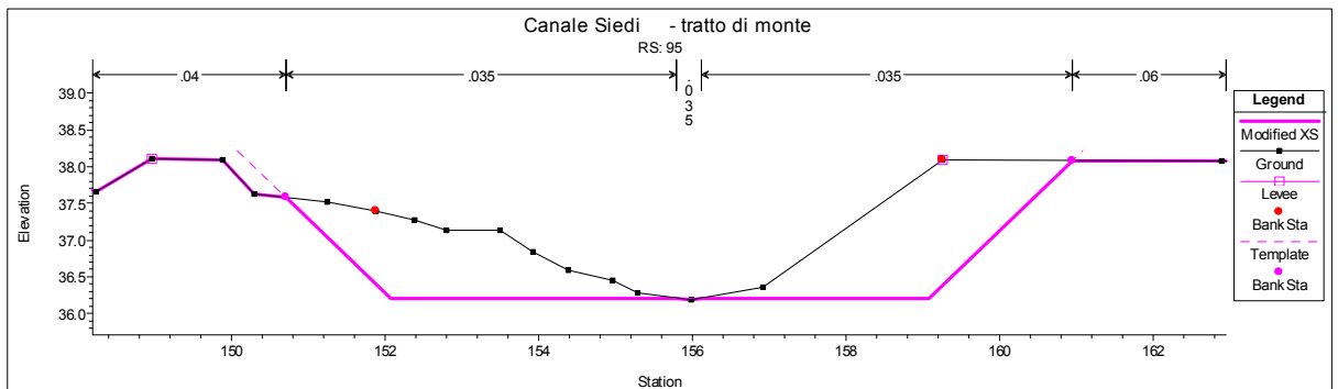
Fig. 5.3/B: Schematizzazione della sezione riprofilata
