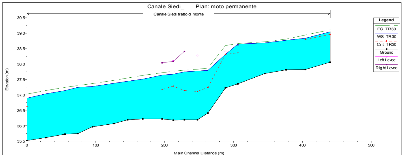
Fig. 6.2/A Profilo di corrente canale Siedi per un T_r=30 anni
