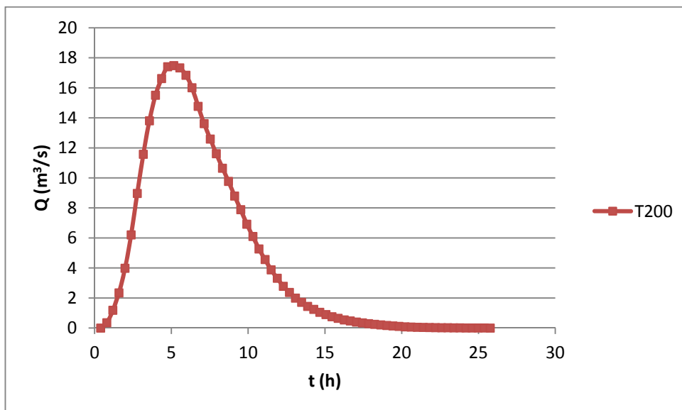
Fig.4.4/A: Idrogramma di piena del bacino del canale Siedi alla sezione di chiusura con T_r=200 anni
