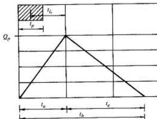
Fig.4.3/A: Idrogramma triangolare utilizzato per il calcolo della portata al colmo con metodo del Soil Conservation Service
