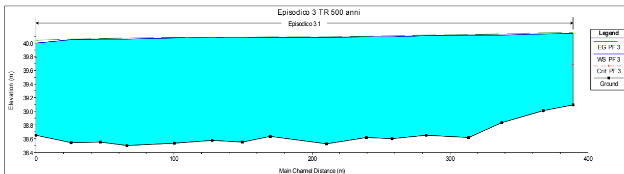
Fig.6.2/B. Profilo di corrente canale Episodico 3 per un Tr=500 anni
