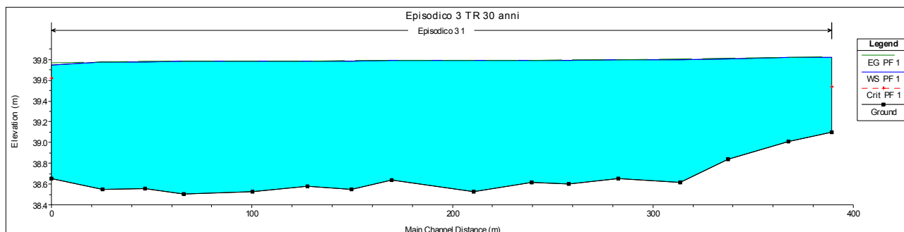
Fig. 6.2/A Profilo di corrente canale Episodico 3 per un Tr=30 anni
