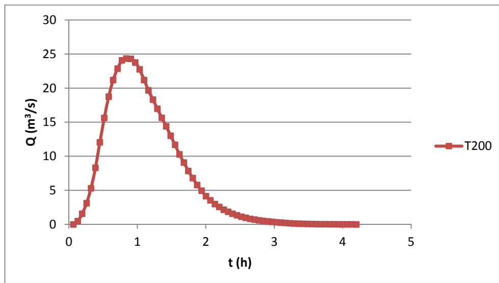
Fig.4.4/A: Idrogramma di piena del bacino del Canale Episodico 3 alla sezione di chiusura con T_r=200 anni
