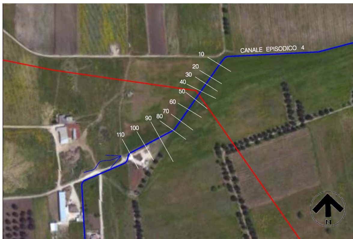
Fig.5.4/A: Tratto del canale analizzato con indicazione delle sezioni studiate
