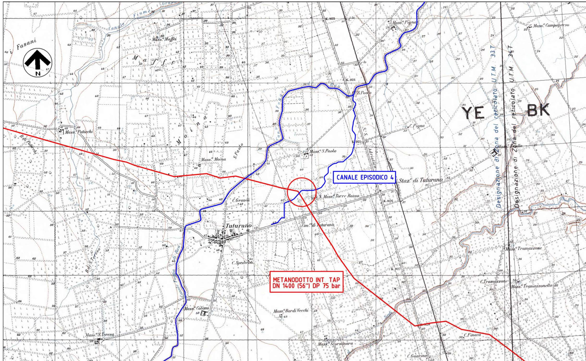
Fig. 2.1/A - Individuazione della zona di attraversamento del Canale Episodico 4 sulla Cartografia IGM 1:25.000
