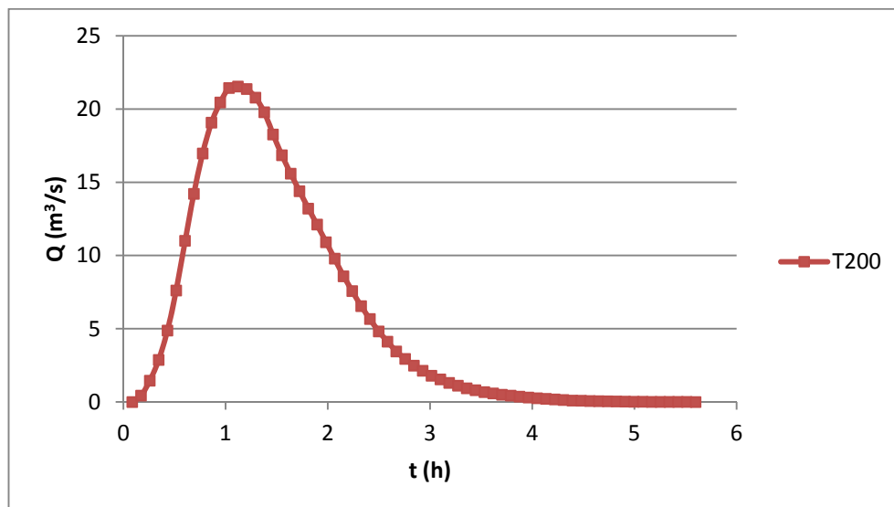
Fig.4.4/A: Idrogramma di piena del bacino del Canale Episodico 4 alla sezione di chiusura con T_r=200 anni
