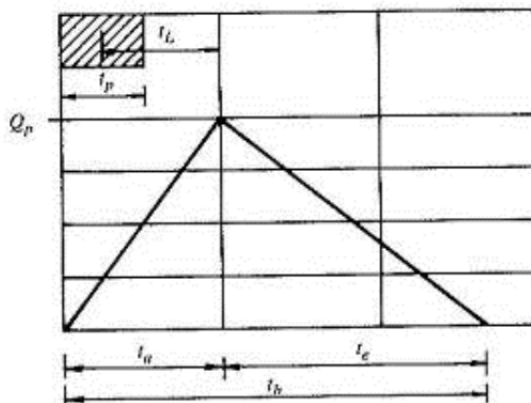
Fig.4.3/A: Idrogramma triangolare utilizzato per il calcolo della portata al colmo con metodo del Soil Conservation Service
