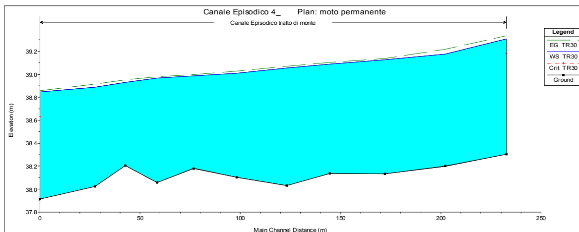
Fig. 6.2/A Profilo di corrente canale Episodico 4 per un Tr=30 anni
