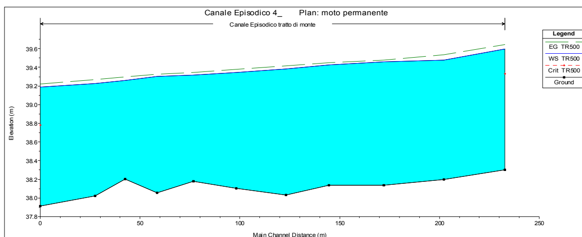
Fig.6.2/B. Profilo di corrente canale Episodico 4 per un Tr=500 anni
