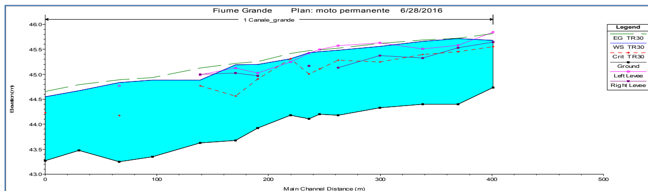
Fig. 6.2/A Profilo di corrente fiume Grande per un Tr=30 anni
