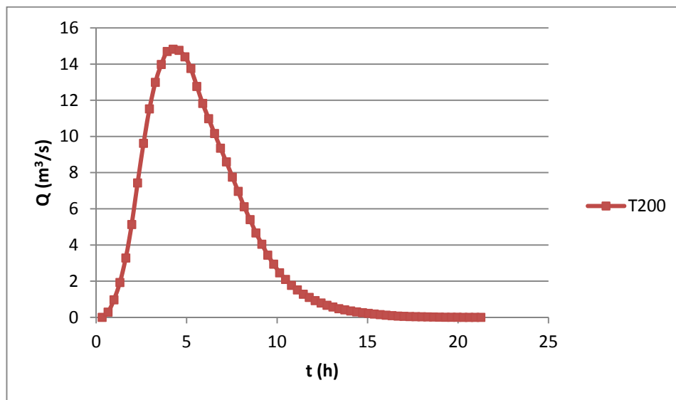
Fig.4.4/A: Idrogramma di piena del bacino del Fiume Grande alla sezione di chiusura con T_r=200 anni
