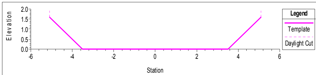
Fig. 5.3/B: Schematizzazione della sezione riprofilata
