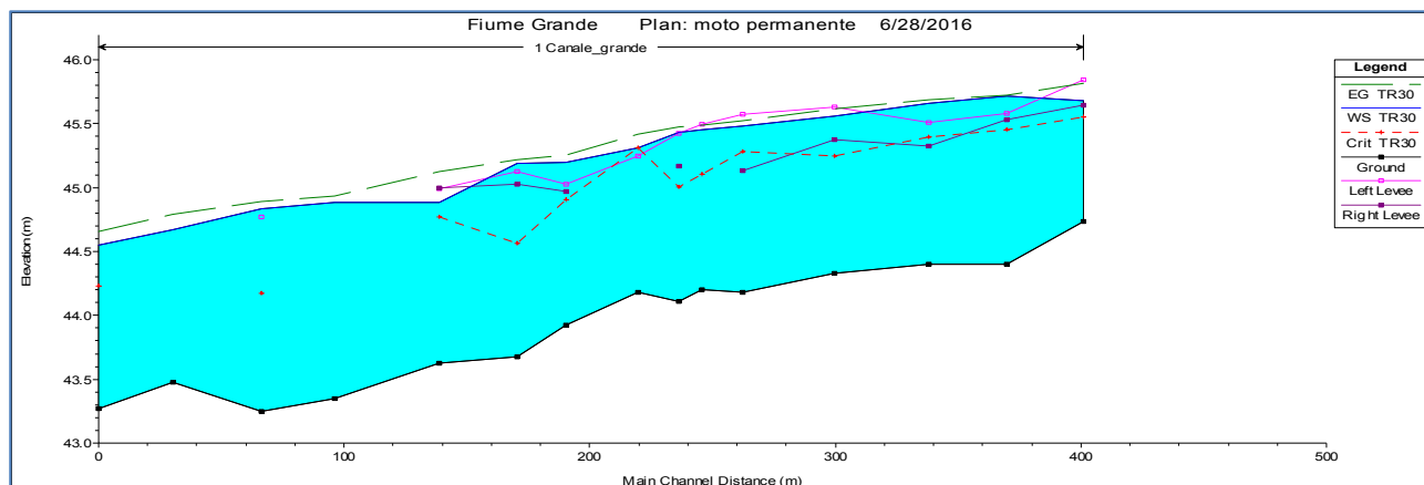
Fig. 6.2/B Profilo di corrente fiume Grande per un T_r=500 anni
