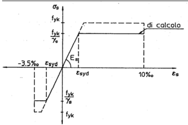
Legame costitutivo acciaio
