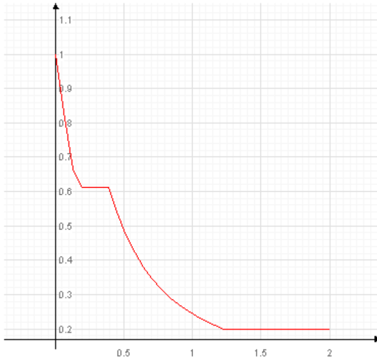
Spettro di risposta per lo stato limite ultimo cond. Dinamica 2
