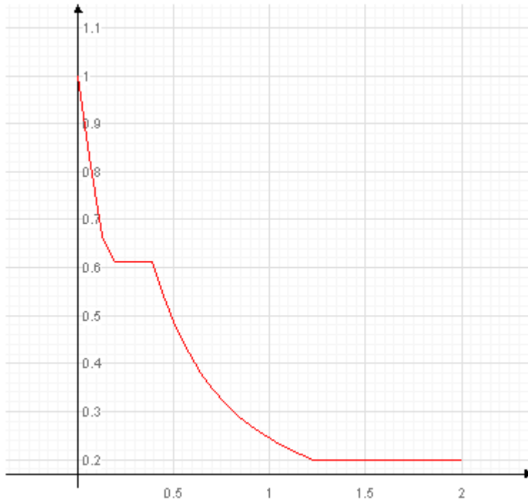
Spettro di risposta per lo stato limite ultimo cond. Dinamica 1
