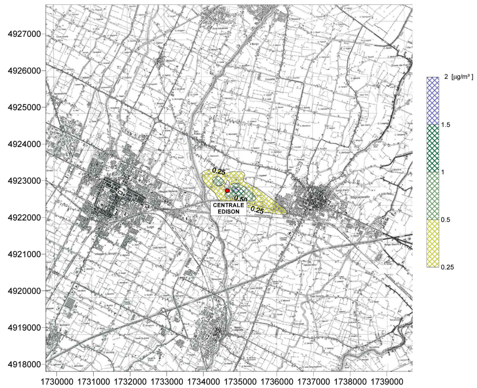
Mappe delle Concentrazioni Medie Annue di NOx
