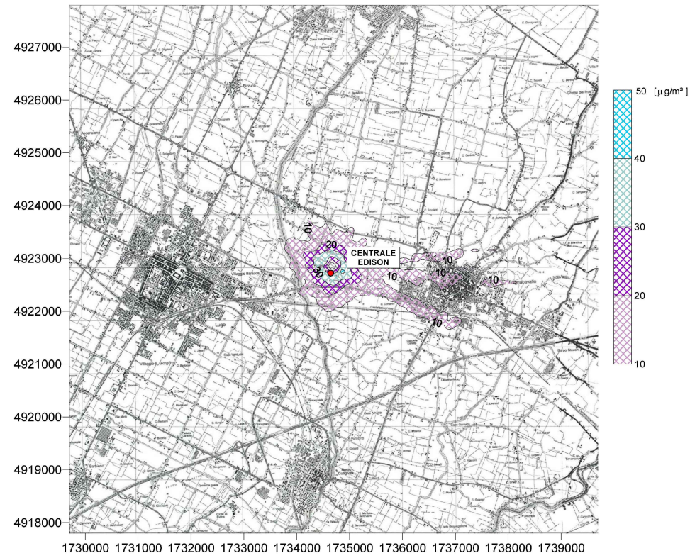
Mappe delle Concentrazioni Massime Orarie di NOx - 99.8° Percentile
