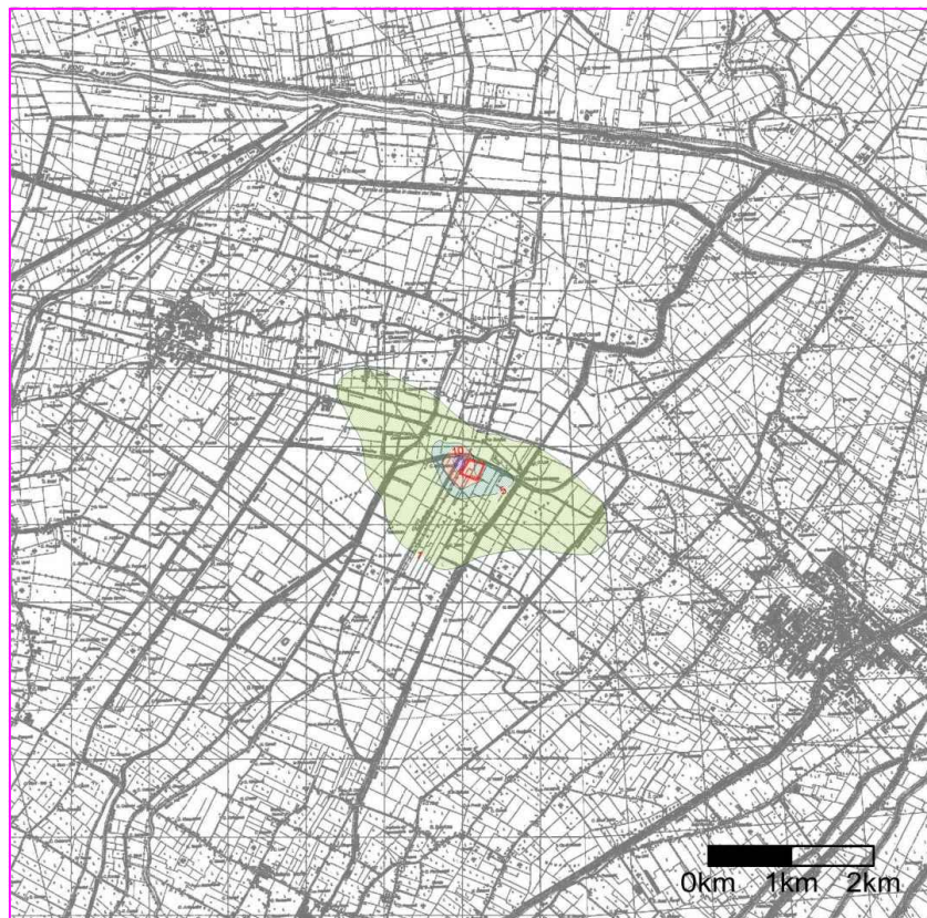
Cluster C, Mappa delle Concentrazioni Medie Annue di Nox
