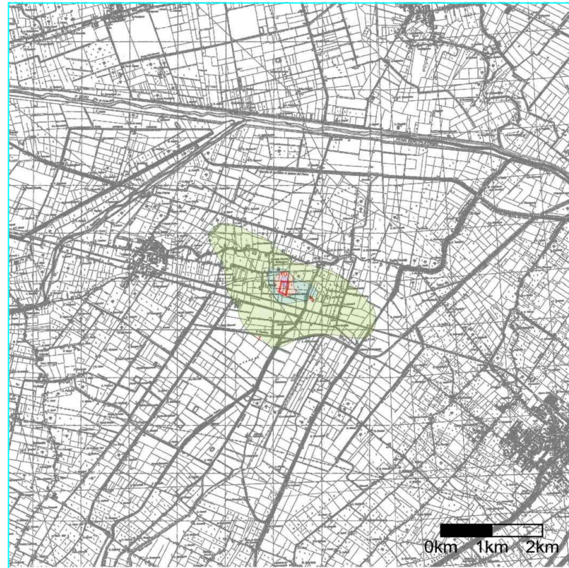
Cluster B-D, Mappa delle Concentrazioni Medie Annue di Nox
