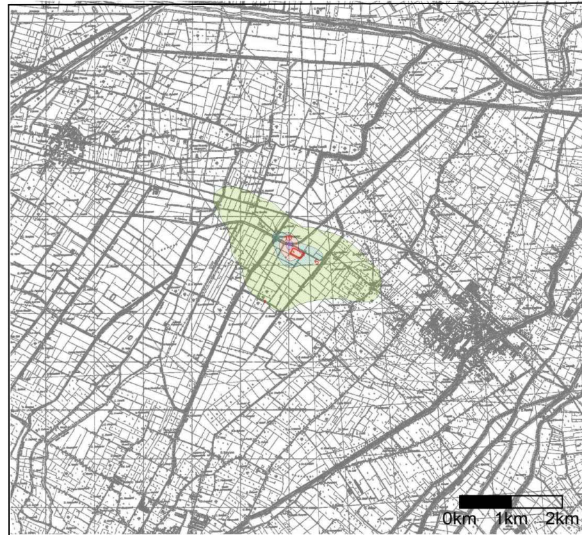
Cluster A, Mappa delle Concentrazioni Medie Annue di Nox
