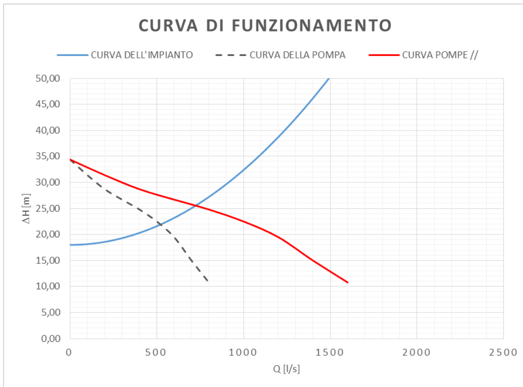
Figura 5.2: Curve Caratteristiche dell'Impianto e delle Due Pompe in Parallelo
