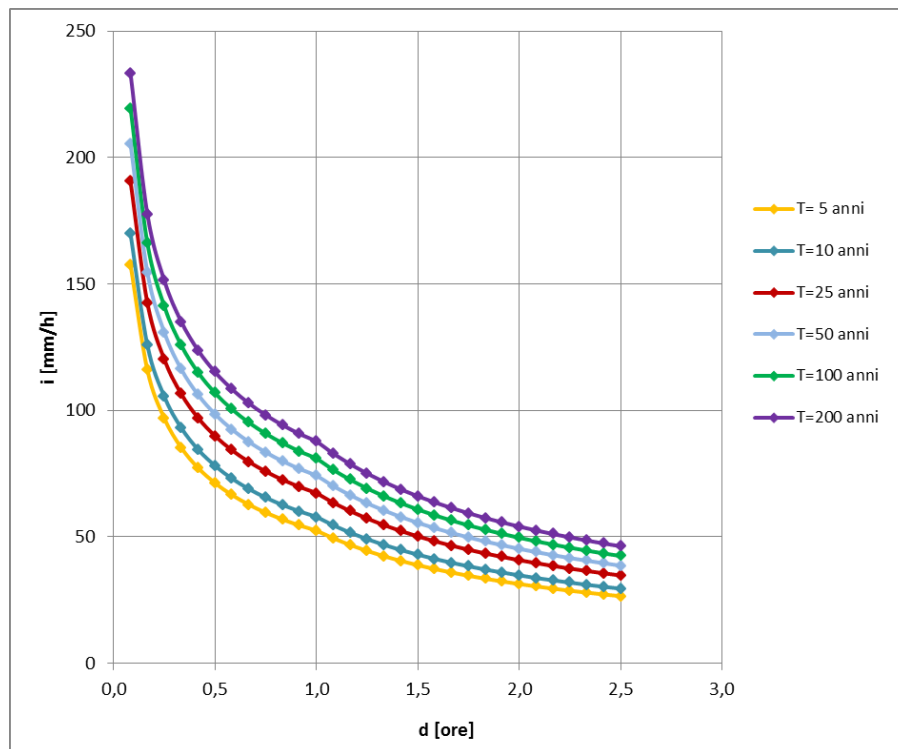
Figura 2.2: Curve Intensità-Durata-Frequenza (IDF)
