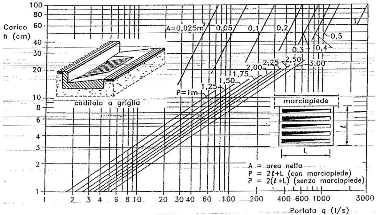
Figura 4.3: Scala delle Portate di una Griglia
