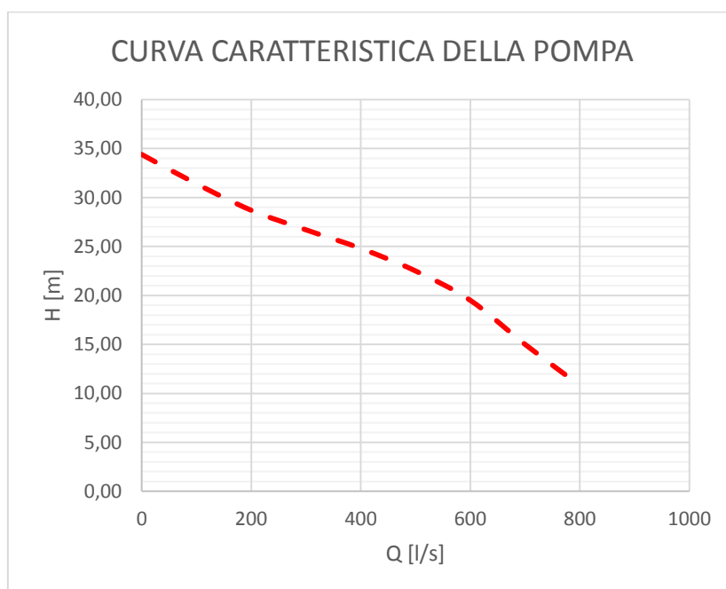
Figura 5.1: Curva Caratteristica della Pompa
