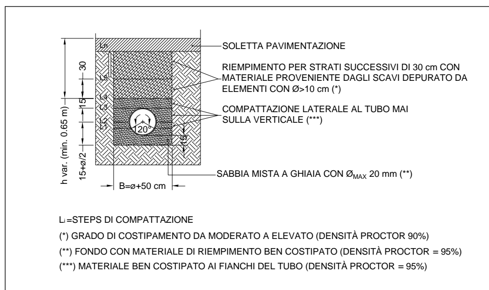
Figura 4.2: Dettaglio Posa Tubazioni PEAD
