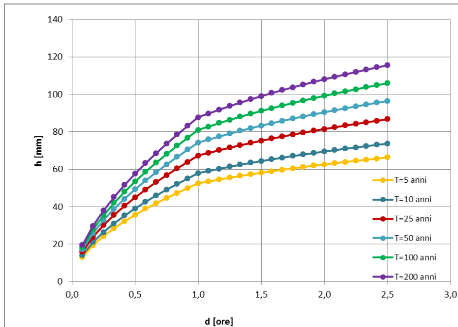
Figura 2.1: Curve di Probabilità Pluviometrica
