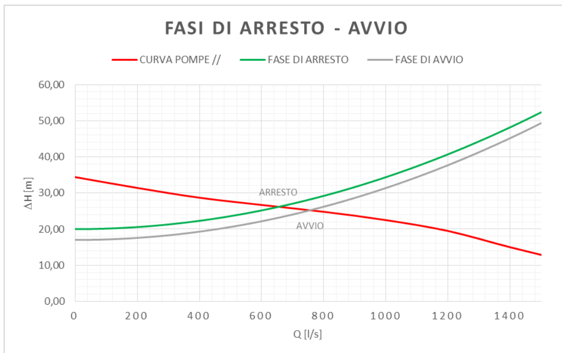
Figura 5.3: Intervallo di Funzionamento delle Pompe tra il Punto di Arresto e Quello di Avvio
