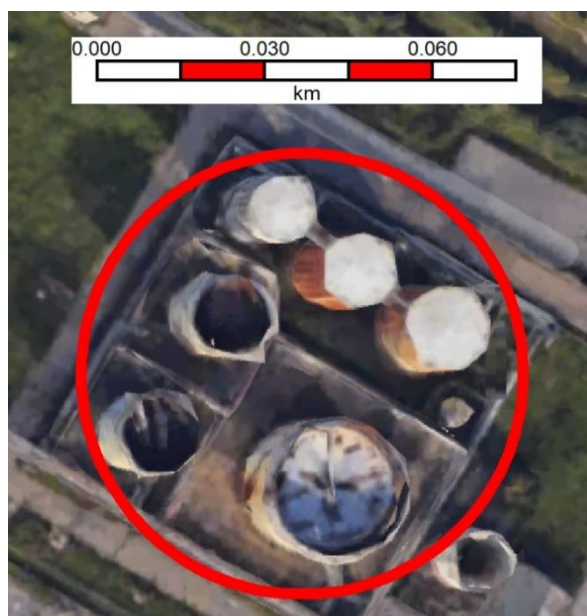
Figura 28 Valutazione di possibili effetti domino di secondo livello indotti dalla rottura dei serbatoi in Z4; rappresentazione dell'inviluppo dello scenario peggiore ( pool fire in 5D ) considerando tutte le possibili direzioni del vento.
