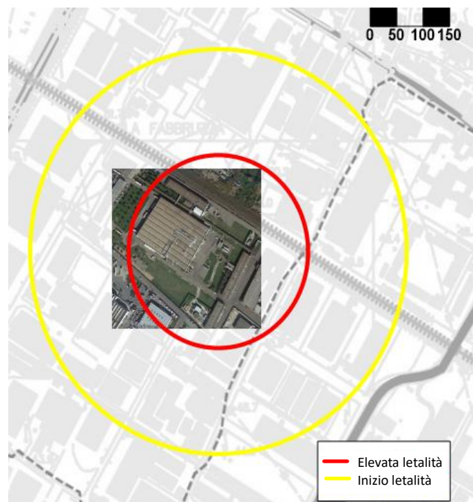
Figura 31 Valutazione dell'impatto sul territorio del flash fire associato alla rottura dei serbatoi di GPL; rappresentazione dell'involuppo dello scenario considerando tutte le possibili direzioni del vento.
