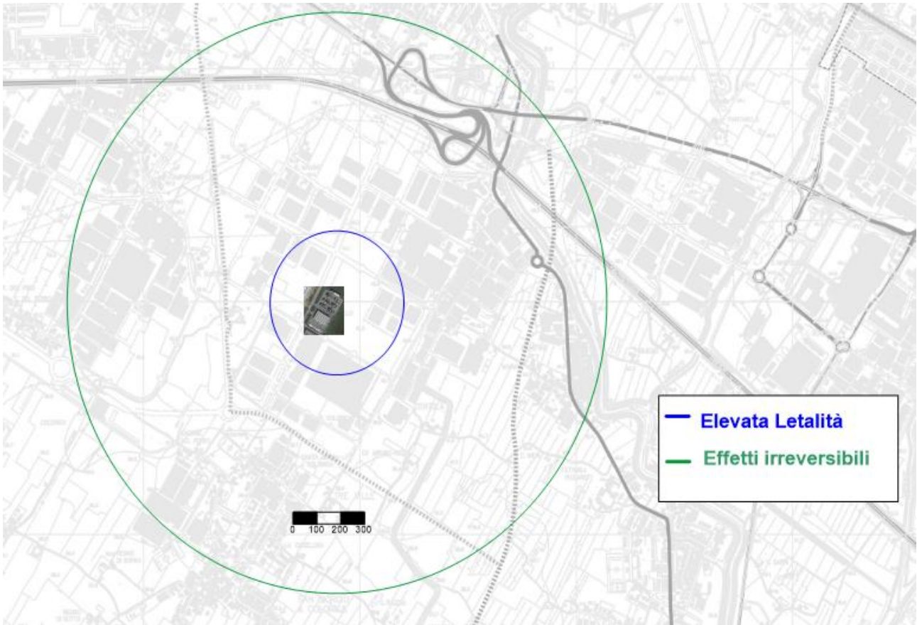
Figura 20 Valutazione dell'impatto sul territorio delle dispersioni tossiche di percloroetilene; rappresentazione dell'involuppo della massima estensione della nube considerando tutte le possibili direzioni del vento.
