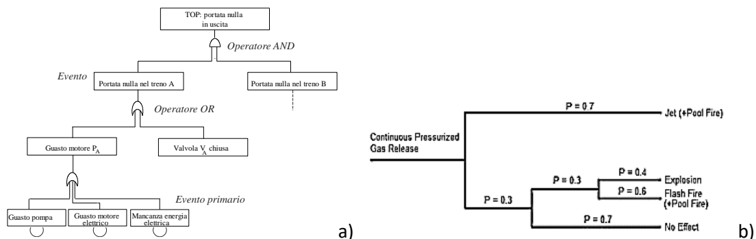
Figura 2 a) Esempio di un albero dei guasti; b) Esempio di un albero degli eventi
