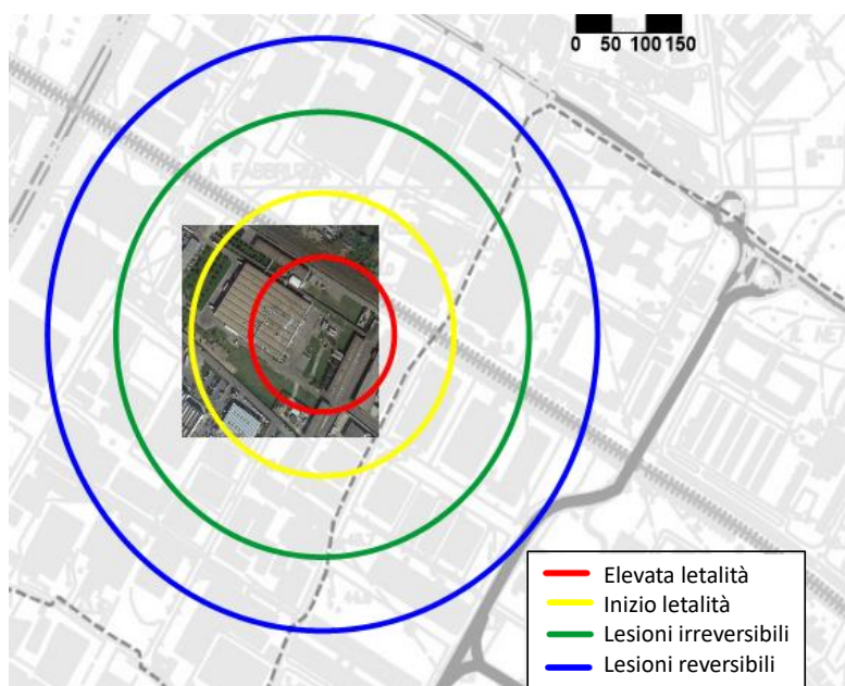
Figura 32 Valutazione dell'impatto sul territorio del fireball associato alla rottura dei serbatoi di GPL; rappresentazione dell'area di impatto effettiva, che risulta indipendente dalla direzione del vento.
