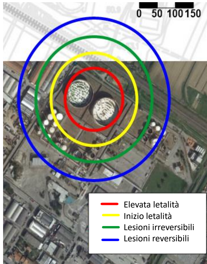
Figura 24 Valutazione dell'impatto sul territorio del pool fire associato alla rottura dei serbatoi nella zona Z2; rappresentazione dell'inviluppo dello scenario considerando tutte le possibili direzioni del vento.
