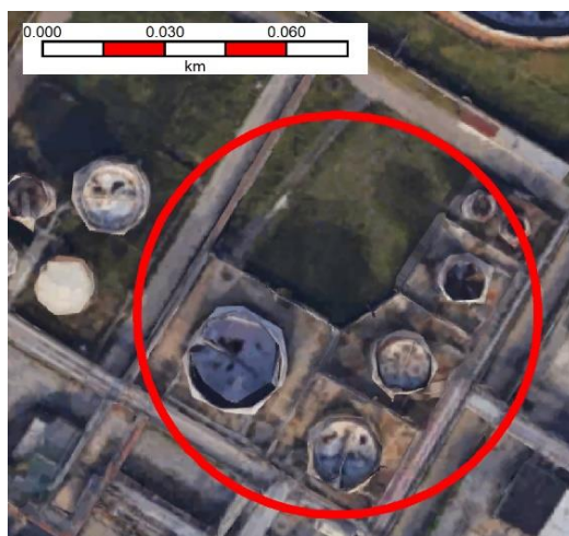
Figura 26 Valutazione di possibili effetti domino di secondo livello indotti dalla rottura dei serbatoi in Z3; rappresentazione dell'involuppo dello scenario peggiore (pool fire in 5D) considerando tutte le possibili direzioni del vento.
