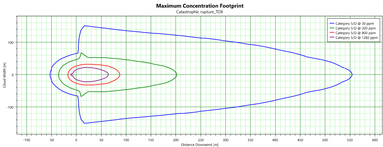
Figura 16 Profili di concentrazione ottenuti per le dispersioni di acido formico: A) condizioni 2F; b) condizioni 5D.
