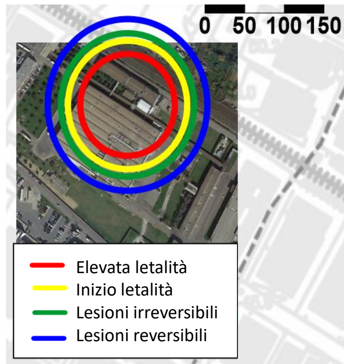
Figura 30 Valutazione dell'impatto sul territorio del pool fire associato alla perdita di etanolo; rappresentazione dell'involuppo dello scenario considerando tutte le possibili direzioni del vento.
