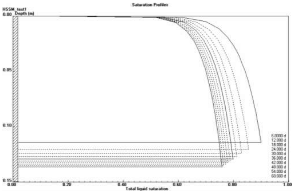
Figura 399 - Scenario I, saturazione in acqua della zona vadosa 2 %. Profilo di saturazione relativo ai primi 60 giorni dal rilascio
