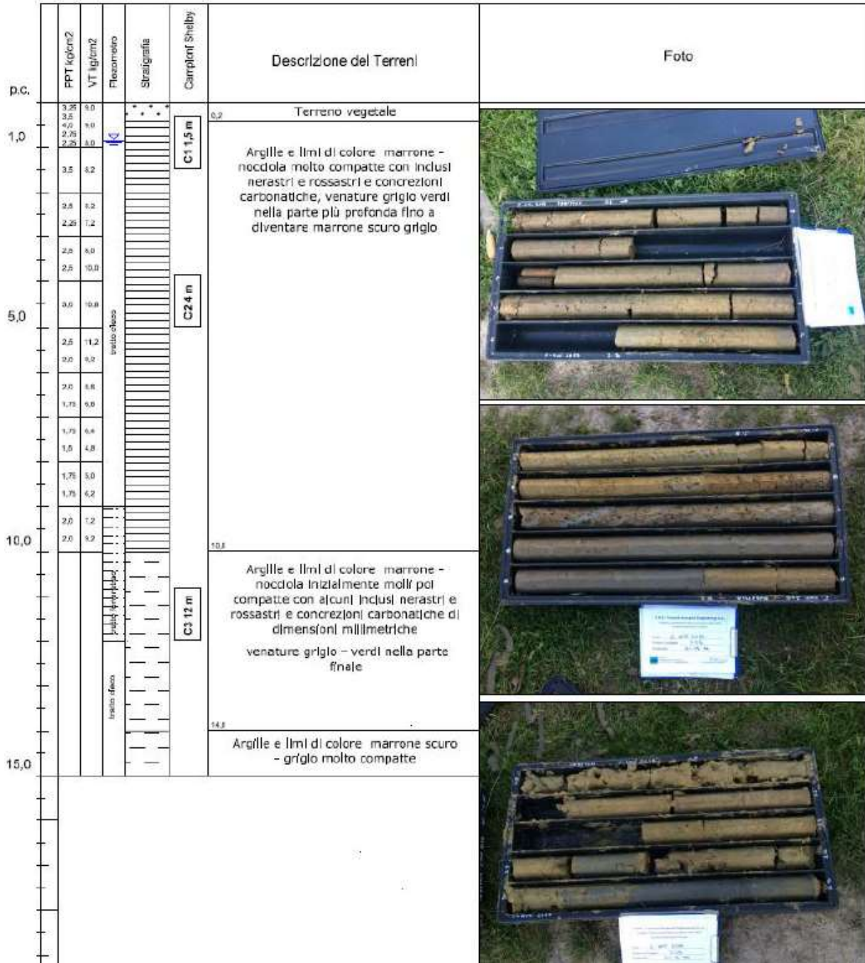
Figura 26 - Stratigrafia del sondaggio S05 realizzato durante la campagna geognostica presso l'area di progetto (in arancione in Figura 22)
