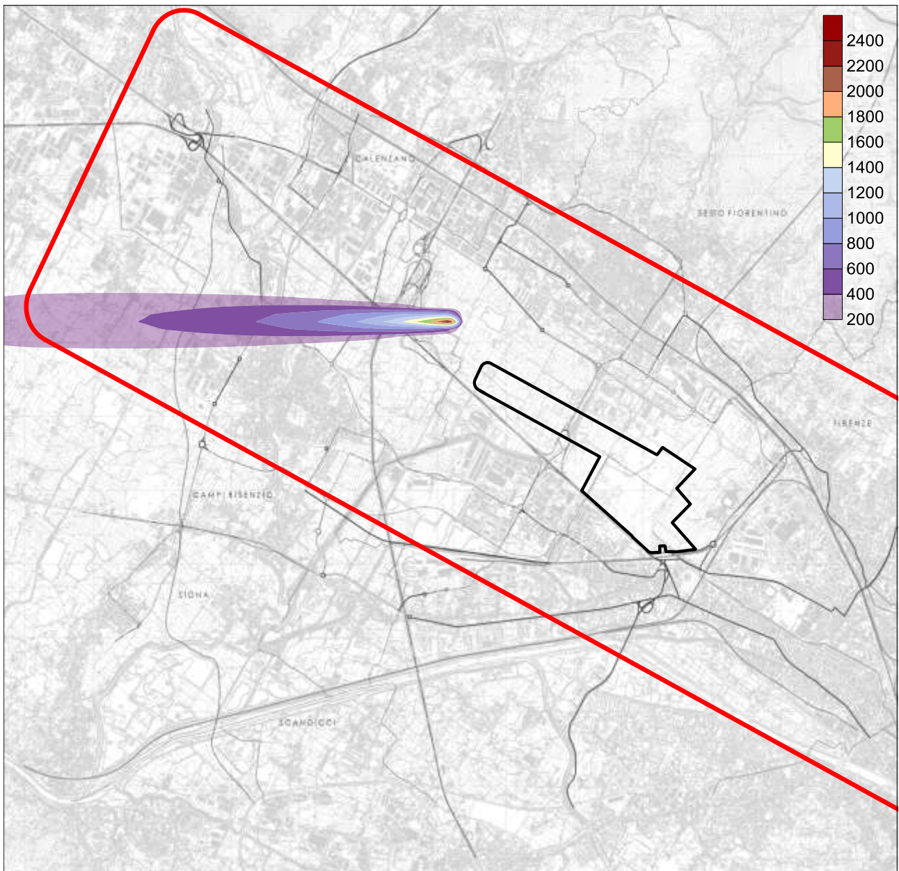
Figura 8 Valori di concentrazione, espressi in \mu\text{g}/\text{m}^3 , massimi orari calcolati sull'arco di 24 ore per emissioni di CO = Monossido di Carbonio da combustione derivata dall'incendio per il crash dell'aeromobile - scenario 3 - condizioni meteo 5D.
