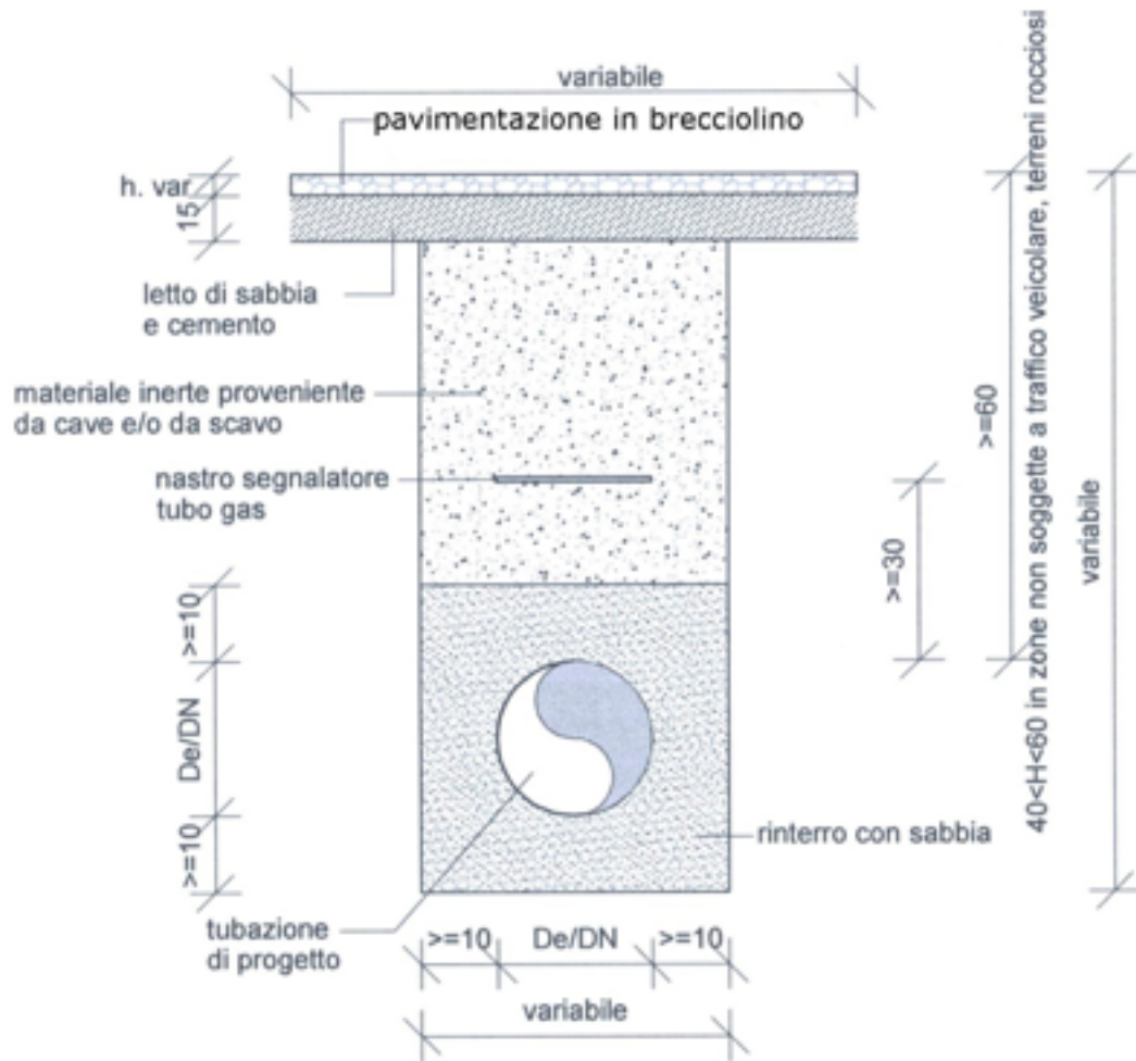
Particolare costruttivo per sezione di scavo su strada sterrata
