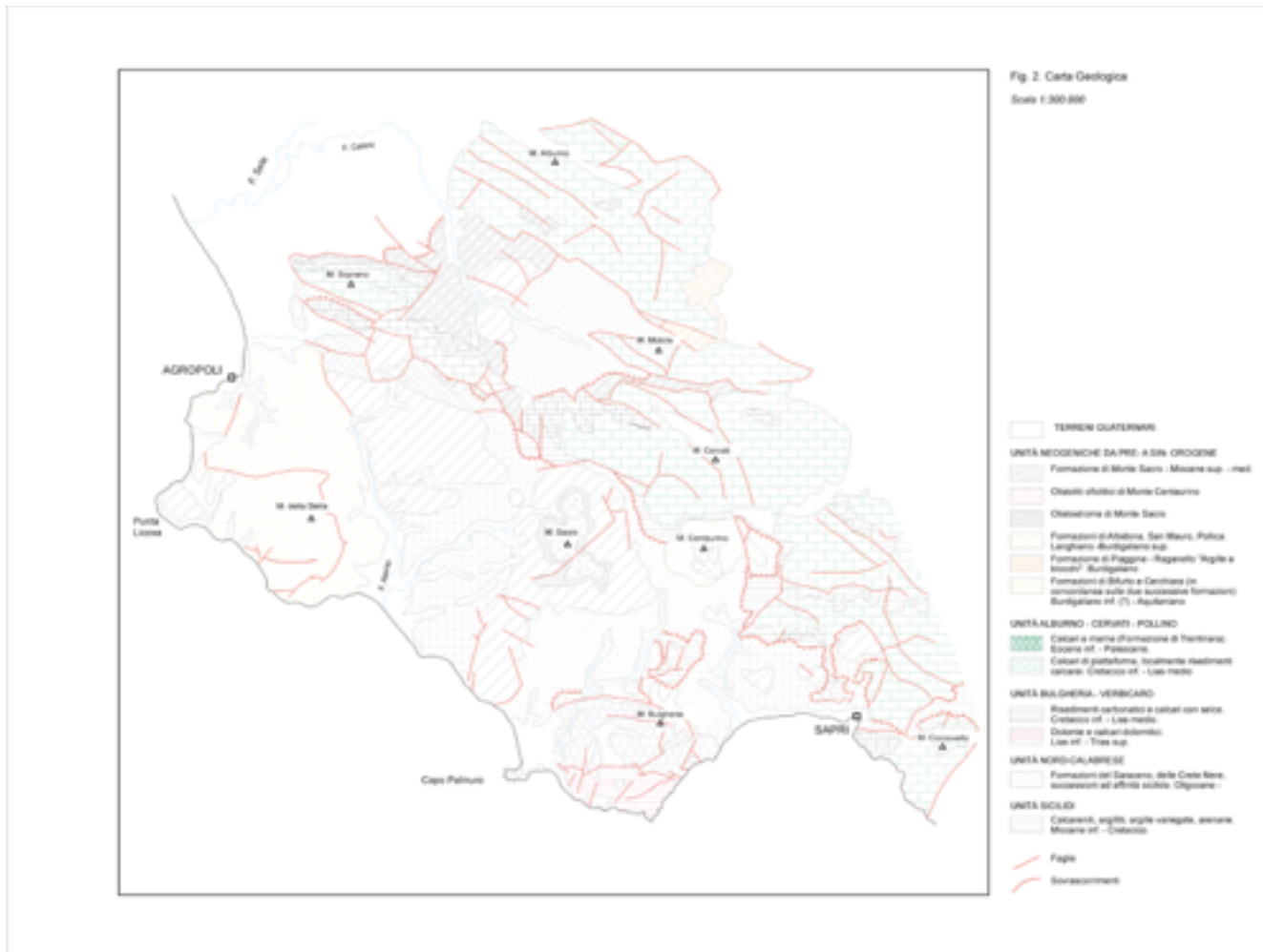
Carta geologica
