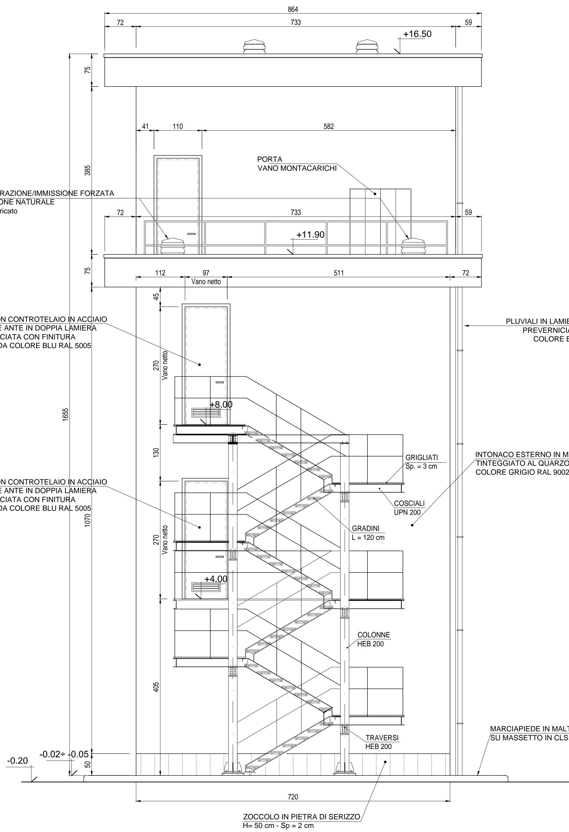
PROSPETTO 3 Scala: 1:50
