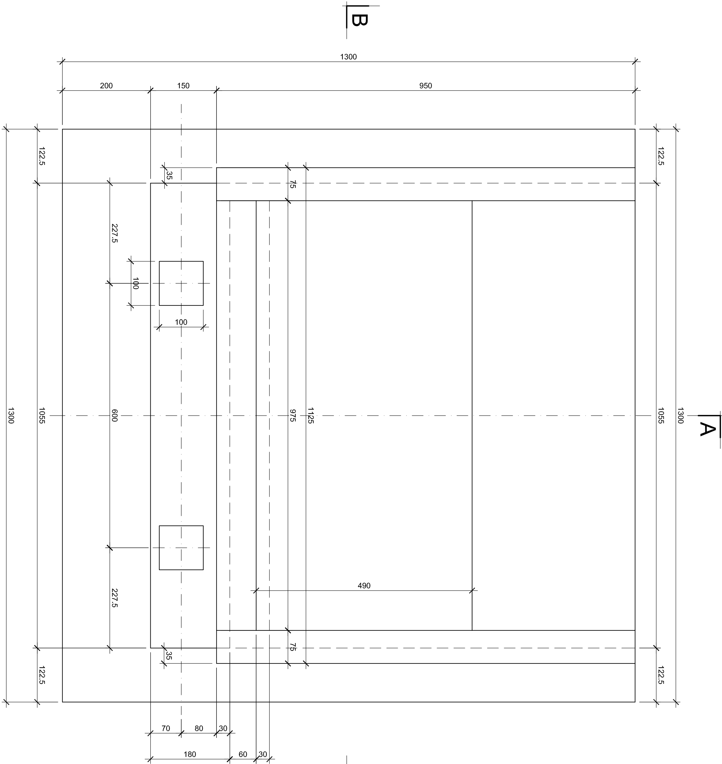
PIANTA 1:50
