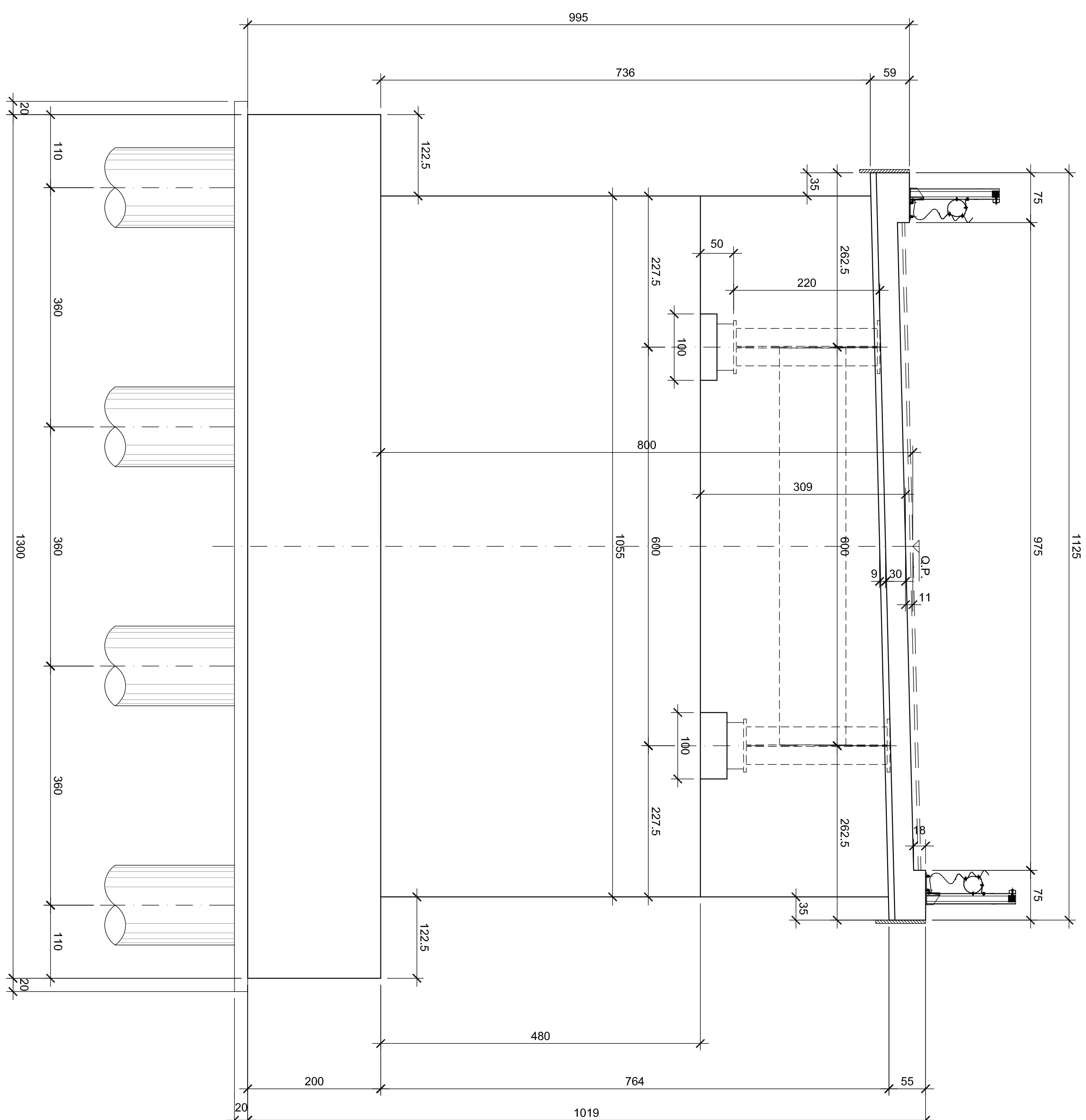
PROSPETTO FRONTALE 1:50
