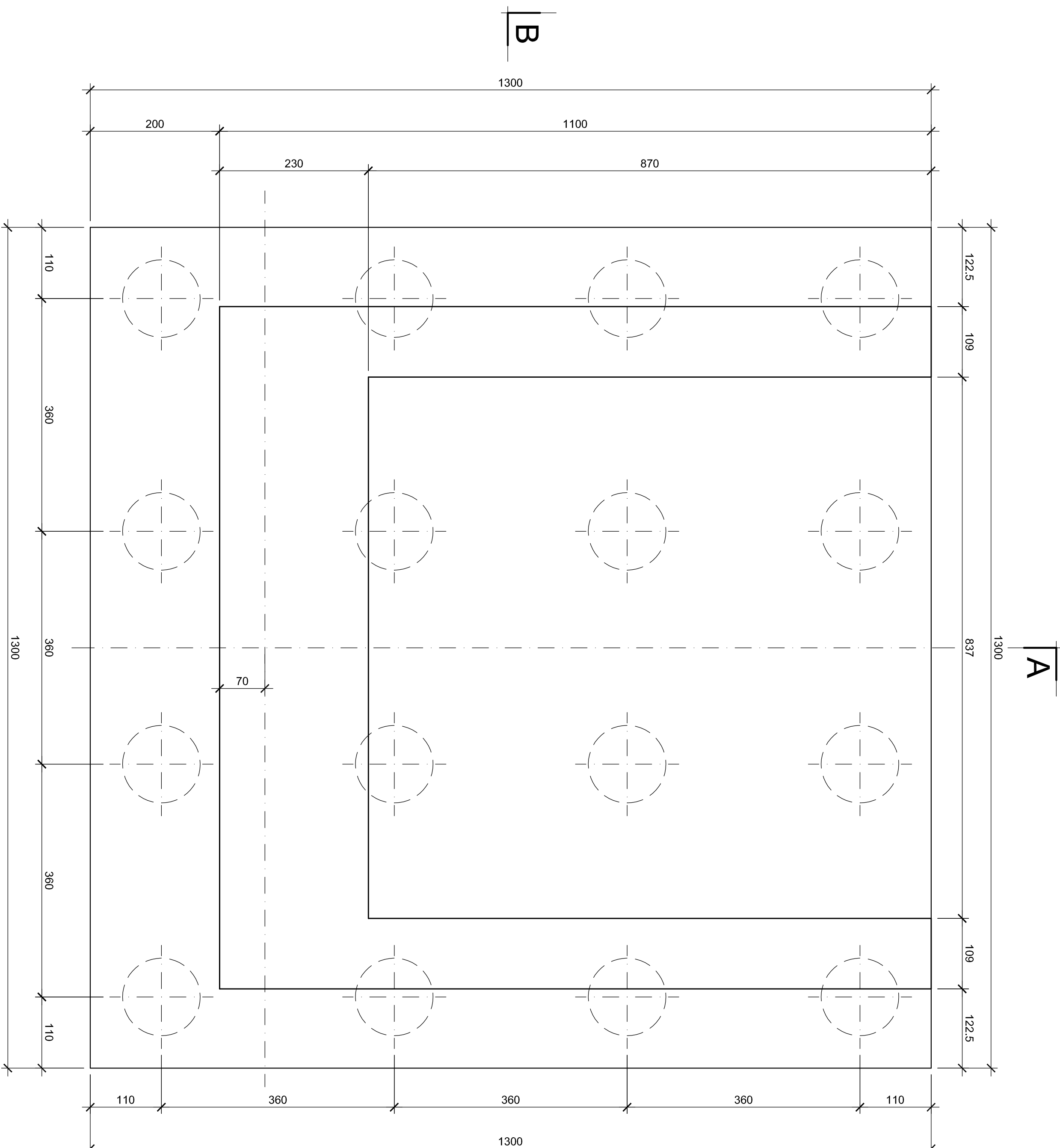
PIANTA FONDAZIONE 1:50
