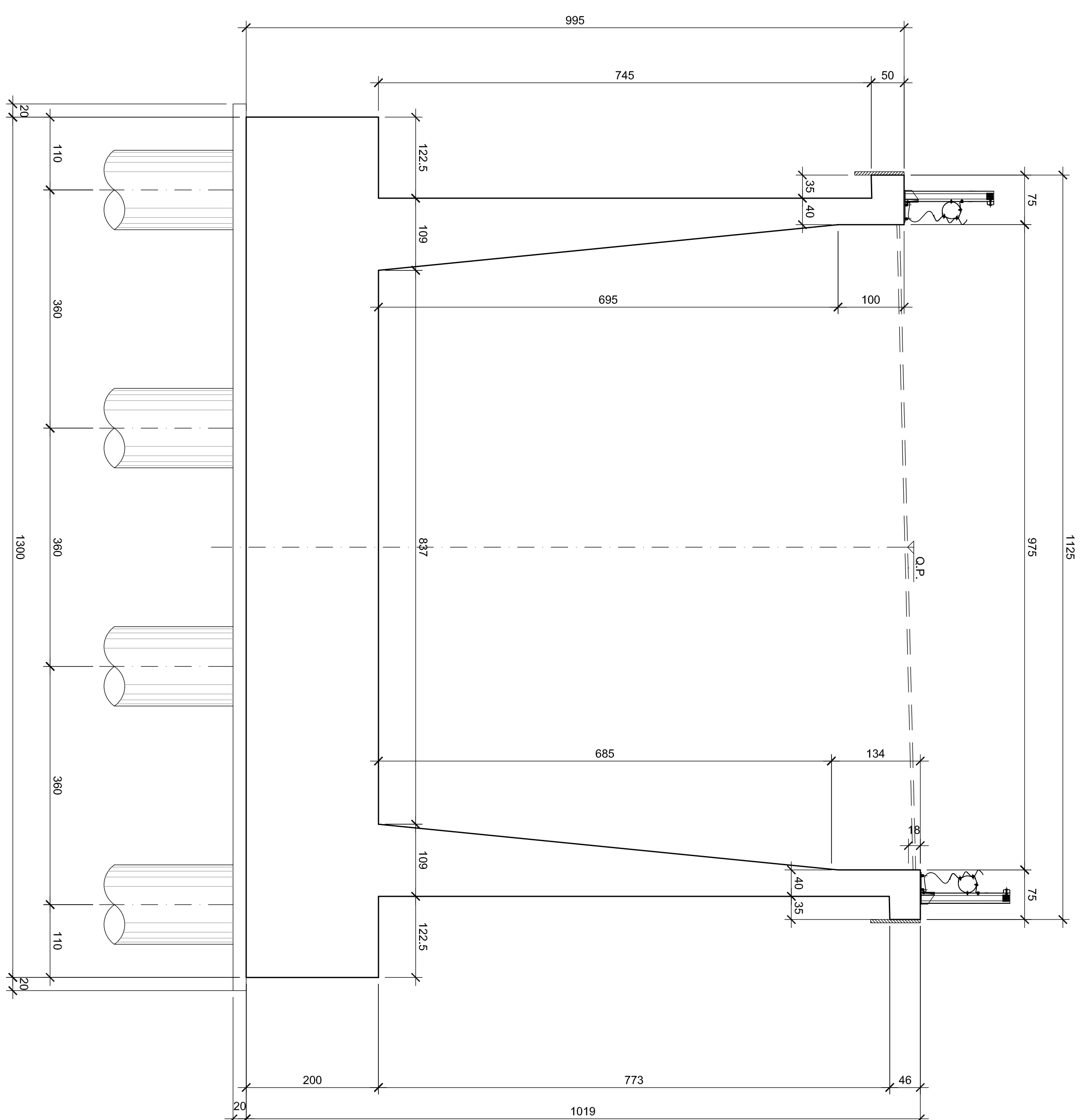
SEZIONE B-B 1:50
