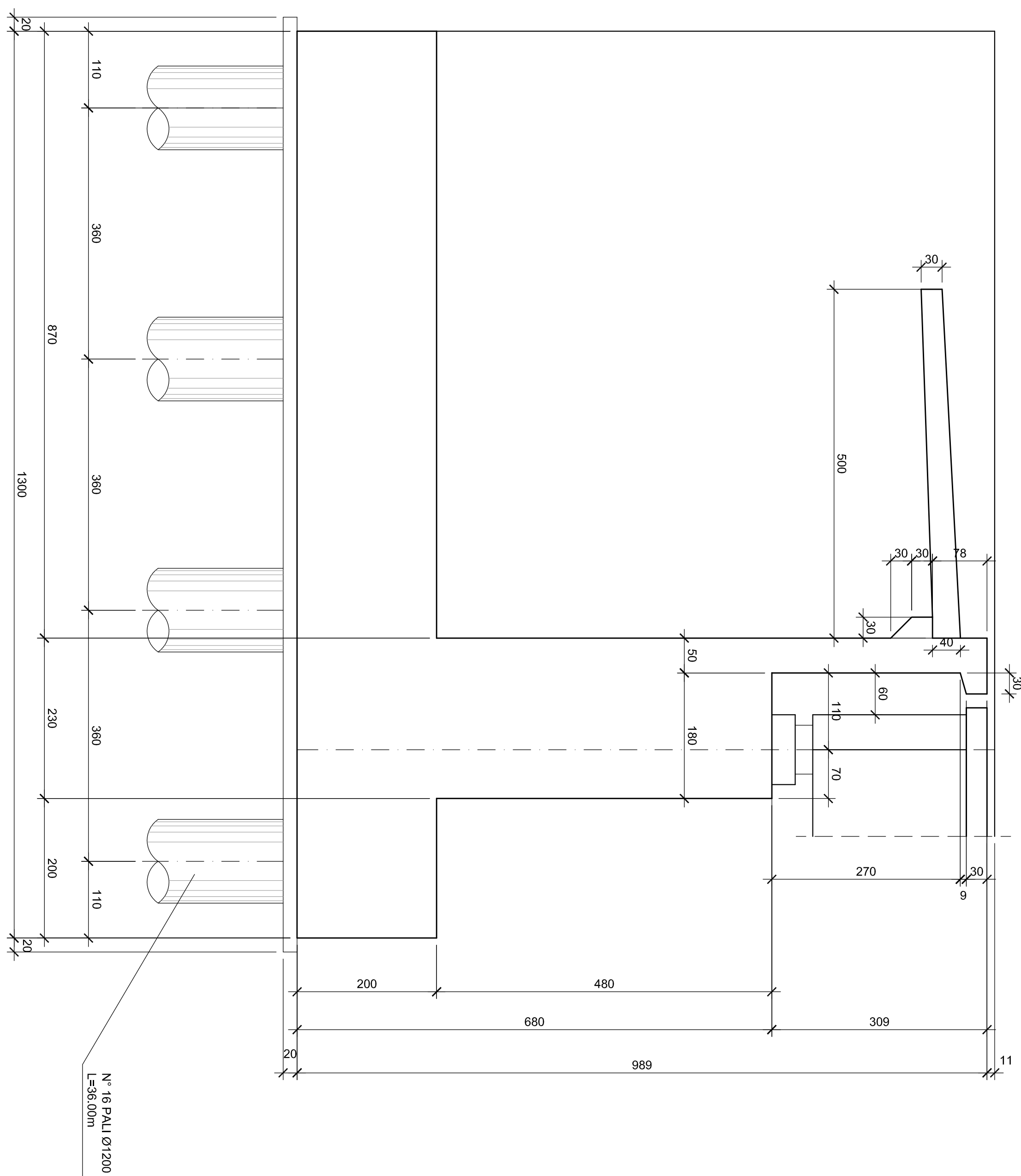
SEZIONE A-A 1:50
