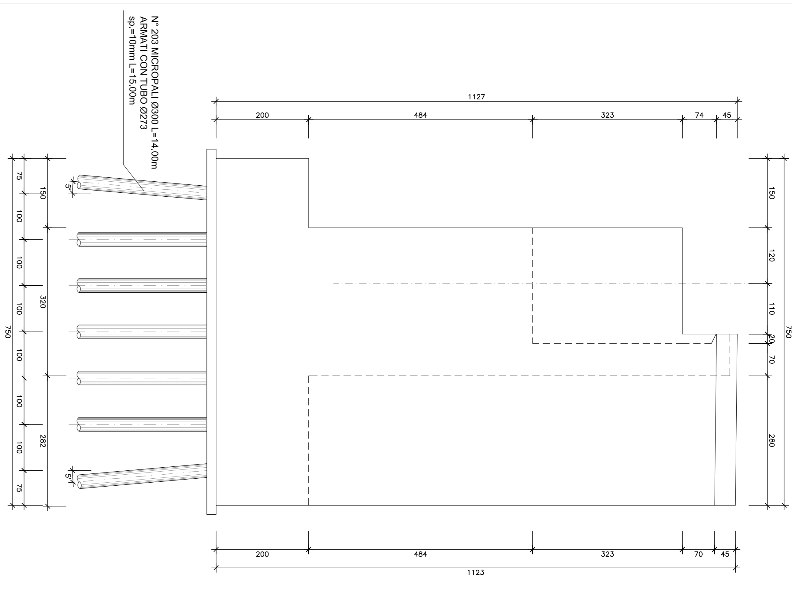
SCALA 1:50
