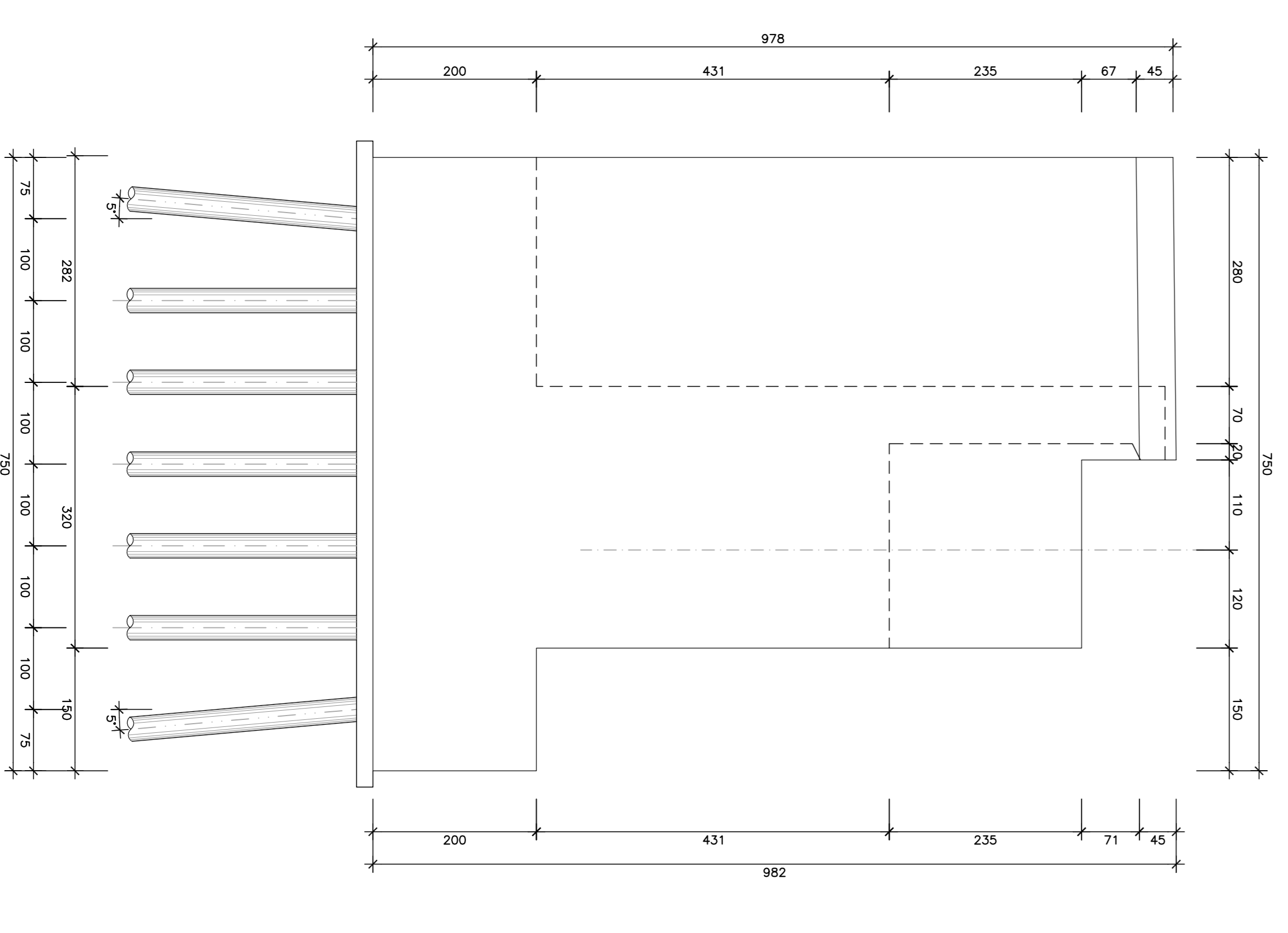
SCALA 1:50
