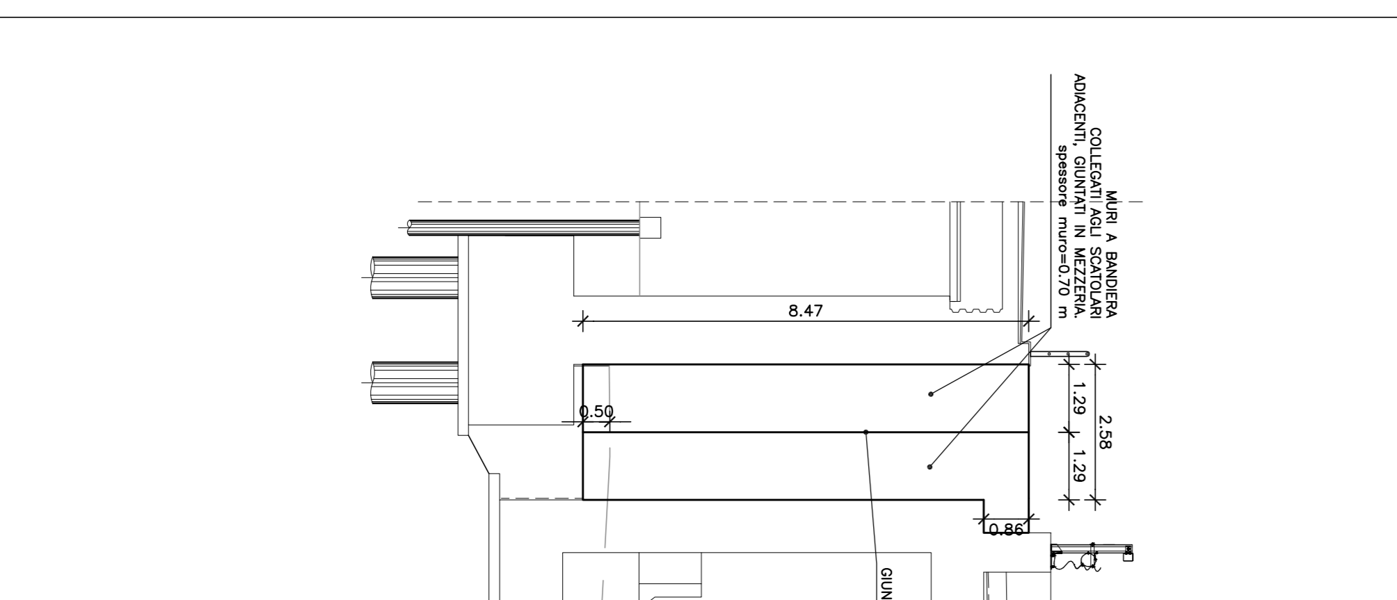
VISTA ALLA PROSP. 0+48.50 - MUR DI CHIUSURA SUD
