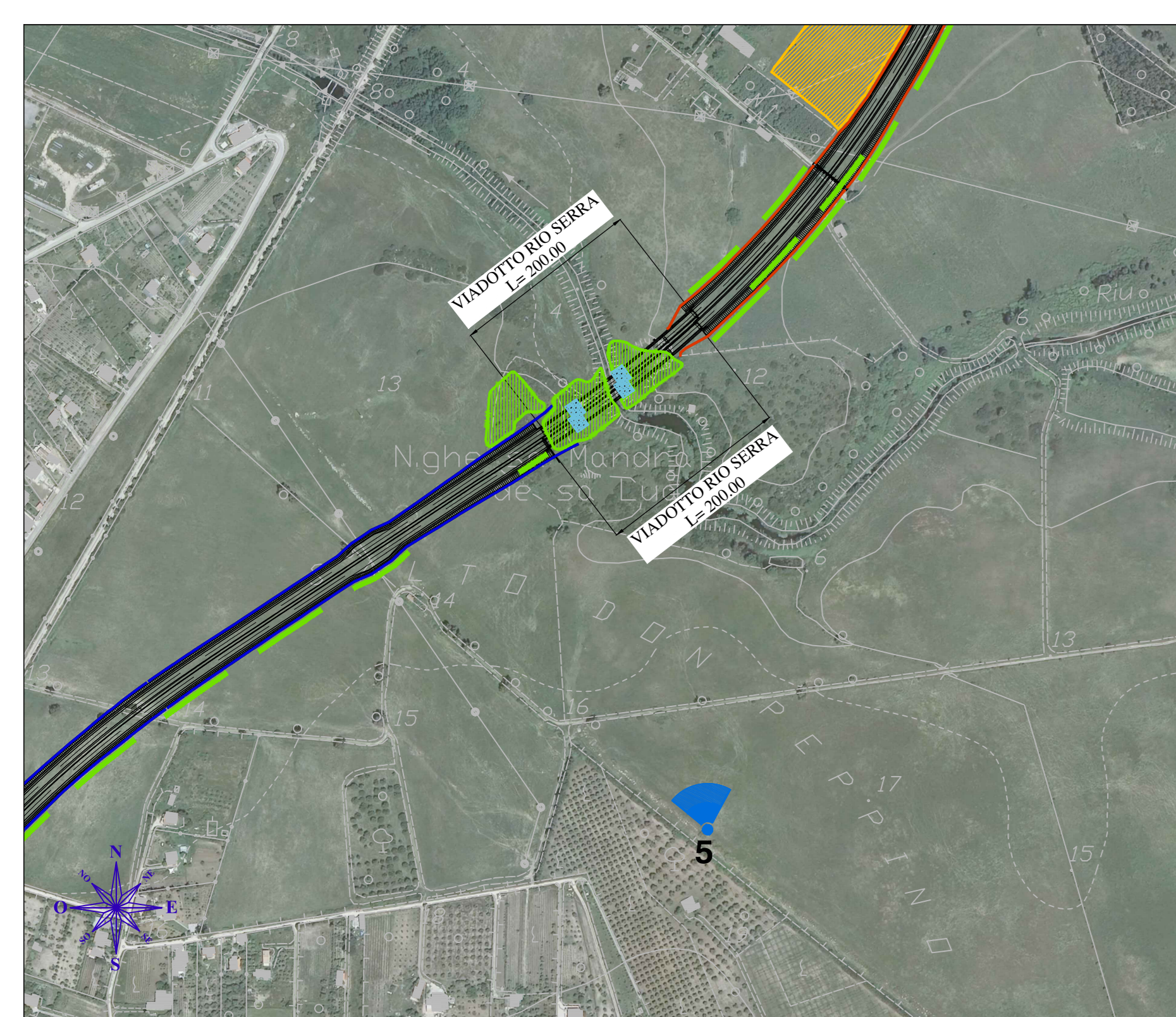
Foto 5 - Post operam - Viadotto Serra
