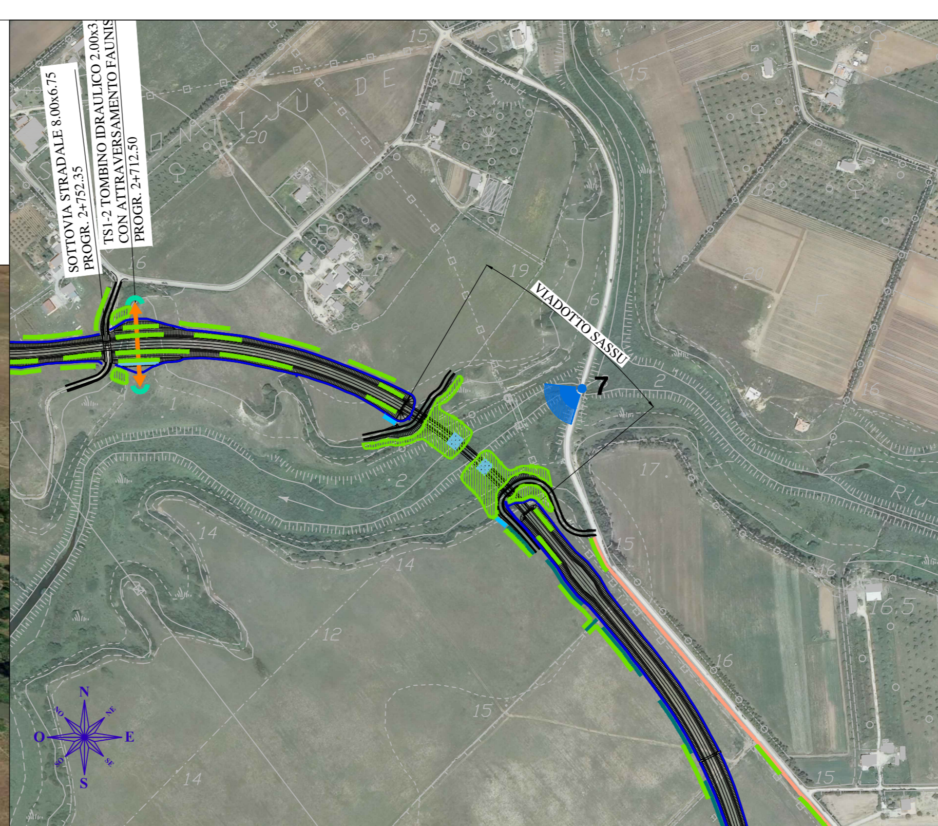
Foto 6 - Post operam - Viadotto Sassu
