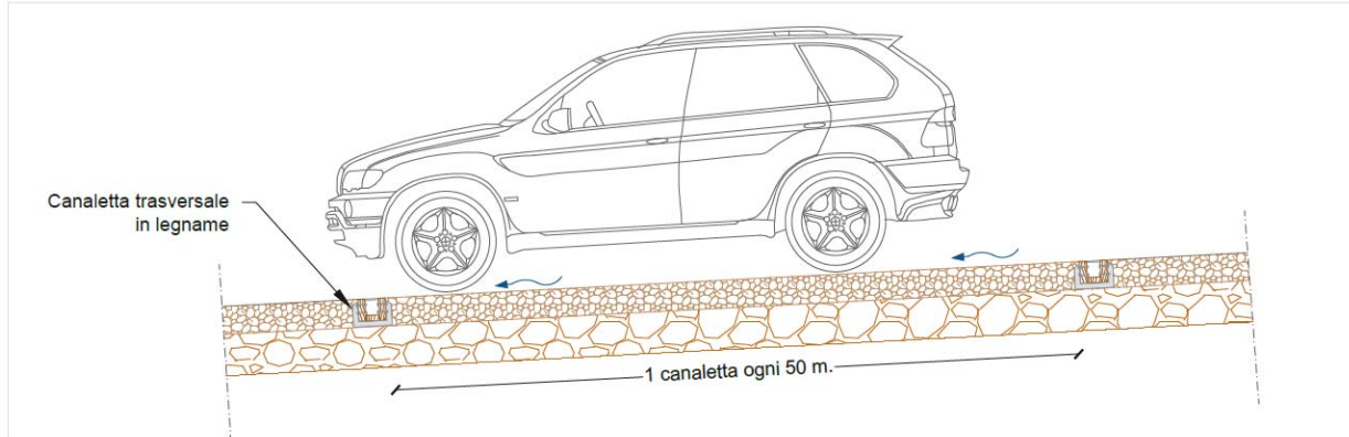
Figura 3.2: Sezione longitudinale con ubicazione delle canalette in legno.
