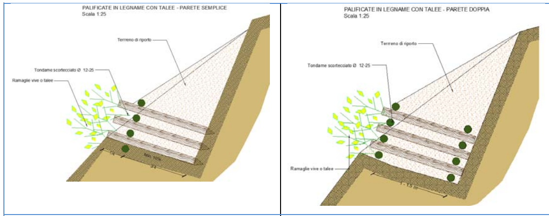
Esempio di palificate in legname - Fonte HE
