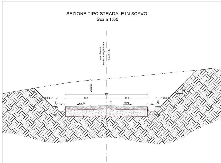
Figura 6: Sezione tipo di strada in scavo
