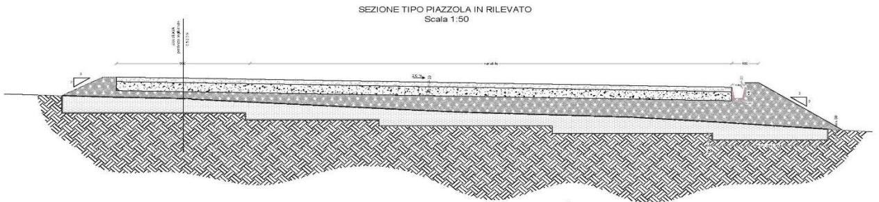
Fig.10 Sezione tipo della piazzola
