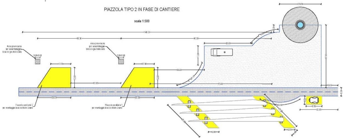
Fig.9 Pianta di una piazzola tipo in fase di cantiere
