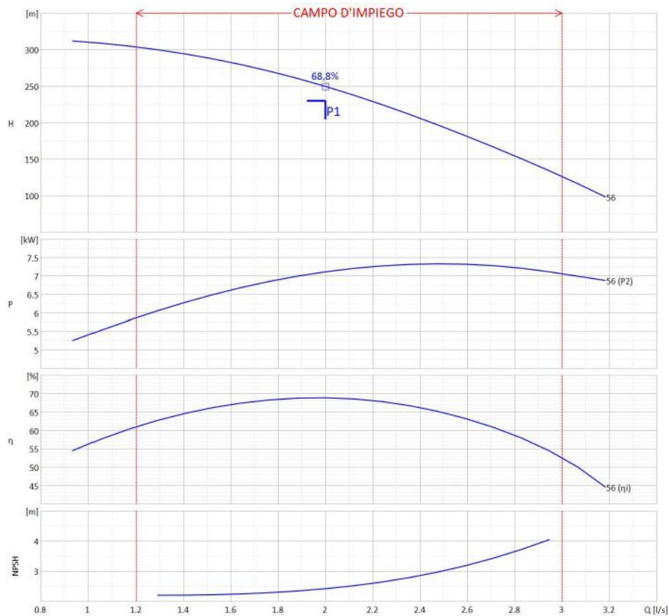
Figura 8 – Caratteristiche di esercizio della pompa prevista.
