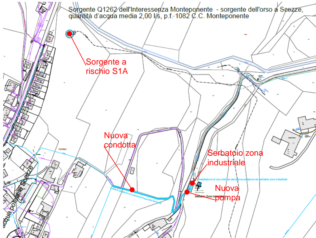
Figura 6 – Stralcio planimetrico della soluzione progettuale proposta dal gestore.
