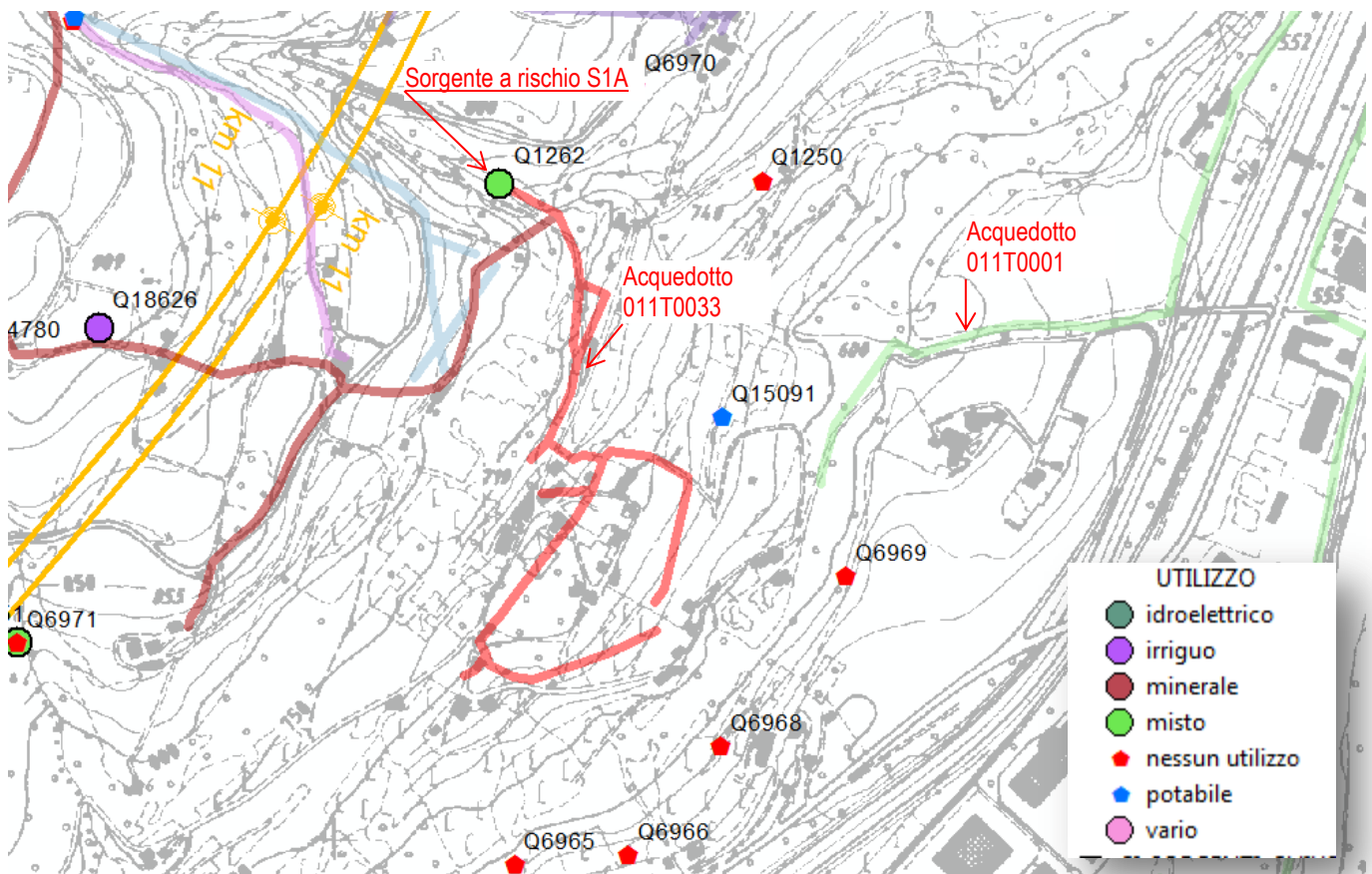
Figura 5 – Stralcio planimetrico delle sorgenti e delle reti acquedottistiche nei pressi della sorgente a rischio.
