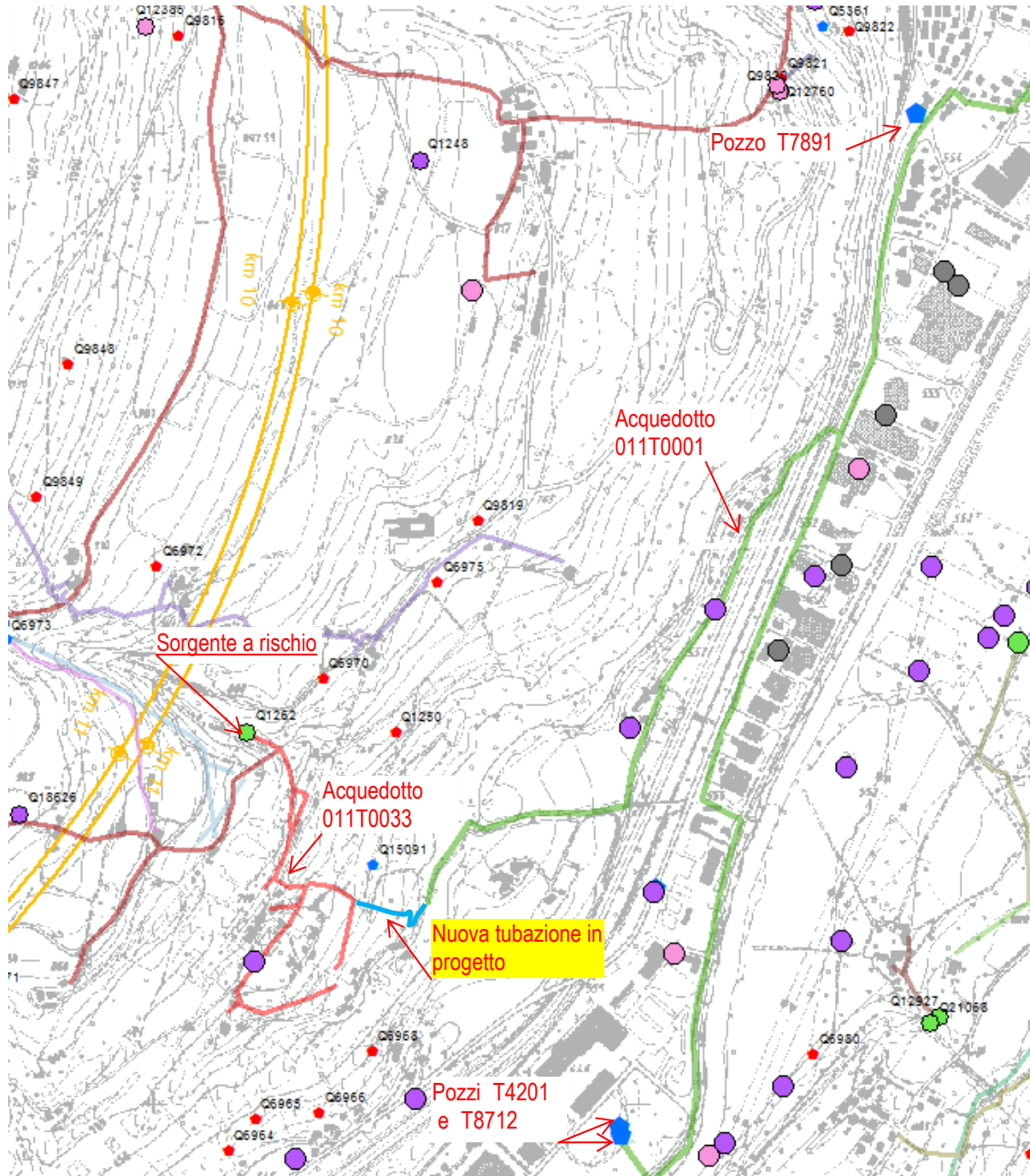
Figura 7 – Stralcio planimetrico della soluzione progettuale con indicazione delle reti acquedottistiche e dei pozzi di compensazione.
