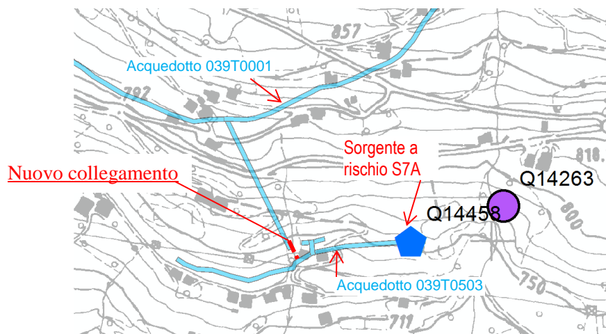
Figura 6 – Schema della soluzione proposta per la compensazione del depauperamento della sorgente S7.
