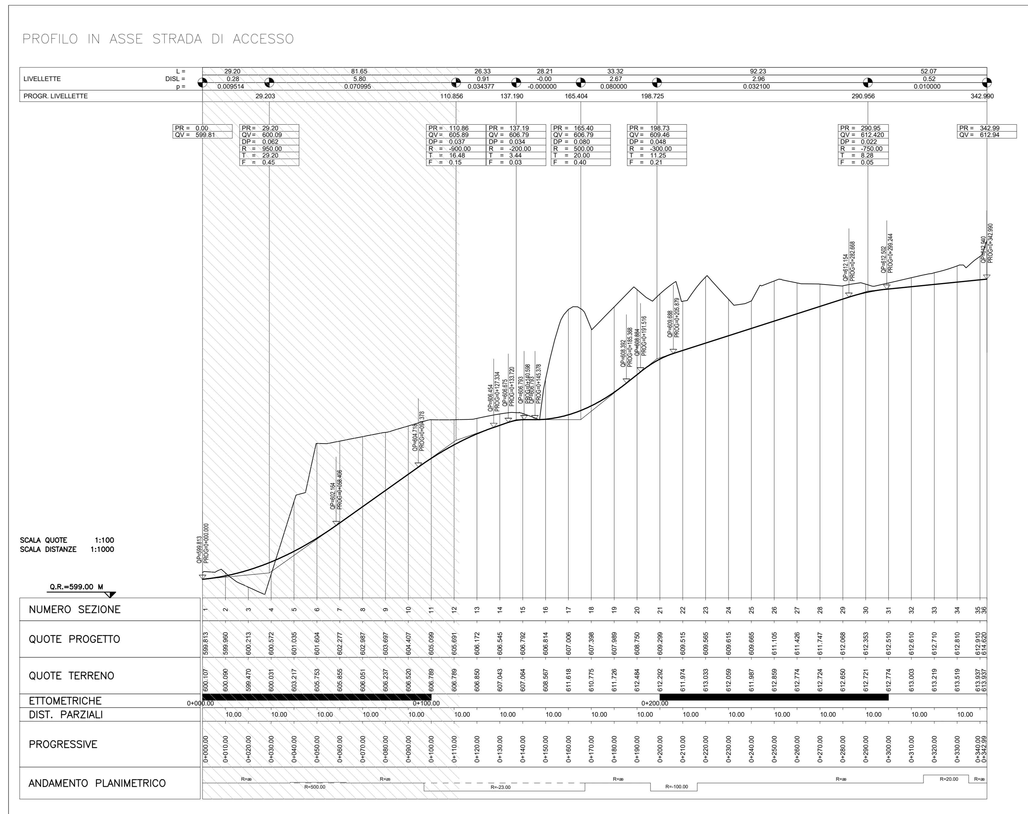
Profilo altimetrico Scala 1:1000/1:100
