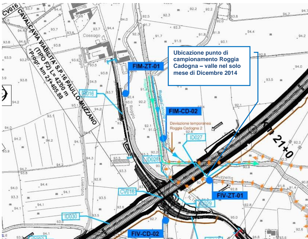
Figura 3-39: deviazione temporanea Roggia Cadogna 2.
