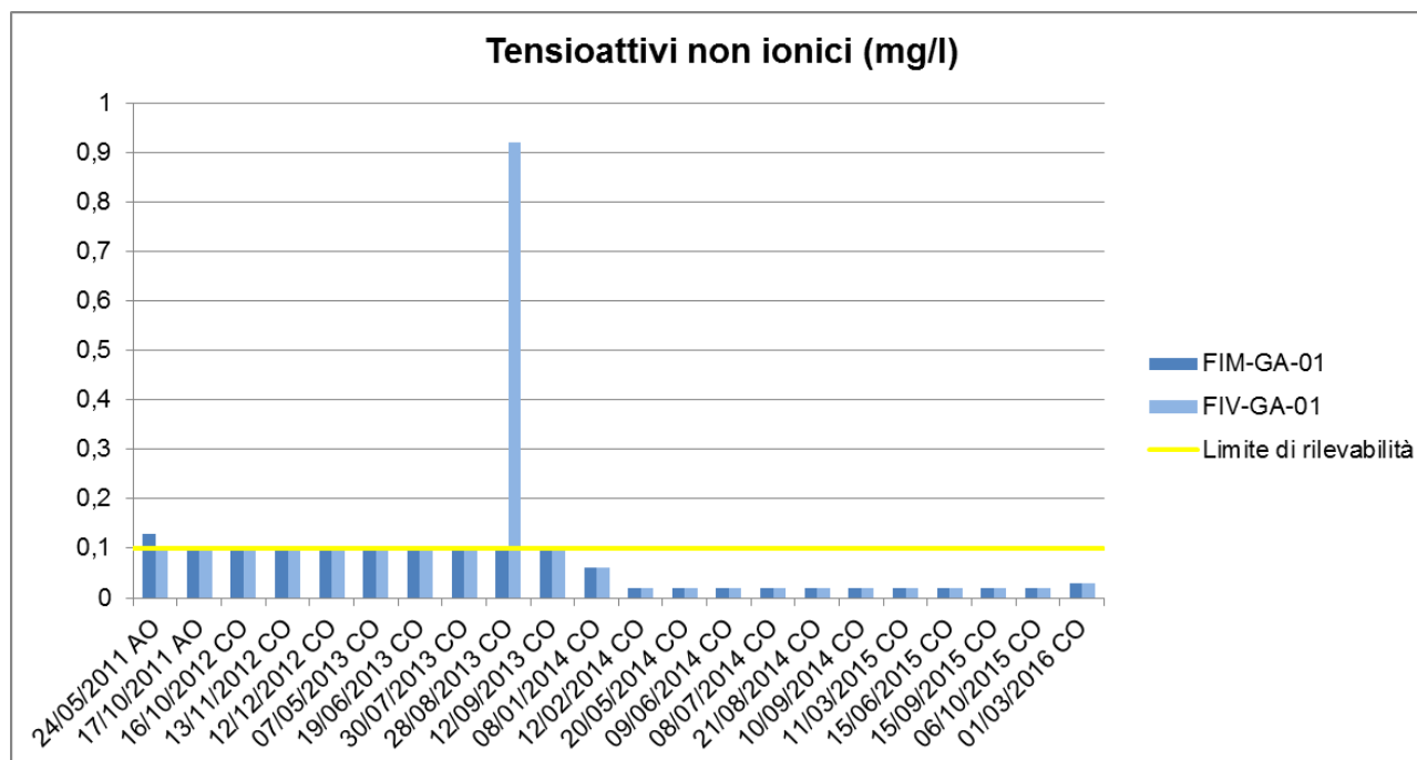
Figura 3-8: andamento nel tempo della concentrazione di Tensioattivi non ionici (mg/L) presso la sezione di monte (FIM-GA-01) e la sezione di valle (FIV-GA-01) del Fontanile Gabbarella.
