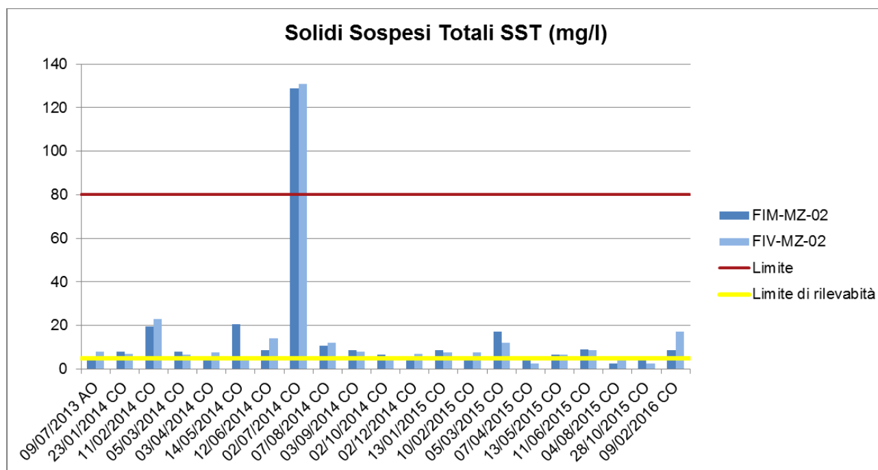
Figura 3-46: andamento nel tempo della concentrazione di SST (mg/l) presso la sezione di monte (FIM-MZ-02) e la sezione di valle (FIV-MZ-02) del Canale Muzza 2.
