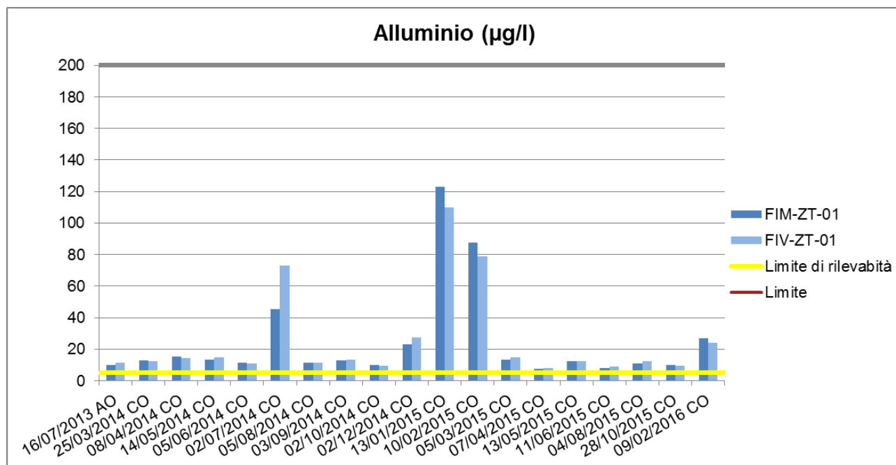
Figura 3-45: andamento nel tempo della concentrazione di Alluminio ( \mu\text{g/l} ) presso la sezione di monte (FIM-ZT-01) e la sezione di valle (FIV-ZT-01) della roggia Muzzetta.
