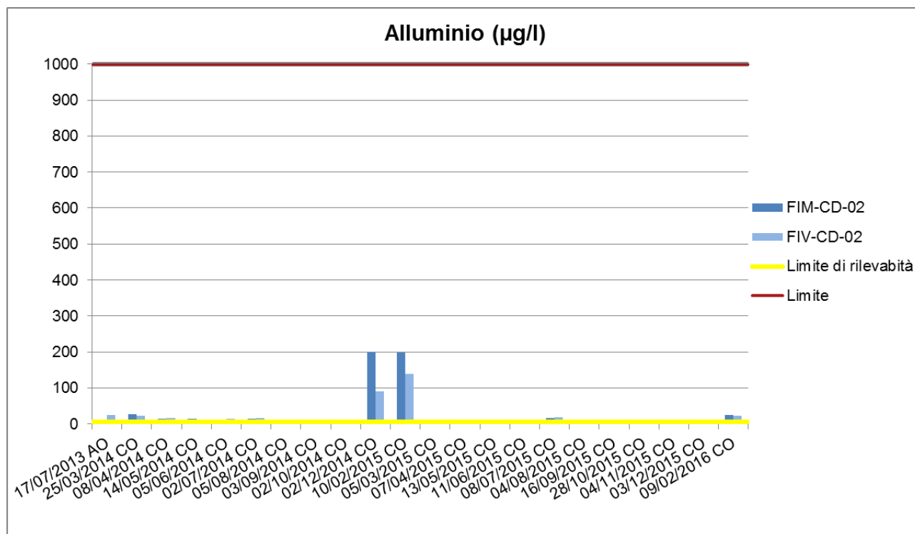
Figura 3-36: andamento nel tempo della concentrazione di Alluminio ( \mu\text{g/l} ) presso la sezione di monte (FIM-CD-02) e la sezione di valle (FIV-CD-02) della Roggia Codogna 2.
