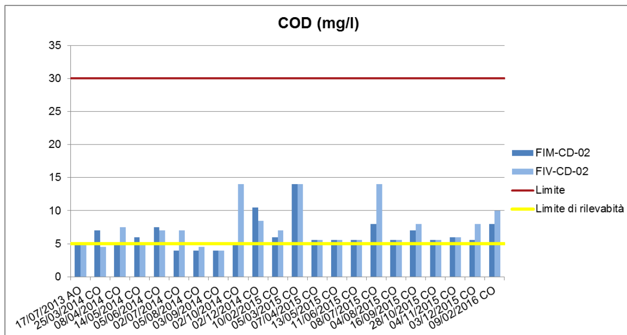
Figura 3-37: andamento nel tempo della concentrazione di COD (mg/l) presso la sezione di monte (FIM-CD-02) e la sezione di valle (FIV-CD-02) della Roggia Codogna 2.
