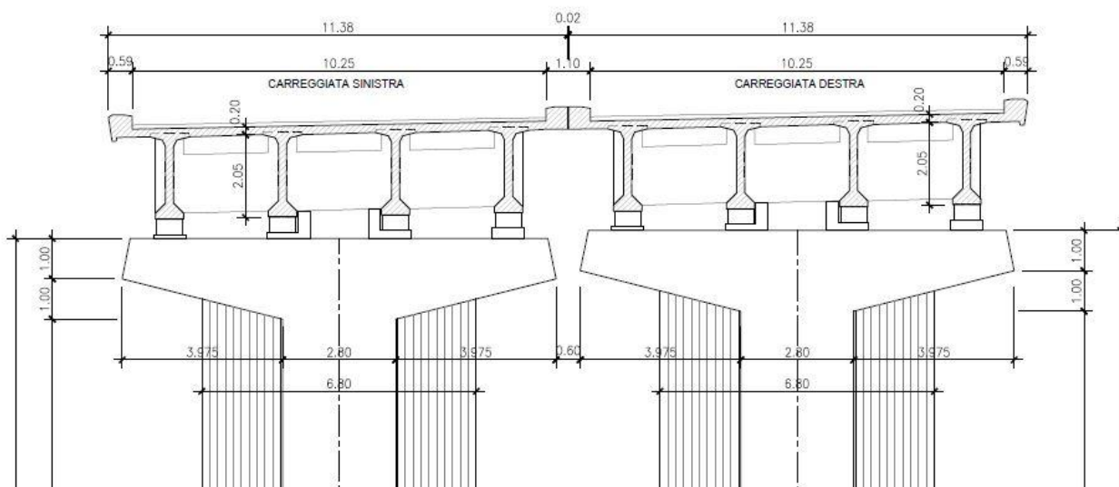
Figura 1: sezione tipica delle opere esistenti (fornaca)
