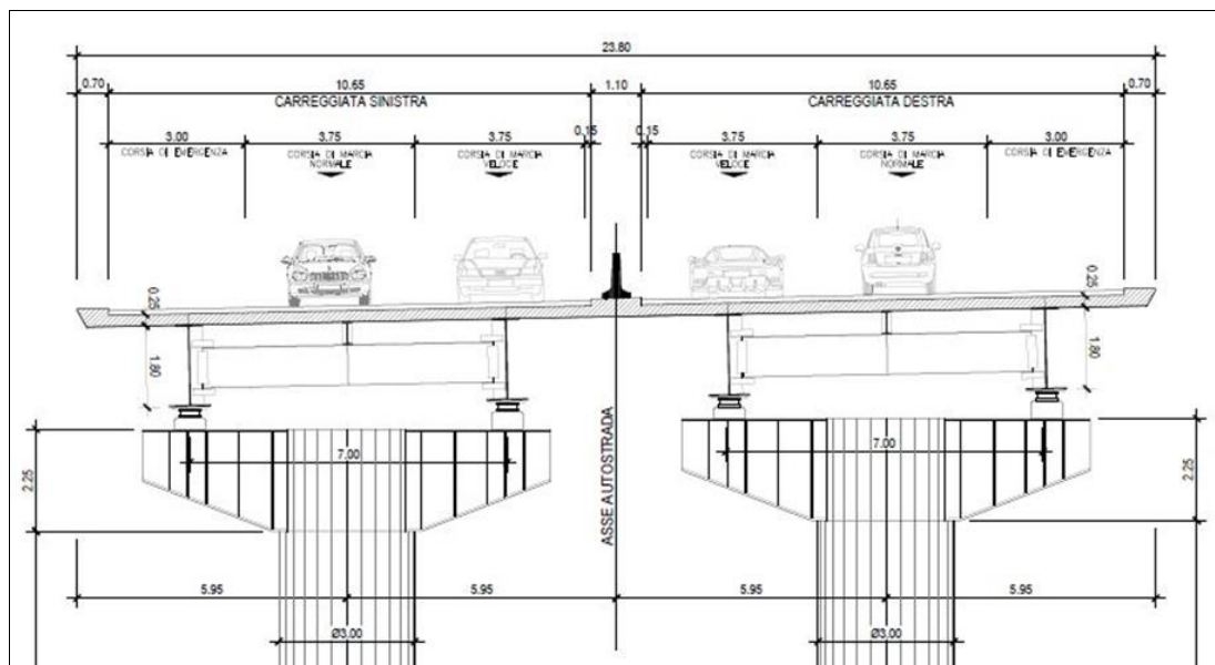
Figura 2: sezione tipo di progetto per carreggiate adiacenti
