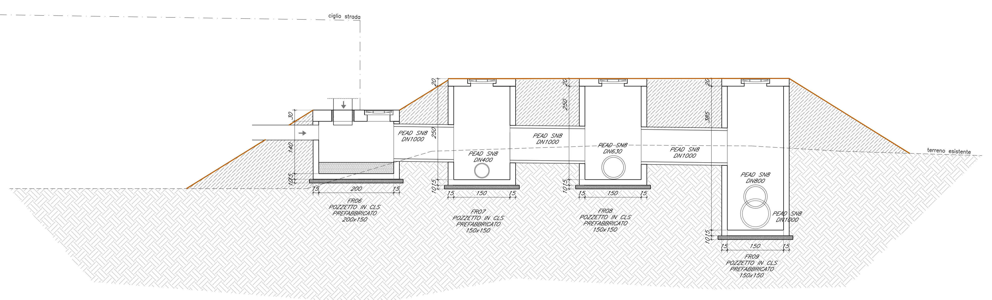
SEZIONE B-B - Scala 1:50
