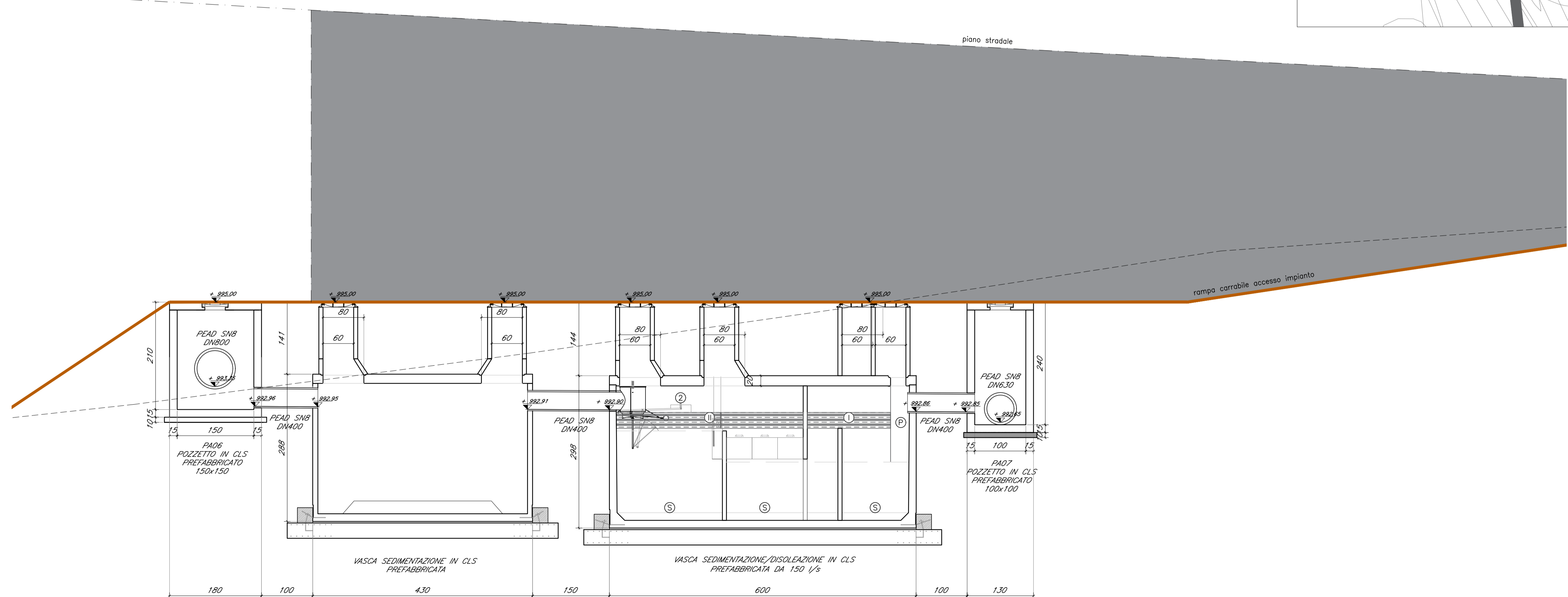
SEZIONE A-A - Scala 1:50
