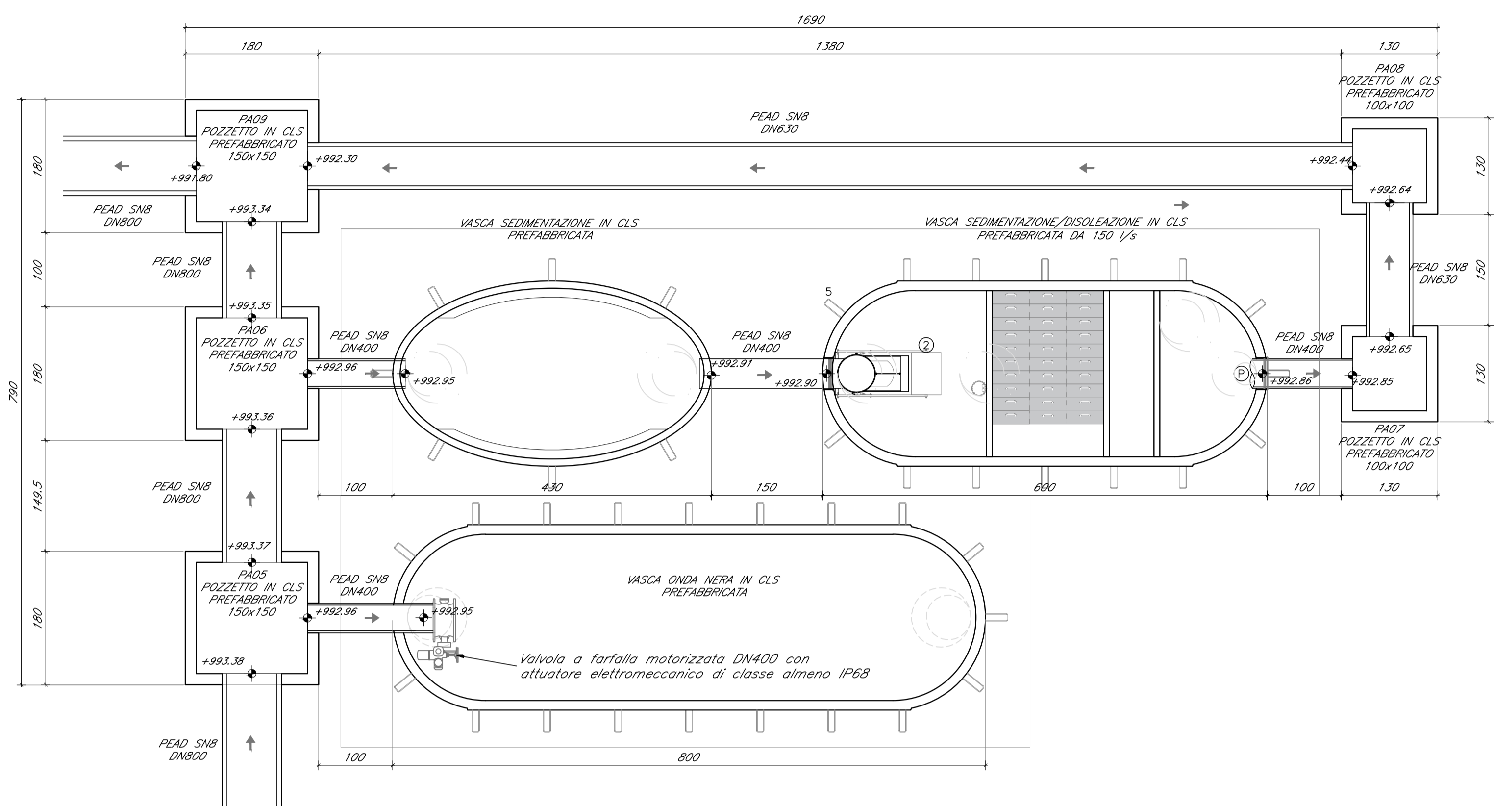
PLANIMETRIA - Scala 1:50
