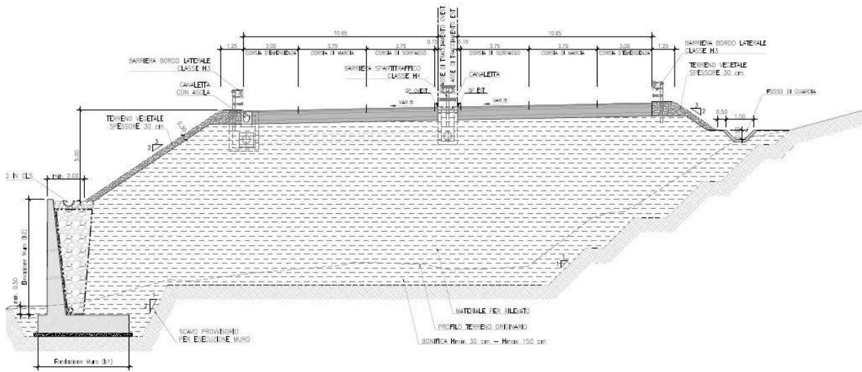
Figura 3. Sezione tipologica del rilevato stradale.
