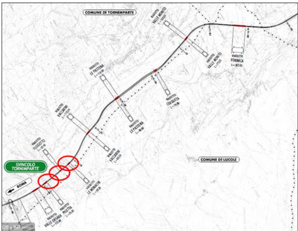
Figura 2. Inquadramento territoriale dei viadotti oggetto di adeguamento.
