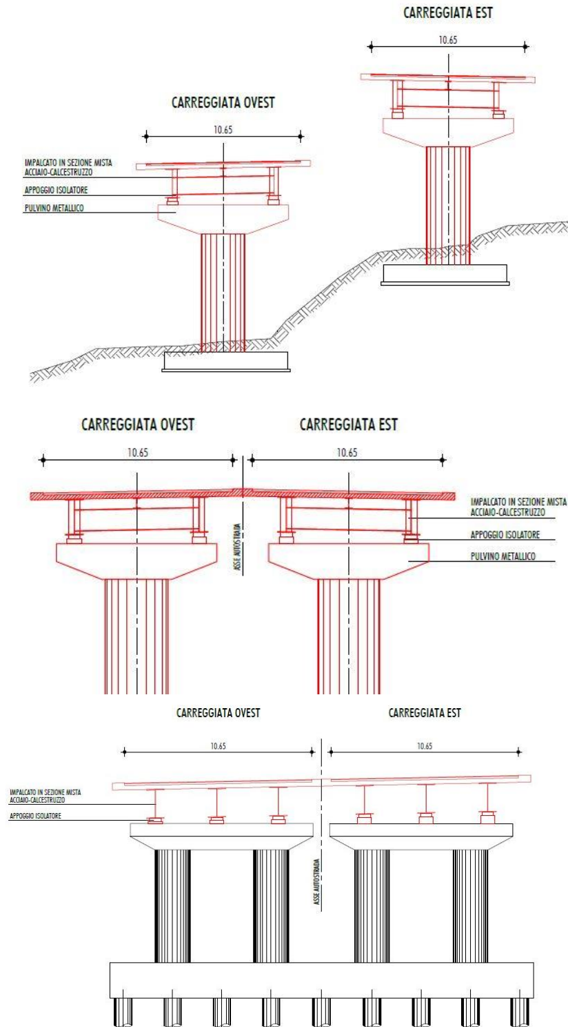
Figura 2. Rappresentazione schematica dell'intervento.
