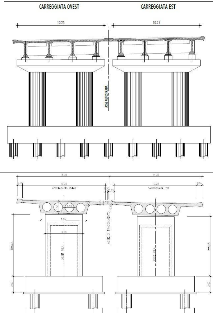
Figura 2: sezione tipologica dello stato attuale (opere a travi: viadotti Raio e Aterno; solettoni: SS17, Vetoio e rampa)
