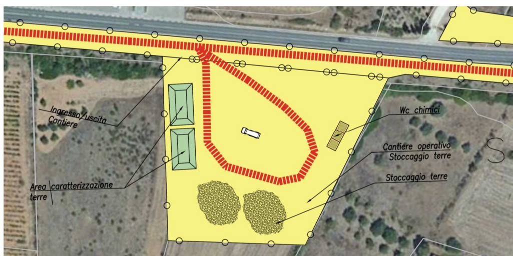
Layout tipologico Cantiere Operativo
