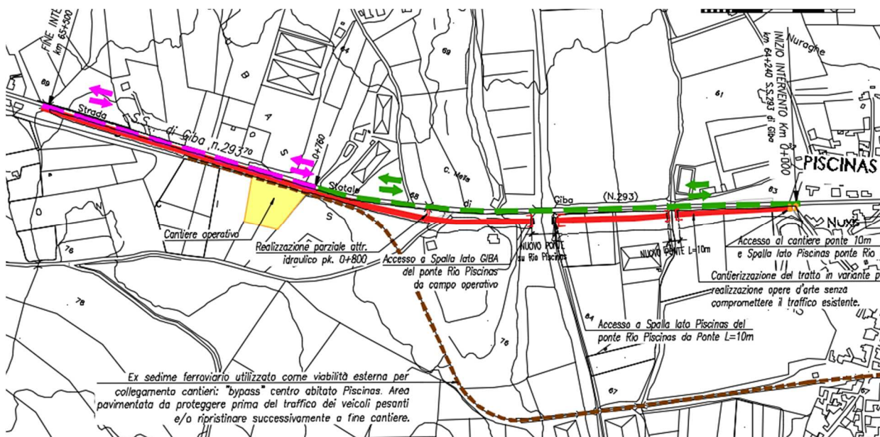
S.S. 293 - FASE 2 – Planimetria del Tratto 2
