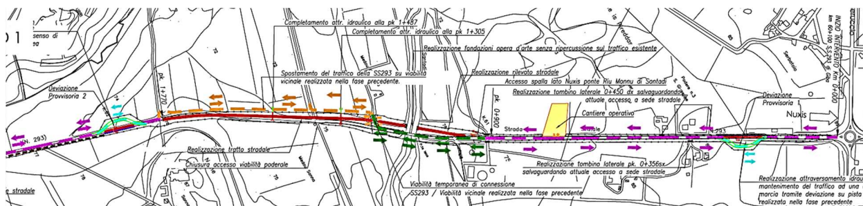
S.S. 293 - FASE 2 – Planimetria del Tratto 1 da inizio intervento a pk. 2+200 ca.
