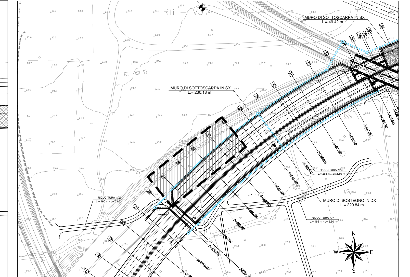
PLANIMETRIA con indicazione della tratta oggetto della tavola-Scala 1:2.000
