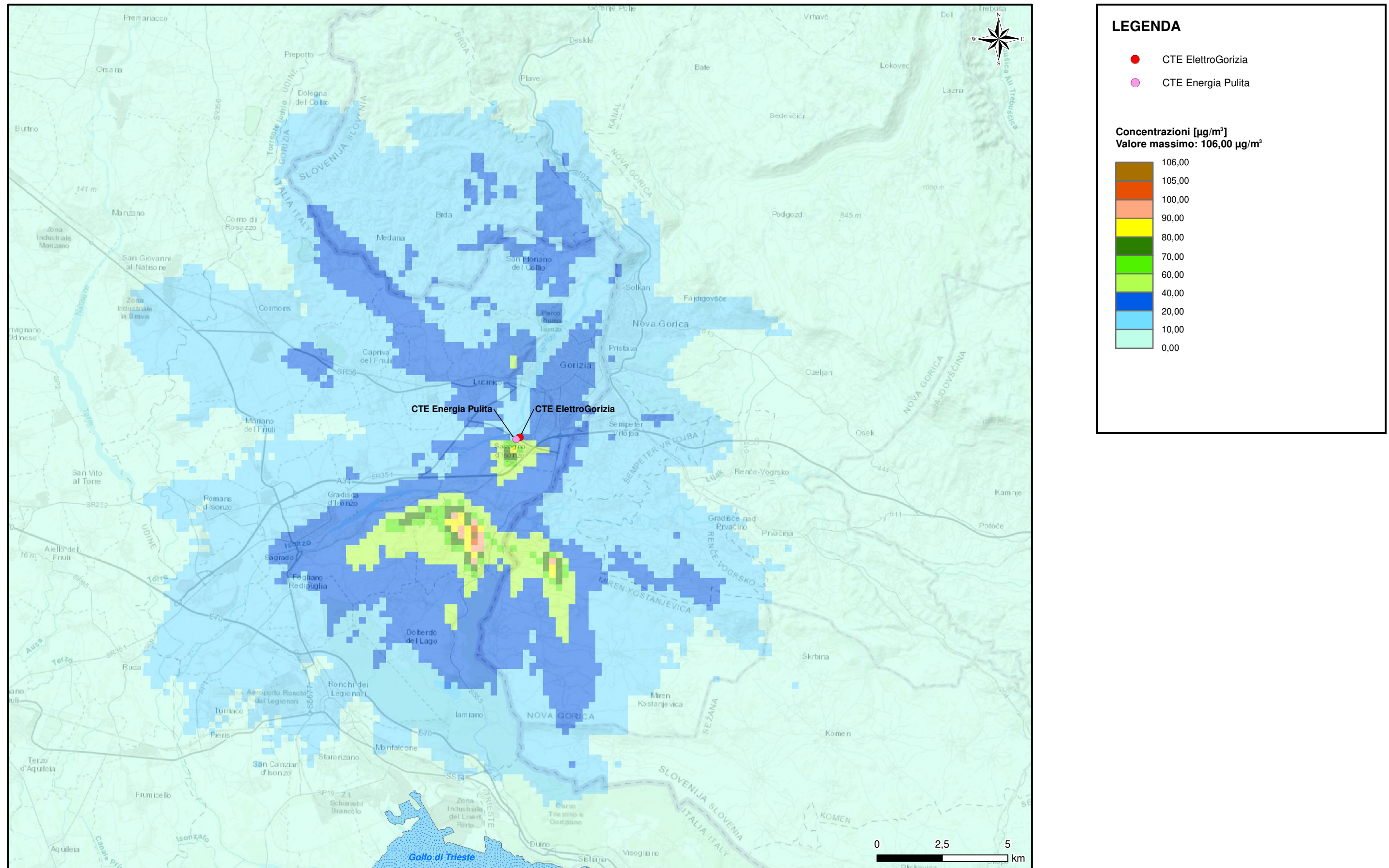
Figura 3.6a 99,8° percentile delle concentrazioni medie orarie di NOx - Scenario "ELETTRGORIZIA+ENERGIA PULITA"
