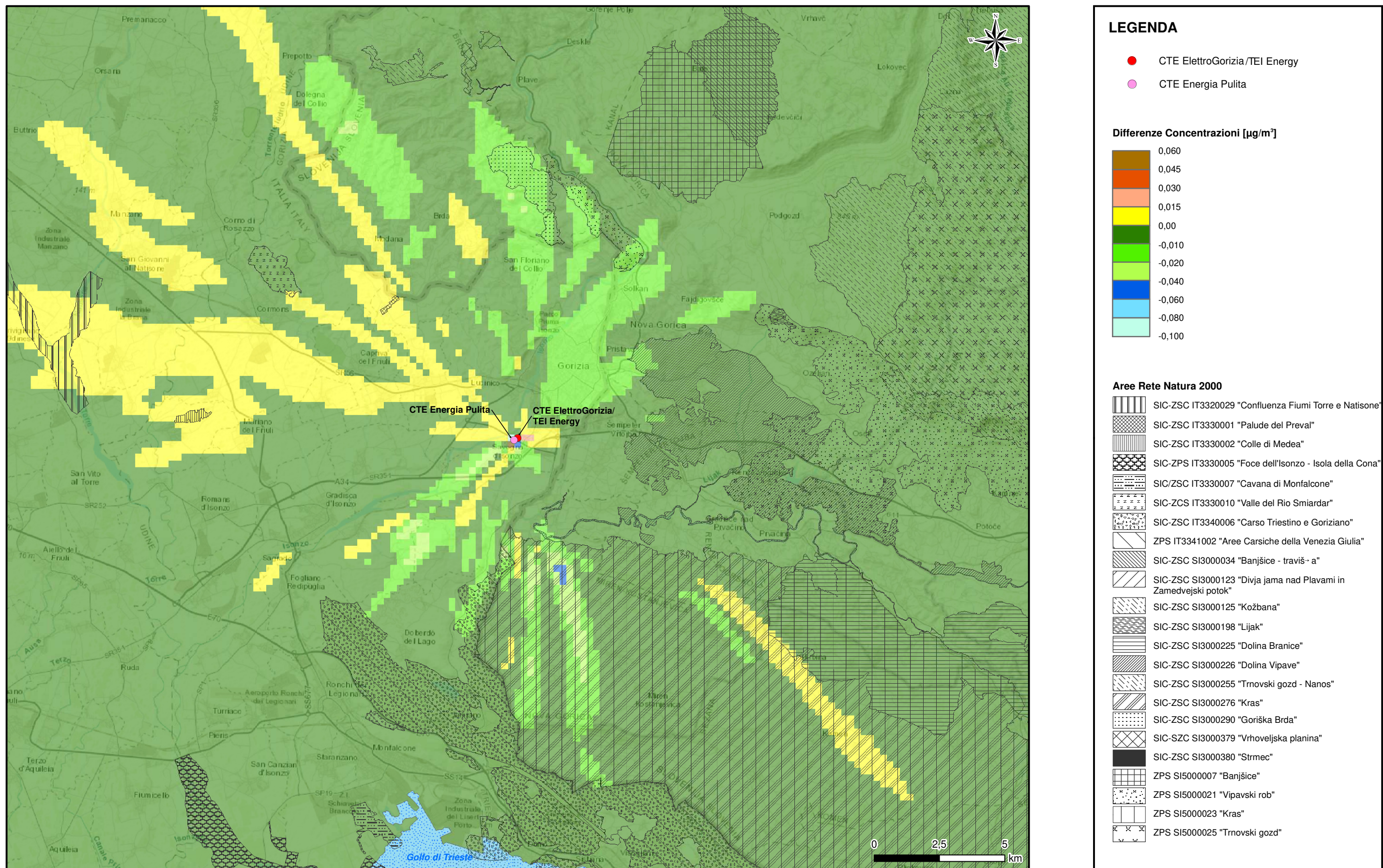
Figura 3.6f Differenza tra Scenario "TEI ENERGY+ENERGIA PULITA" e Scenario "ELETTRGORIZIA+ENERGIA PULITA": concentrazione media annua di NOx
