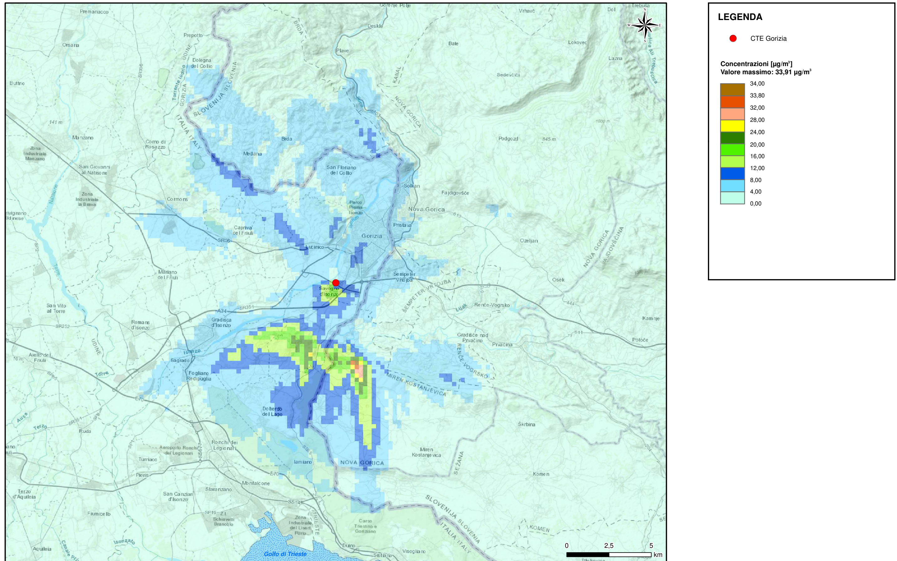
Figura 4.2a 99,8° percentile delle concentrazioni medie orarie di NOx
