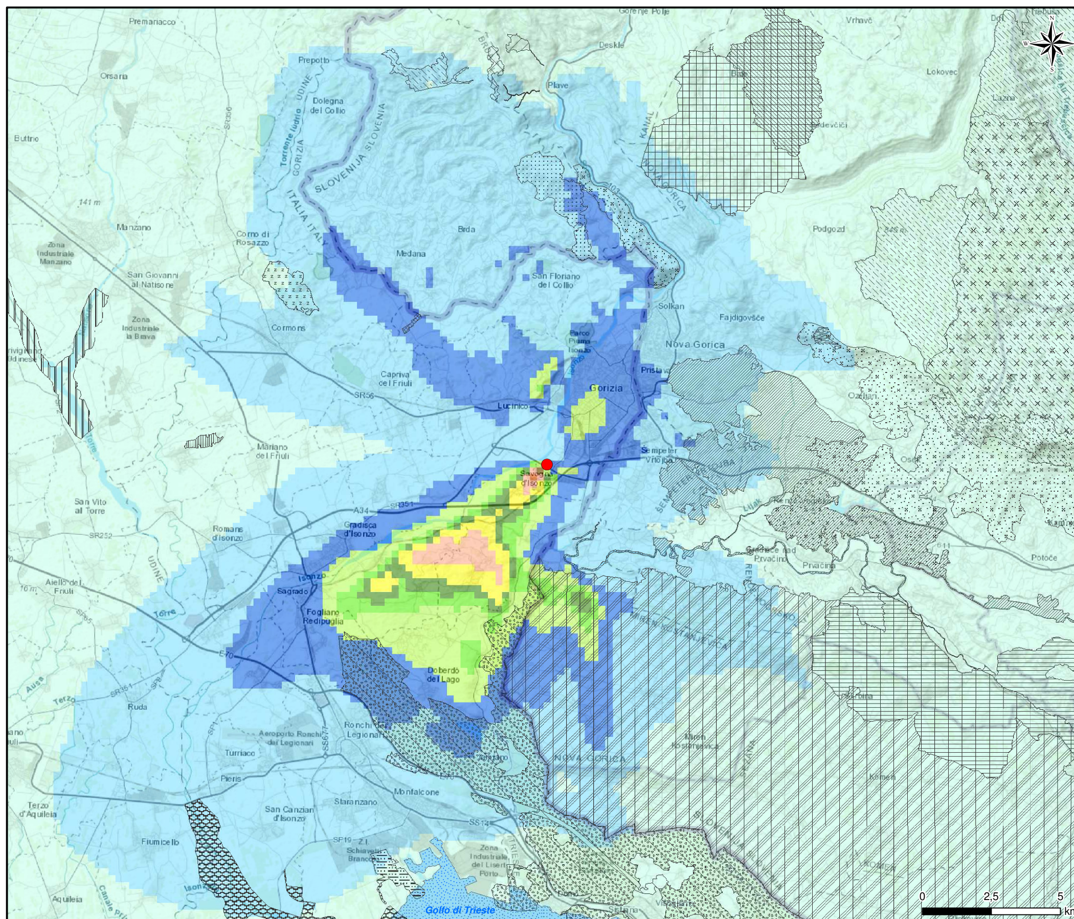
Figura 4.2b Concentrazione media annua NOx
