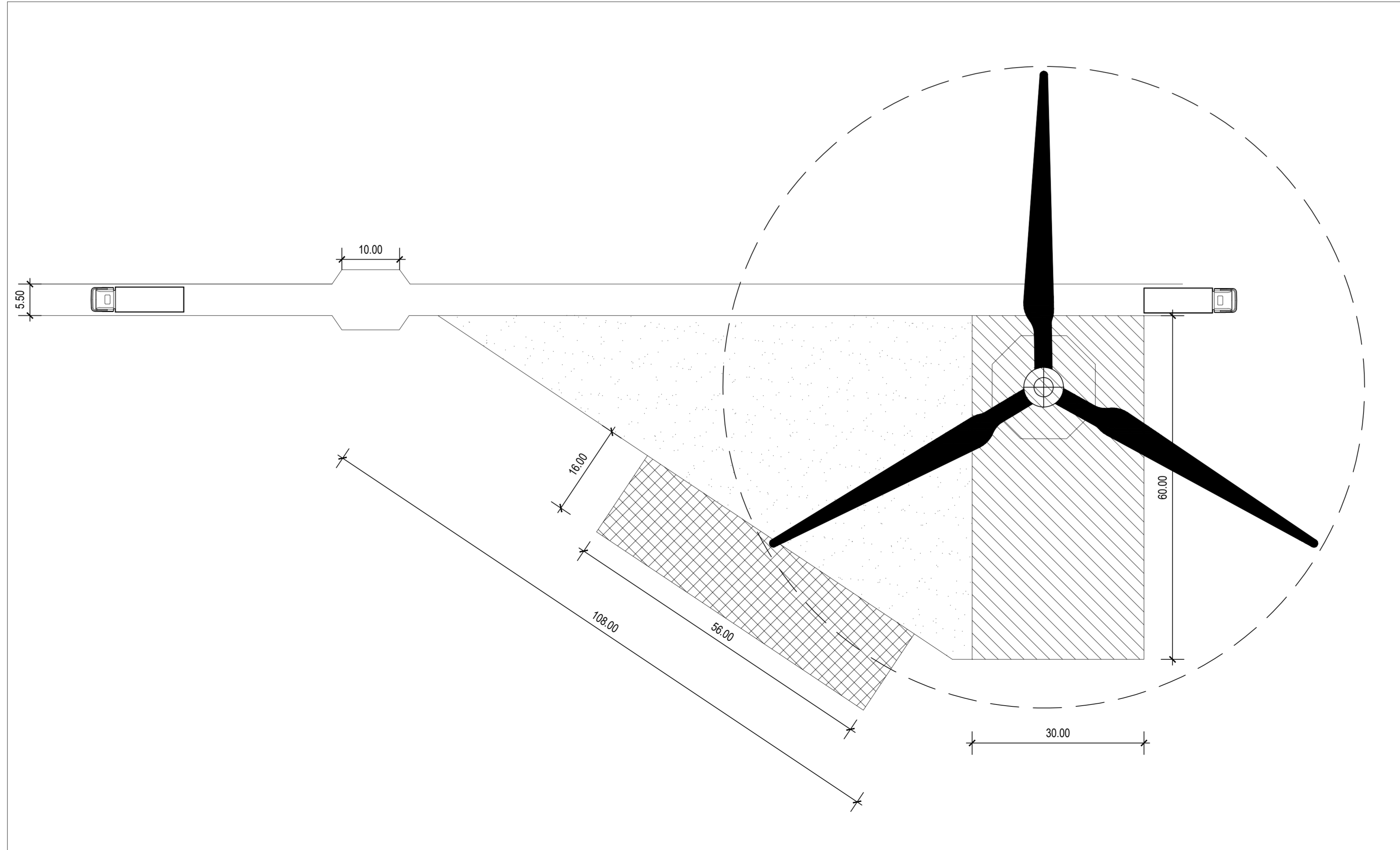
PIAZZOLA DI MONTAGGIO - TIPO 2 - PIANTA
