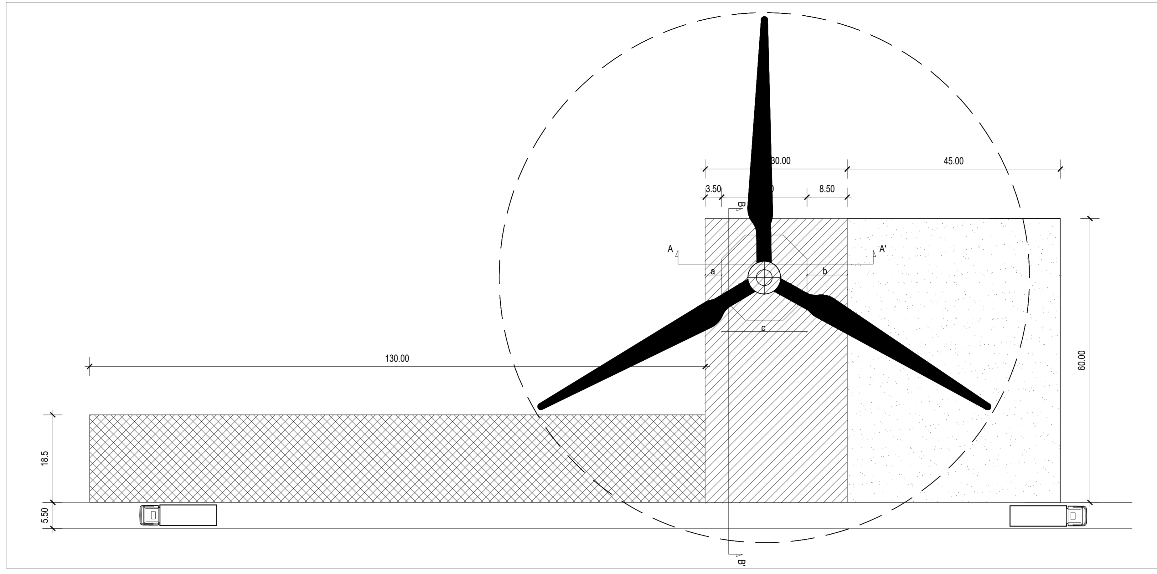
PIAZZOLA DI MONTAGGIO - TIPO 1 - PIANTA
