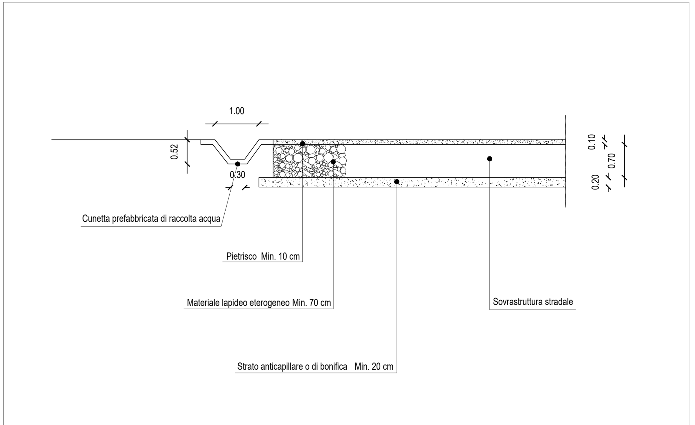
PIAZZOLA - SEZIONE TIPO
