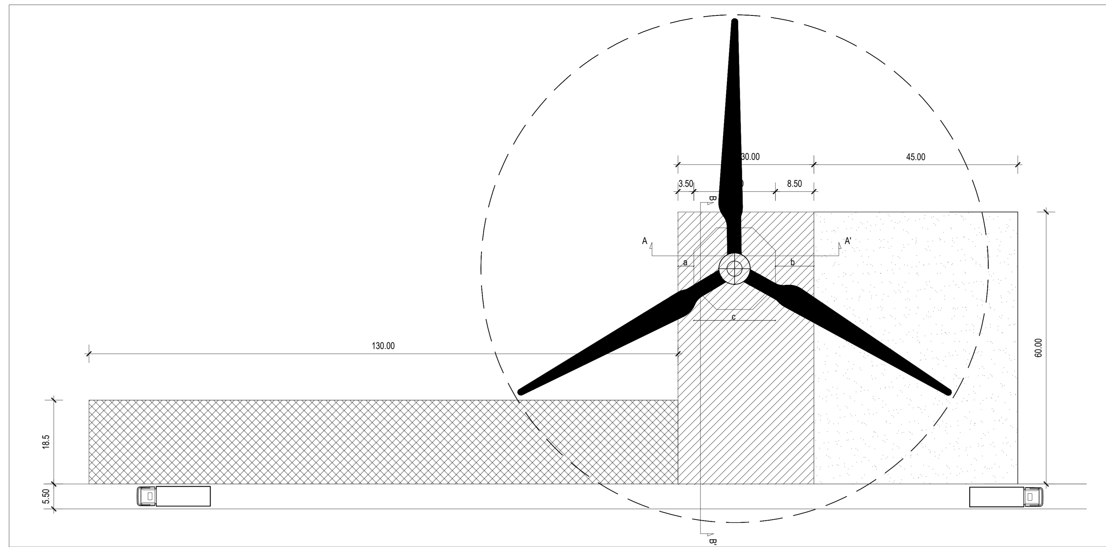
PIAZZOLA DI MONTAGGIO - TIPO 1 - PIANTA SCALA 1:500
