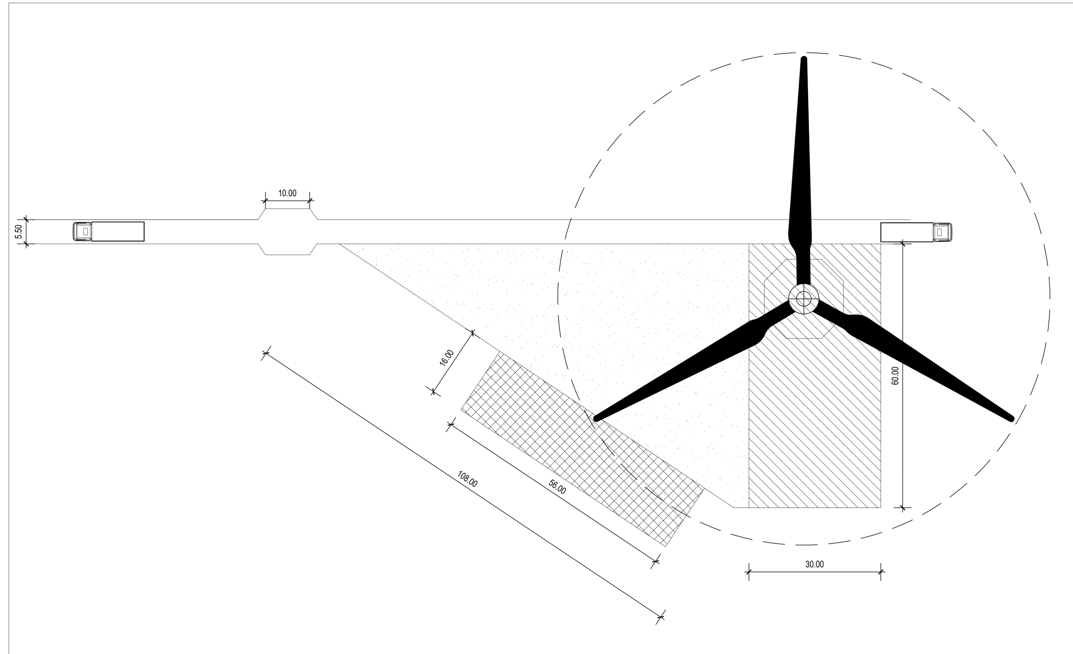
PIAZZOLA DI MONTAGGIO - TIPO 2 - PIANTA SCALA 1:500
