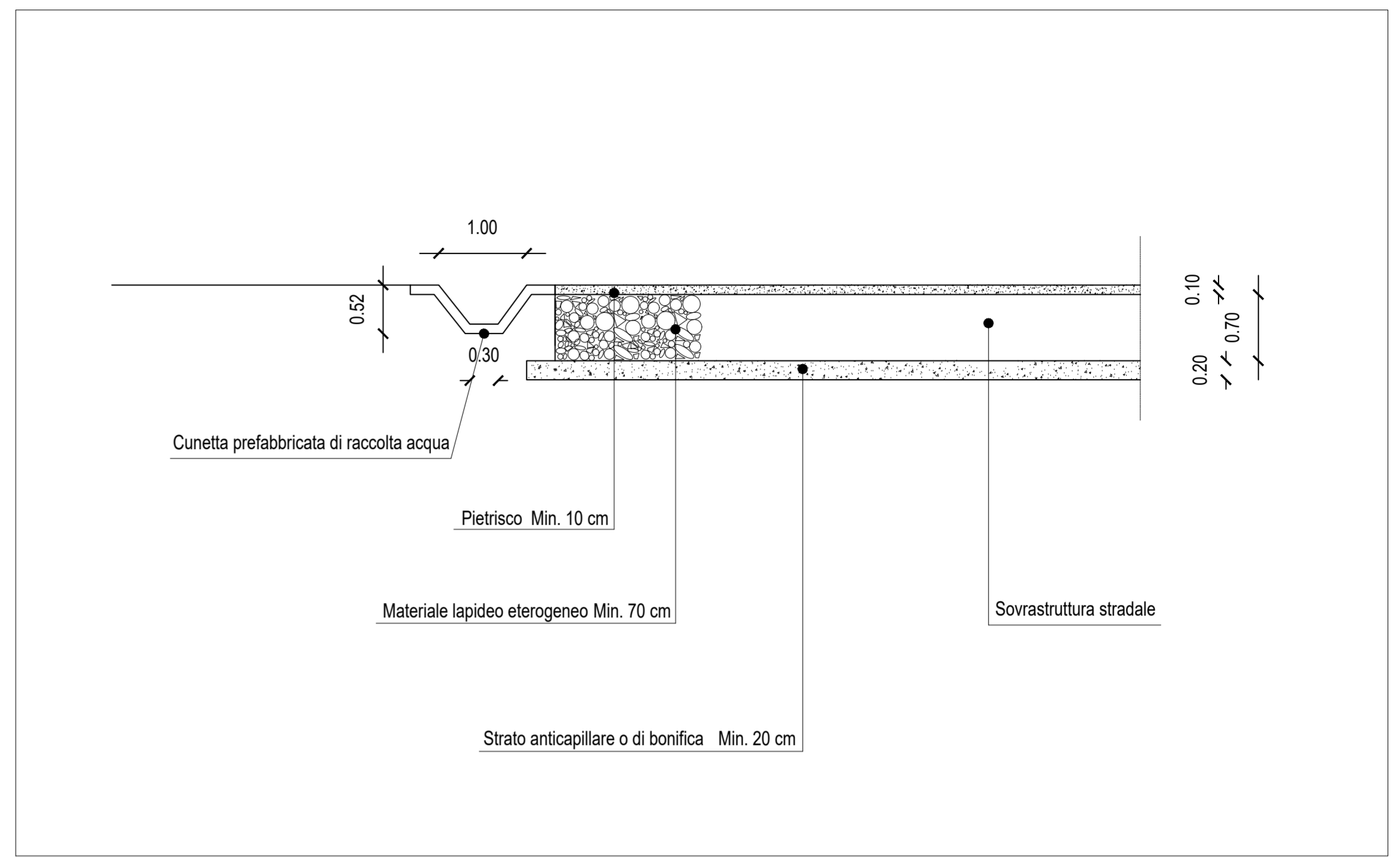
PIAZZOLA - SEZIONE TIPO SCALA 1:50
