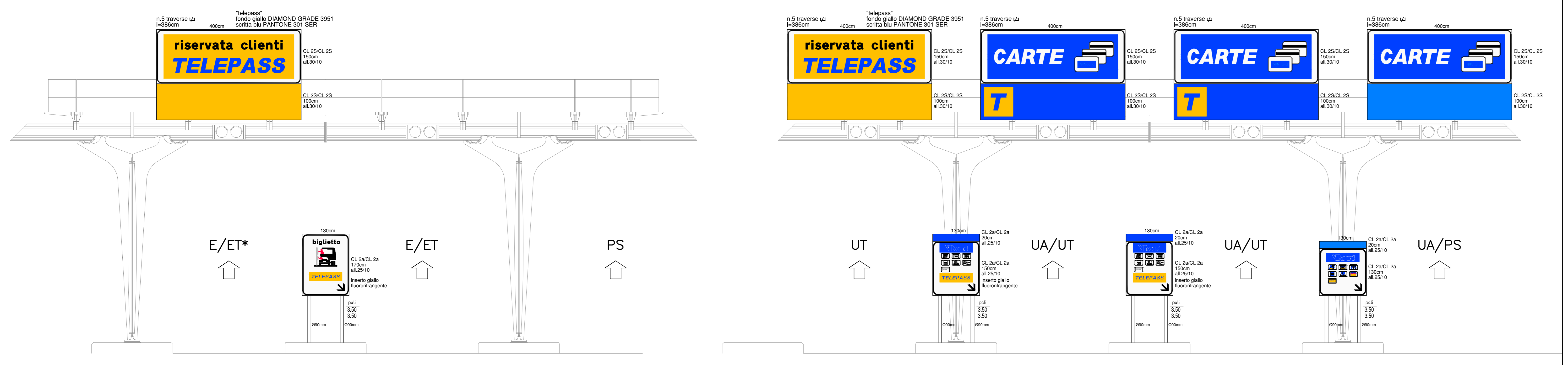
VISTA LATO ENTRATE Rapp. 1:50
