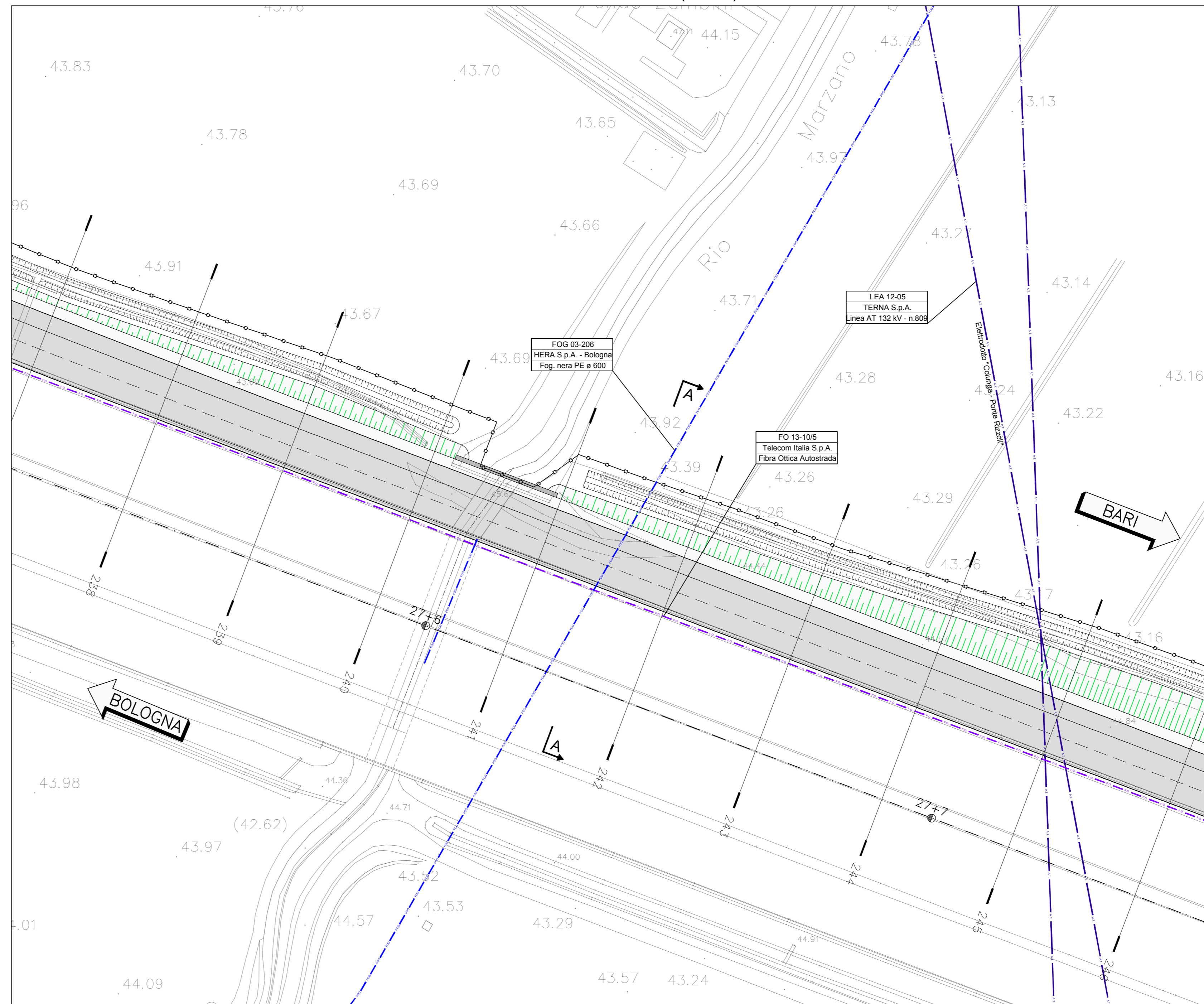
PIANTA PROGETTO (1:500)
