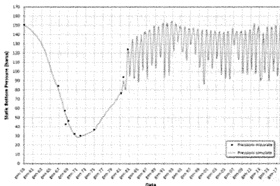
Confronto tra l'andamento della pressione statica simulata e i dati di pressione statica misurati per il pozzo Minerbio 34dir
