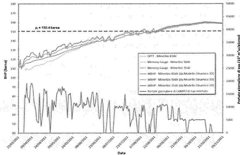
Andamento dei valori di pressione al fondo misurati e simulati in corrispondenza dei pozzi utilizzati per il monitoraggio in continuo
