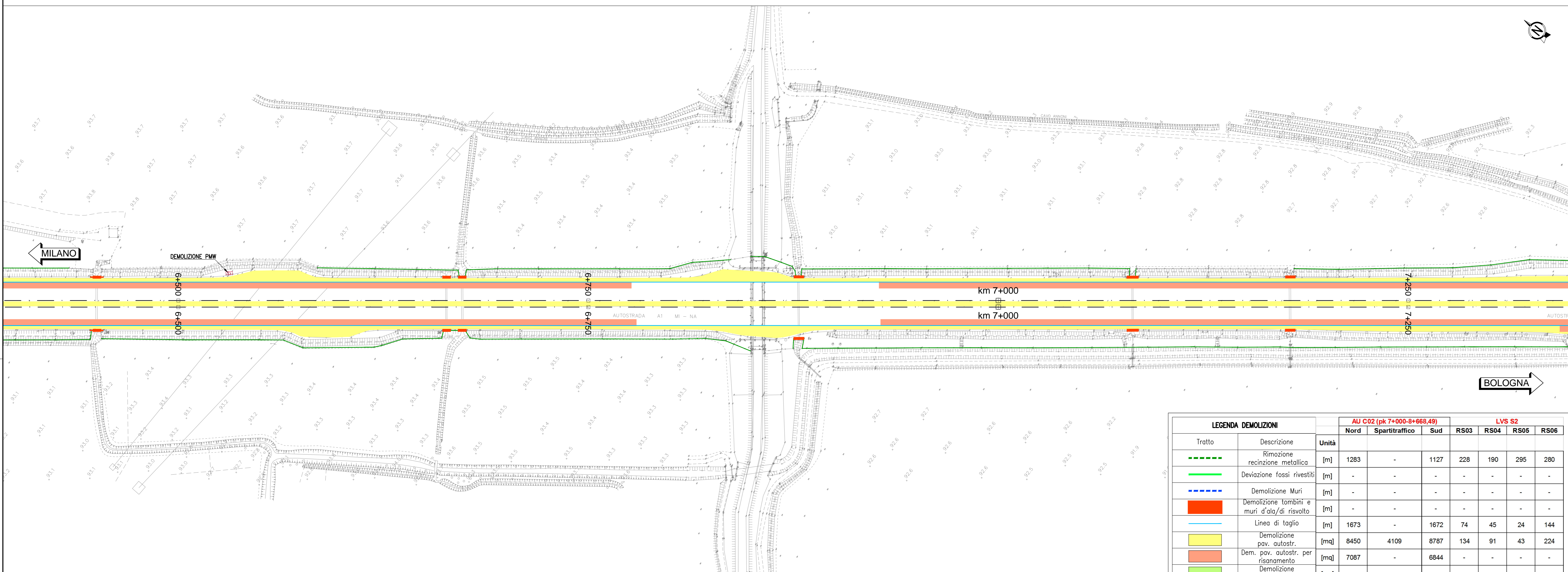
PLANIMETRIA (1:1.000) da km 6+420 a km 7+340
