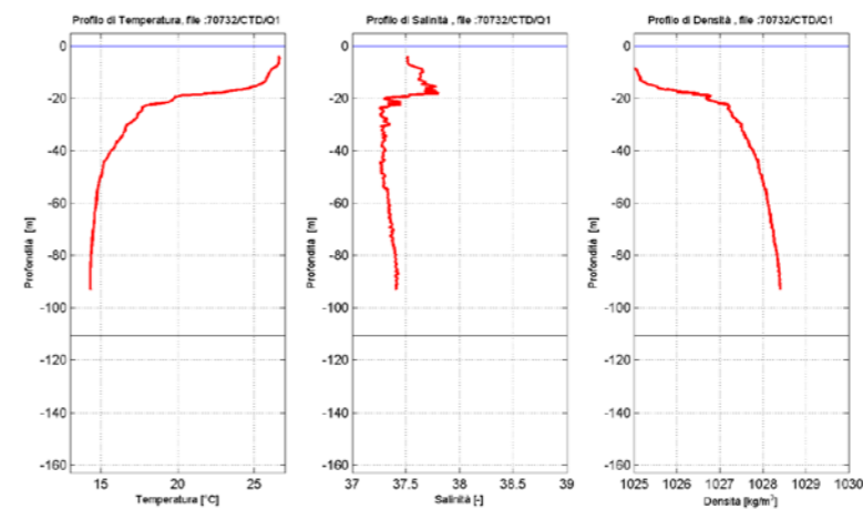
Figura 2.8: Profili di Temperatura (sinistra), Salinità (centro) e Densità (destra) misurati in D, E, F, G, O, Q in Agosto (inizio) 2017
