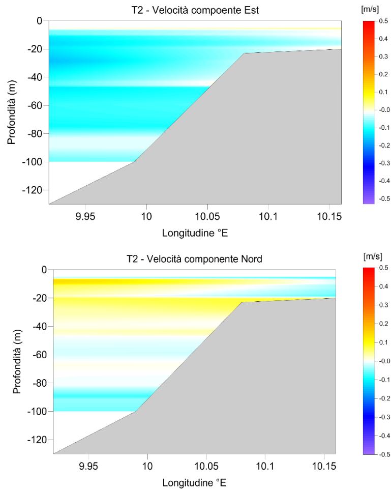
Figura 2.17: Transetto T2 – Ottobre 2017 – Valori Caratteristici delle Componenti Est (Sopra) e Nord (Sotto) della Velocità di Corrente
