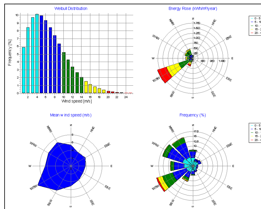
Figura 5: Caratteristiche anemologiche previste nel punto di installazione della turbina AS01 ad altezza mozzo di 110 m s.l.t.
