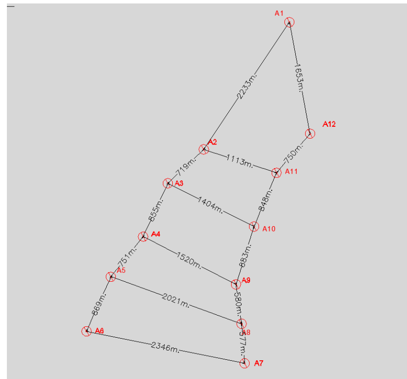
Figura 3 – Schema layout con indicazione delle interdistanze tra le turbine di progetto
