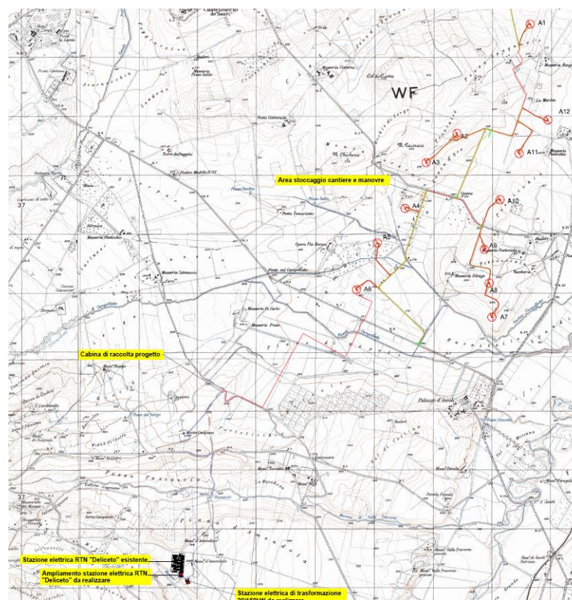
Figura 4 – layout d'impianto
