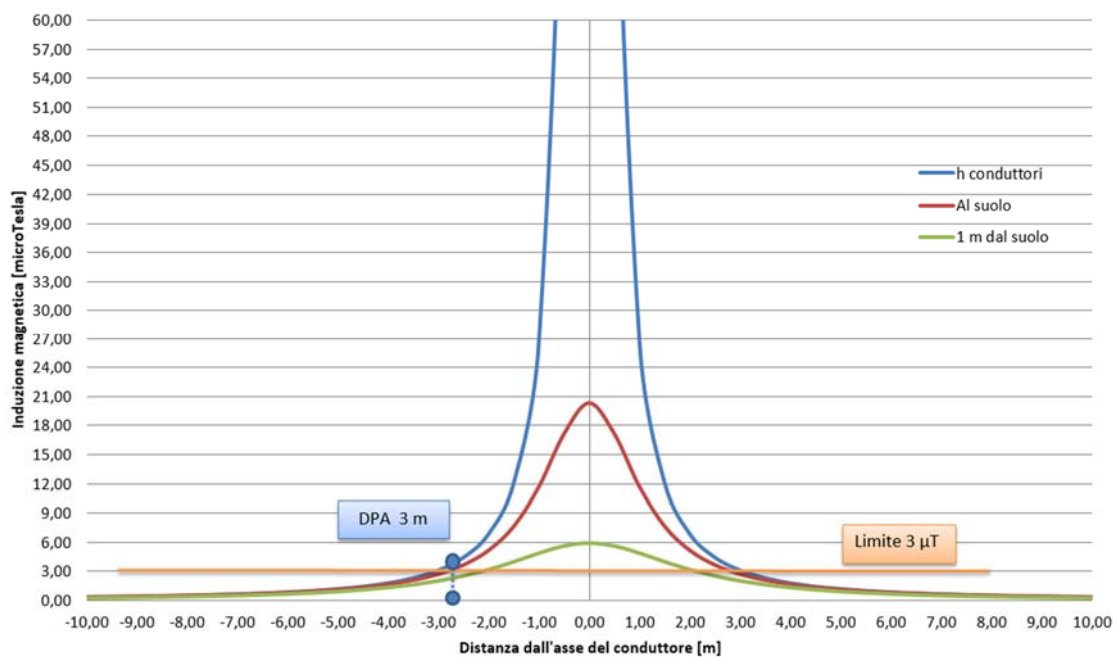
Figura 19: Andamento del campo magnetico in funzione della distanza dall'asse dei conduttori in forma grafica - Cavidotto AT.
