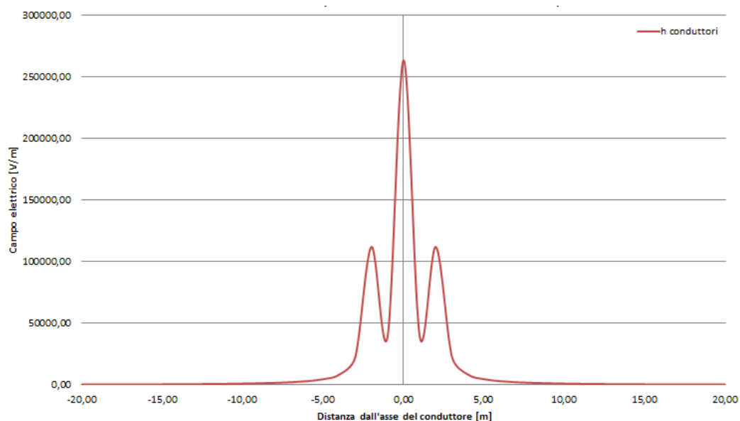
Figura 16: Andamento del campo elettrico in forma grafica - Sbarre AT stazione elettrica 30/150 kV.
