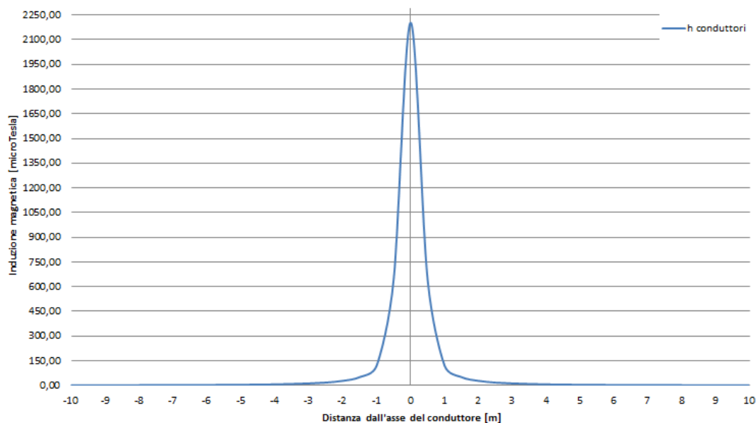
Figura 15: Andamento del campo magnetico in funzione della distanza dall'asse dei conduttori in forma grafica - Sbarre MT stazione elettrica 30/150 kV - Valutazione della Distanza di prima Approssimazione.
