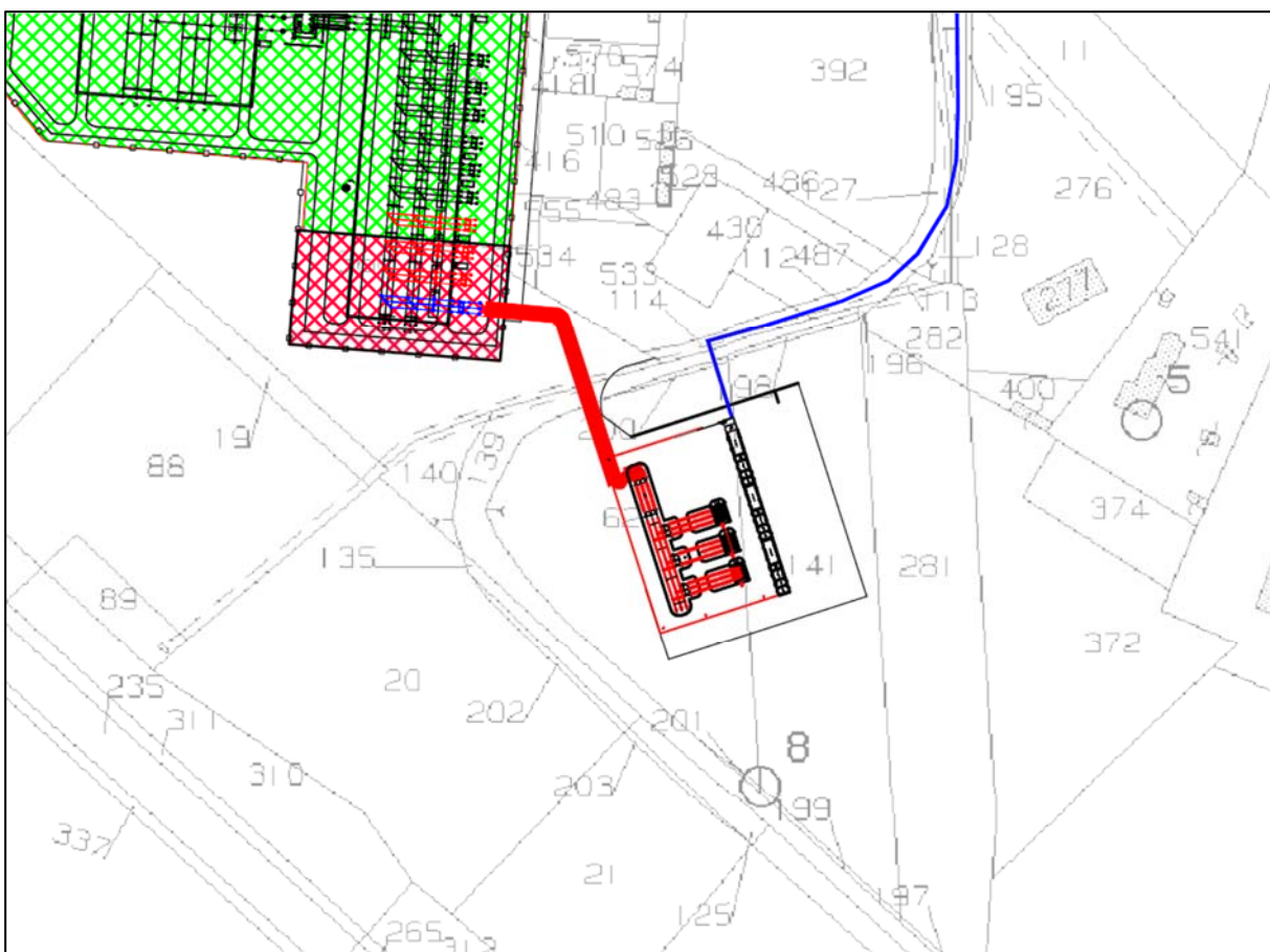
Figura 20: Rappresentazione grafica delle DPA del cavidotto AT.
