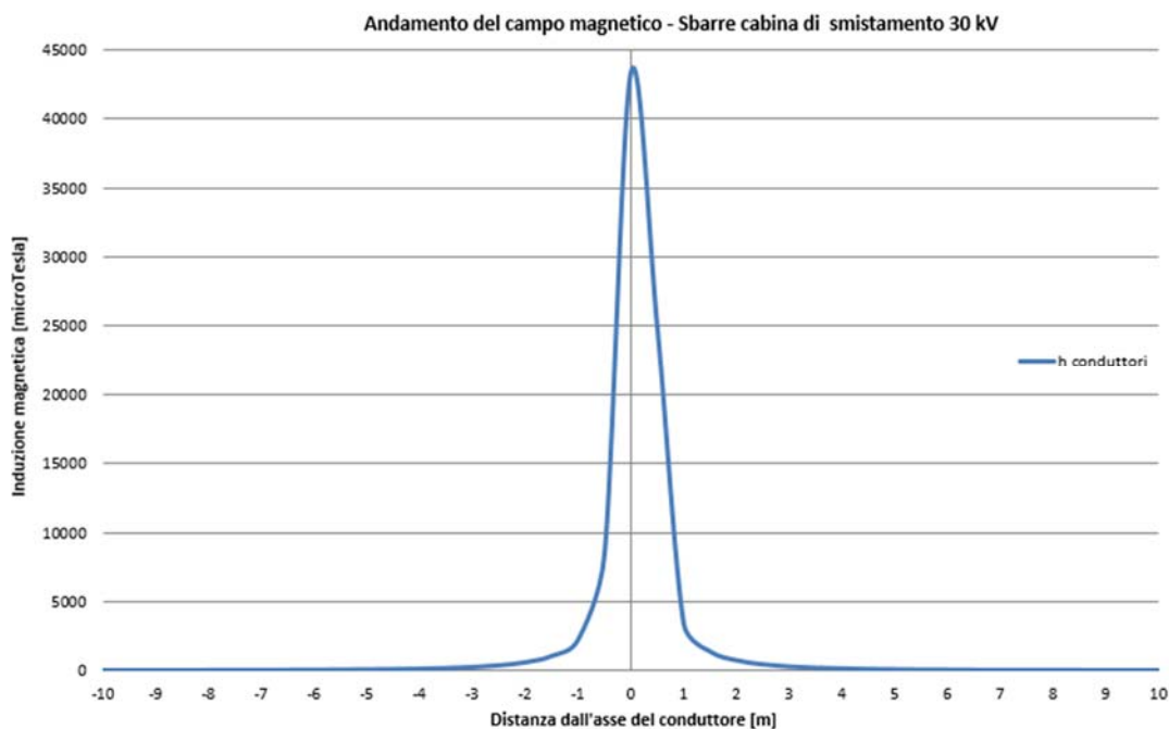
Figura 11: Andamento del campo magnetico in funzione della distanza dall'asse dei conduttori in forma grafica - Sbarre MT della cabina di raccolta.
