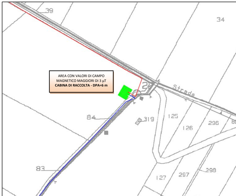
Figura 13: Rappresentazione grafica della DPA cabina di raccolta.
