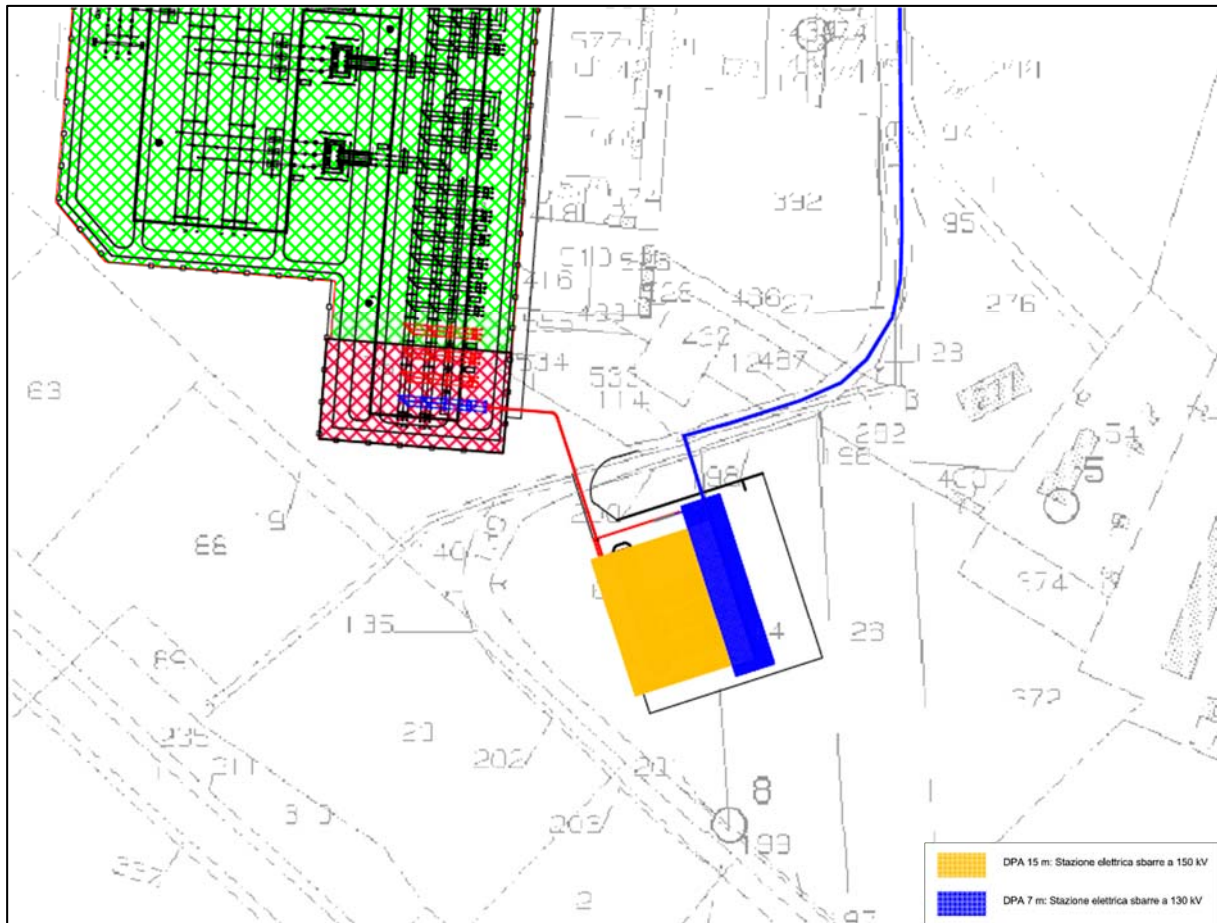
Figura 18: Rappresentazione grafica delle DPA della stazione d'utenza 30/150 kV.
