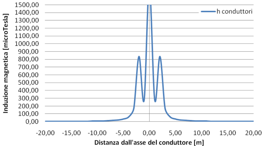
Figura 14: Andamento del campo magnetico in funzione della distanza dall'asse dei conduttori in forma grafica - Sbarre AT stazione elettrica 30/150 kV - Valutazione della Distanza di prima Approssimazione.
