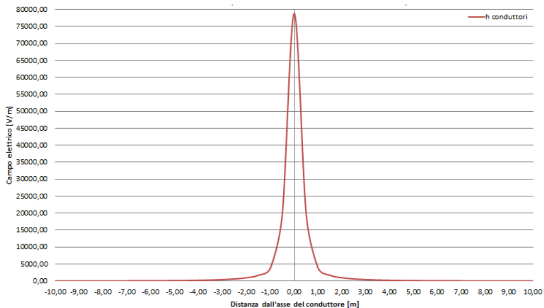
Figura 17: Andamento del campo elettrico in forma grafica - Cabina MT in stazione elettrica 30/150 kV.
