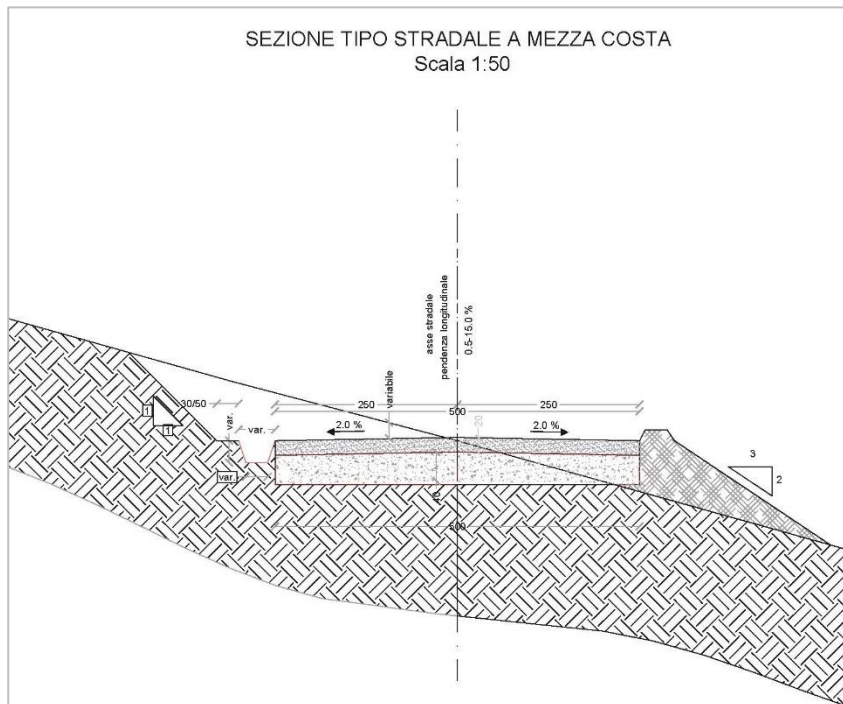
Figura 7: Sezione tipo di strada a mezzacosta
