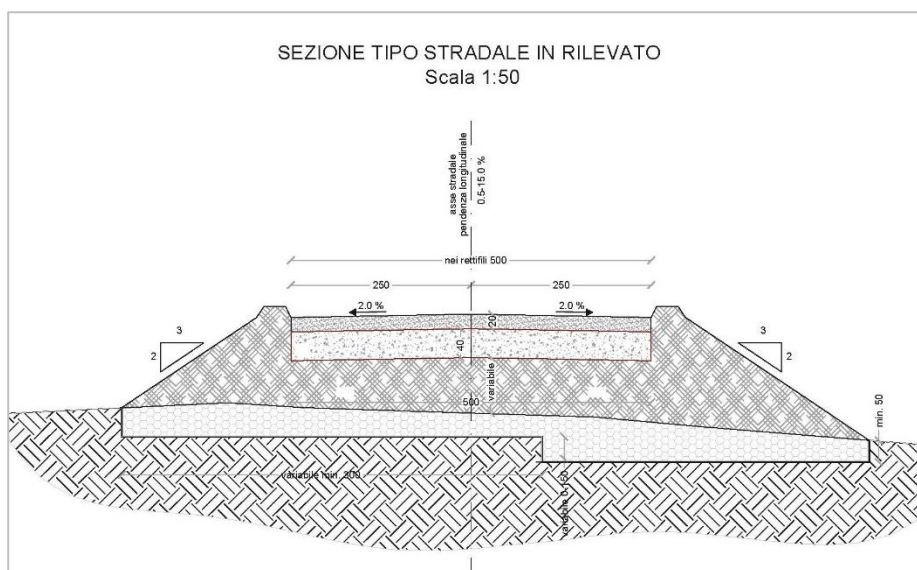
Figura 8: Sezione tipo di strada in rilevato
