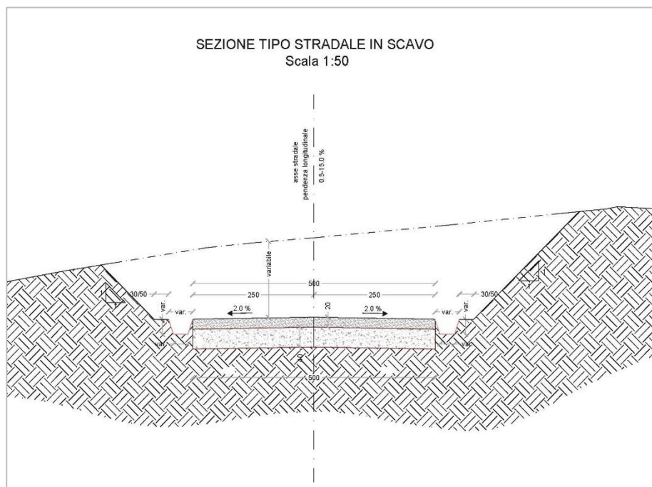
Figura 6: Sezione tipo di strada in scavo
