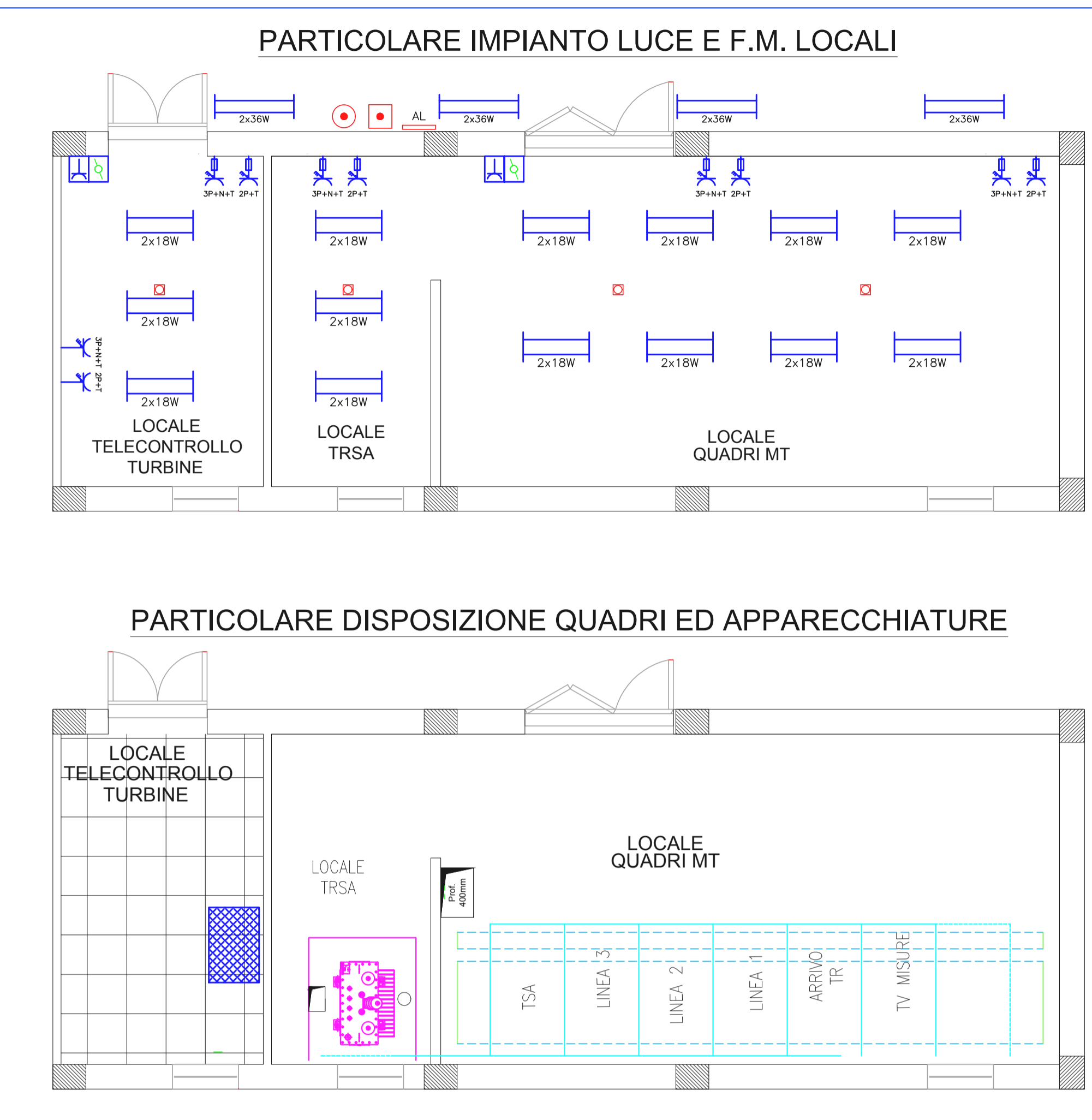
PARTICOLARE SERVIZI AUSILIARI EDIFICIO SSE DI NUOVA REALIZZAZIONE - SCALA 1:50
