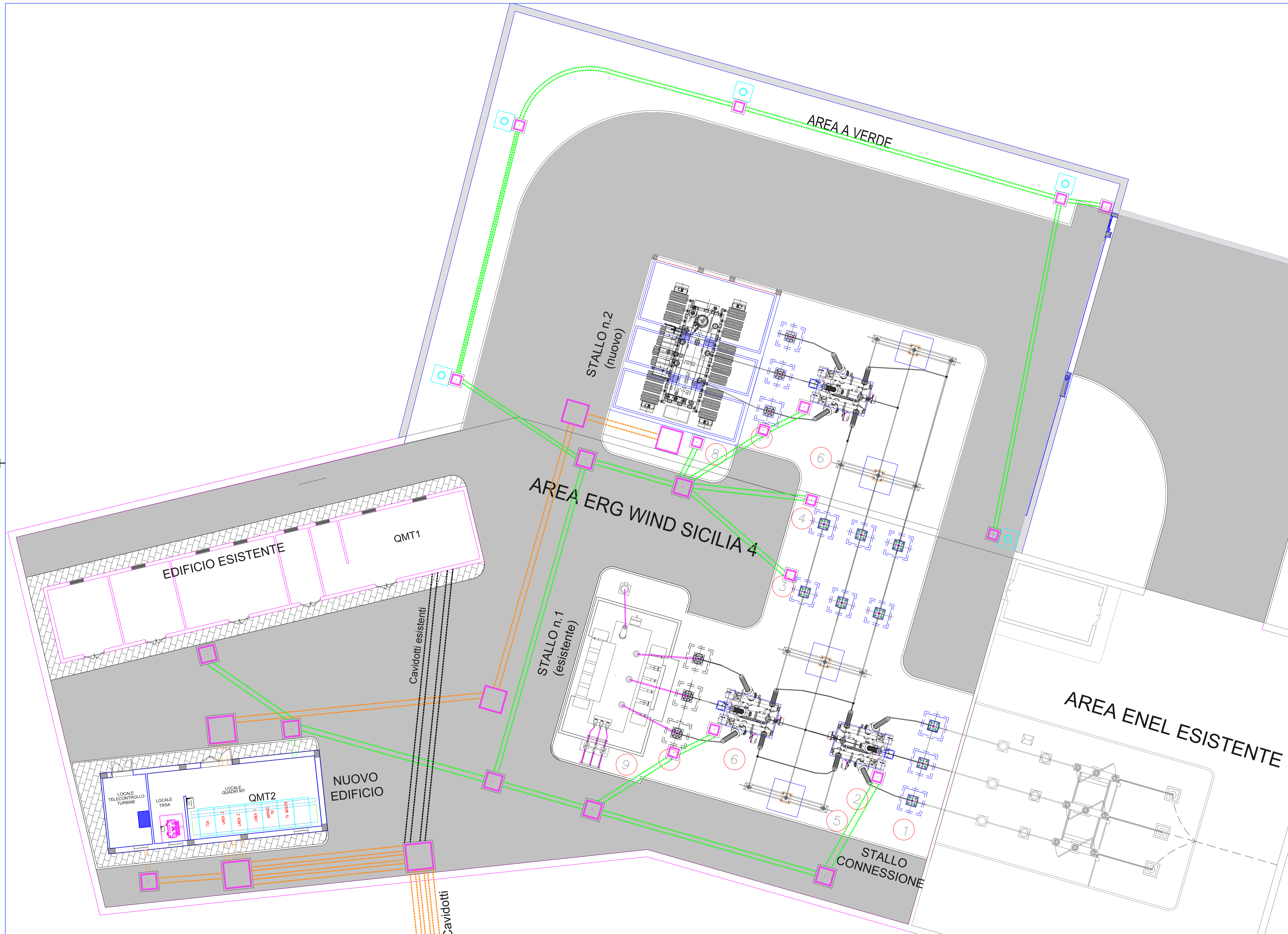
PLANIMETRIA SERVIZI AUSILIARI SSE - SCALA 1:100
