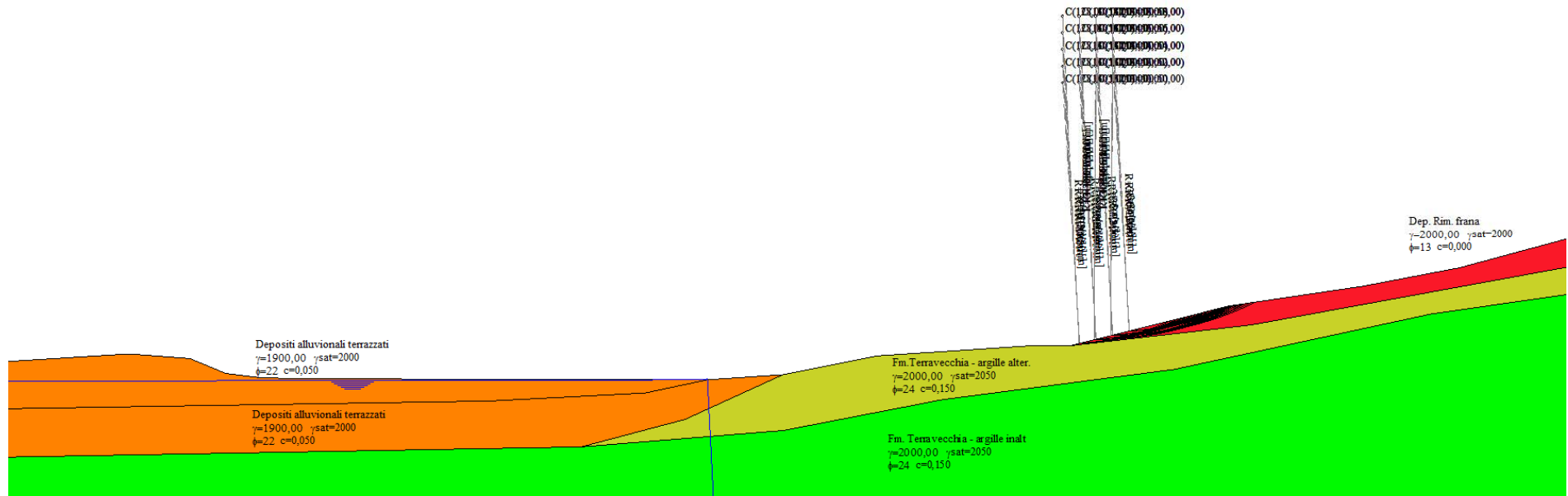
Superfici di scivolamento con F < 1,1
