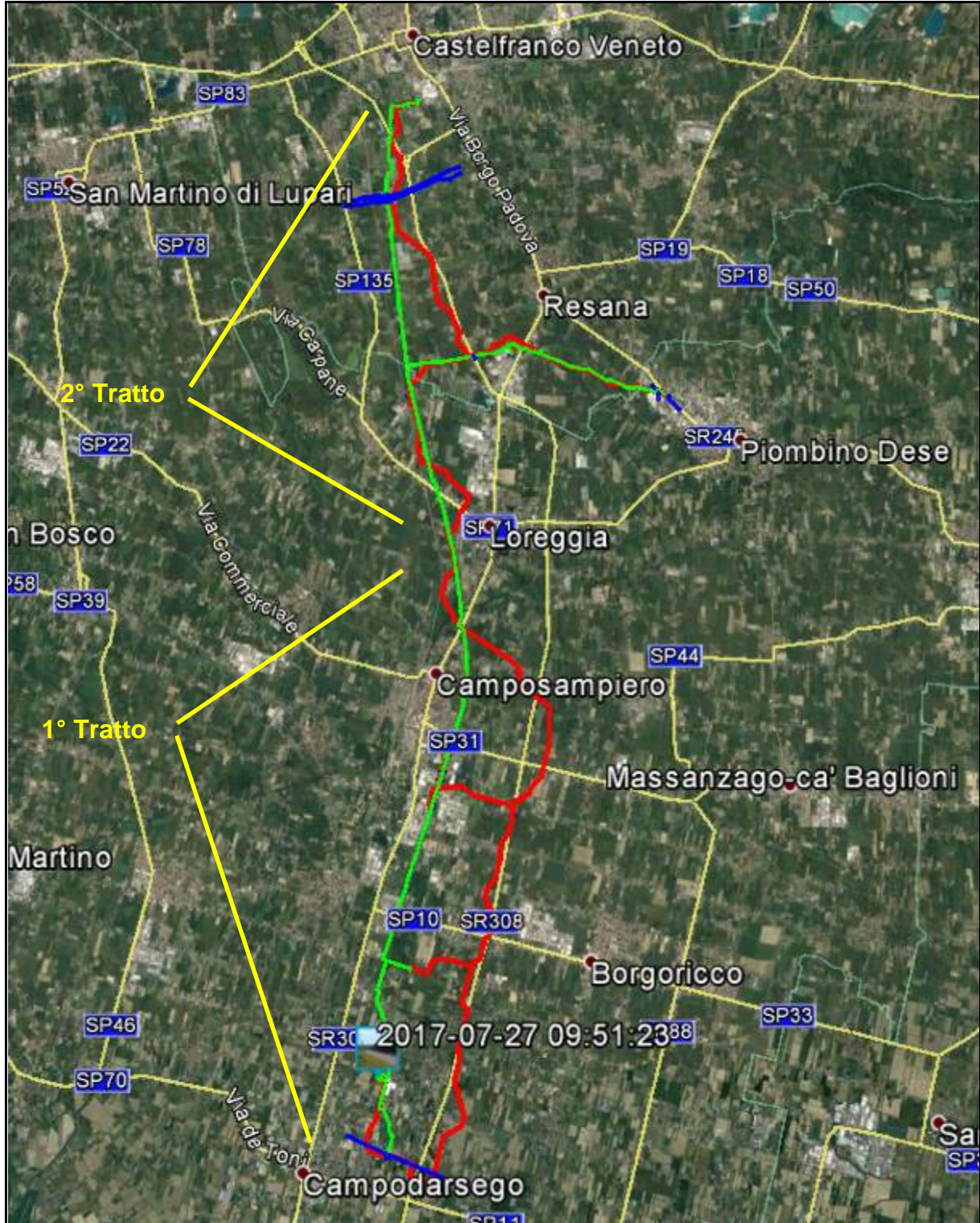
Figura 2.2/B – Immagine aerea della zona progettuale 1° Tratto (in rosso met. in progetto, in verde met. esistenti da dismettere)
